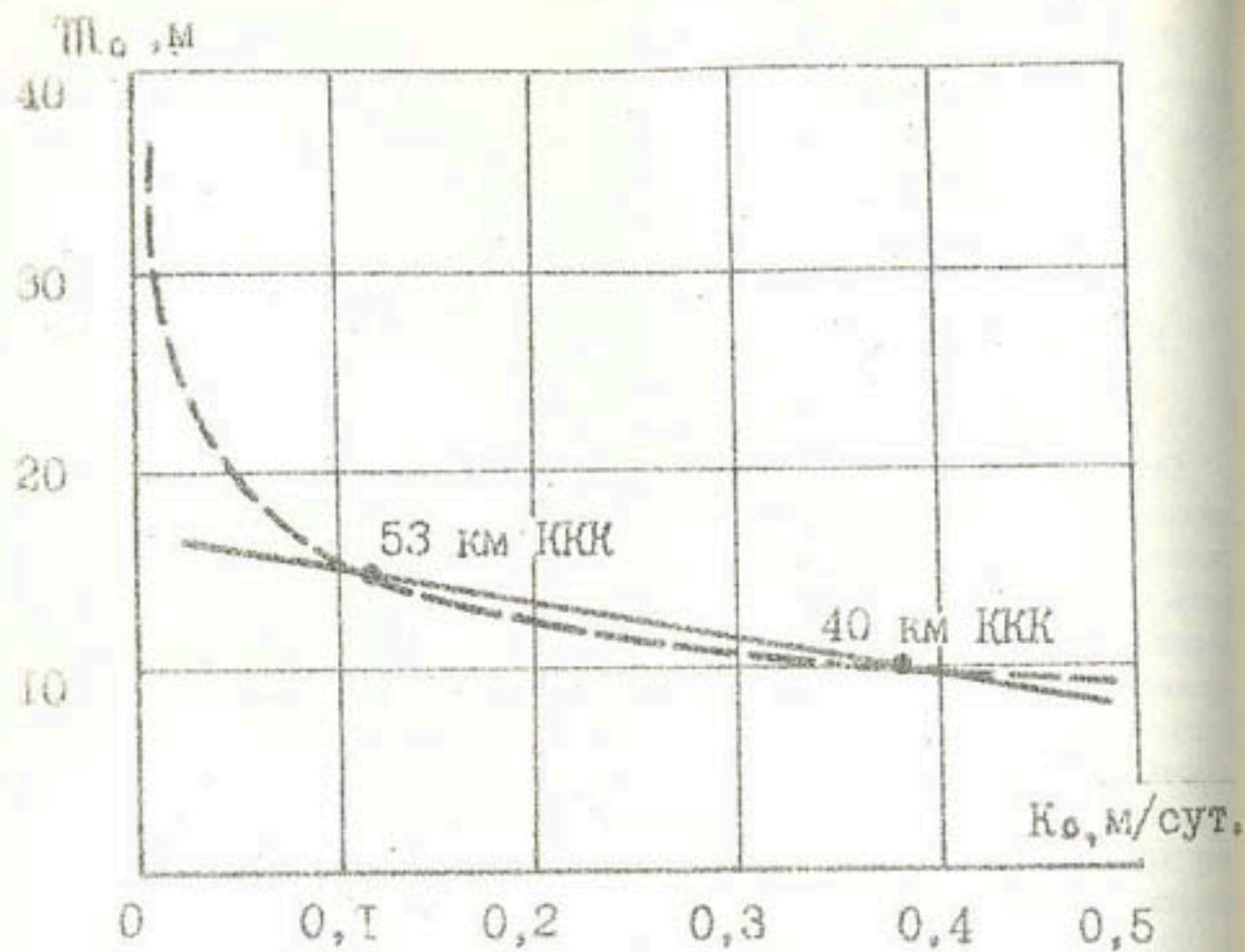
Рис. 3. Зависимость суммарной водопроницаемости песистой толщи от её мощности K_o = f(m_o) .
