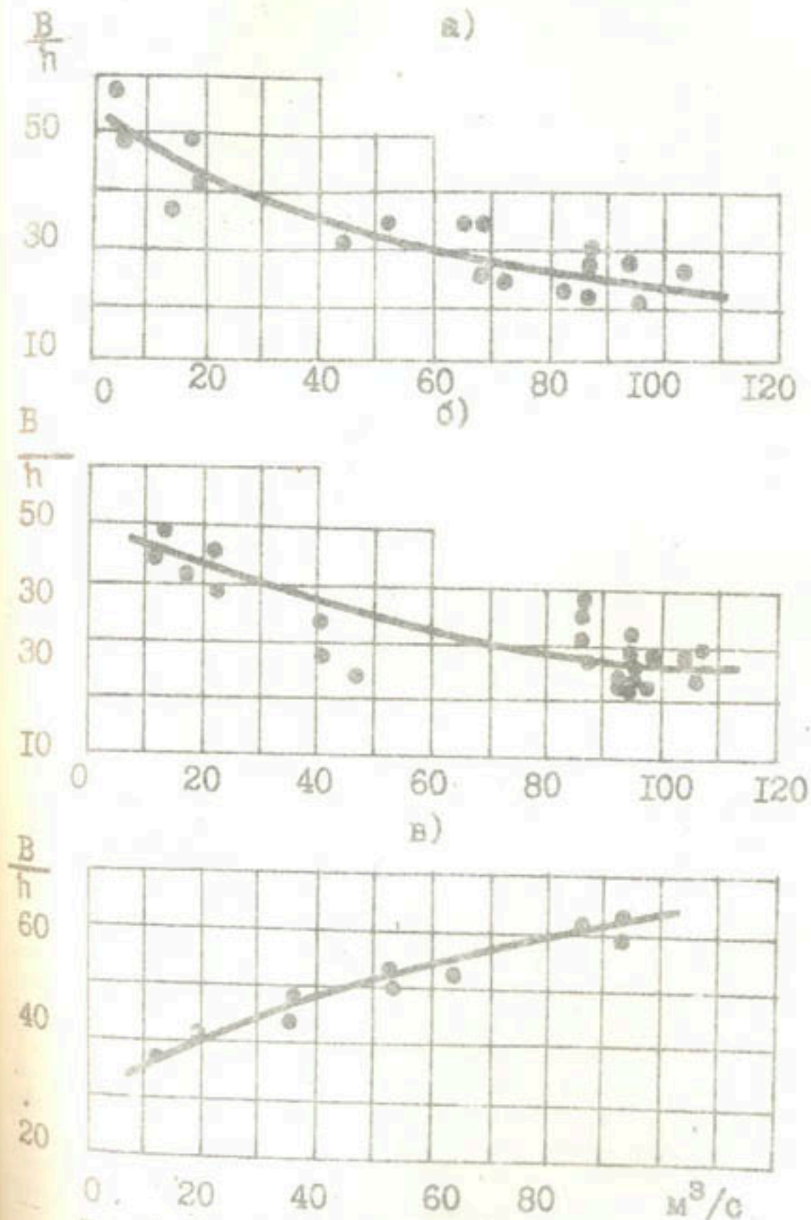
Рис. 1. Зависимость относительной ширины русла кол-лектора ( B: h_{cp.} ) от расхода воды: а - на участке су-глинистых грунтов (8, 17, 70 км); б - супесчаных грунтов (92, 122, 135 км); в - мелких песков (38-46 км).
