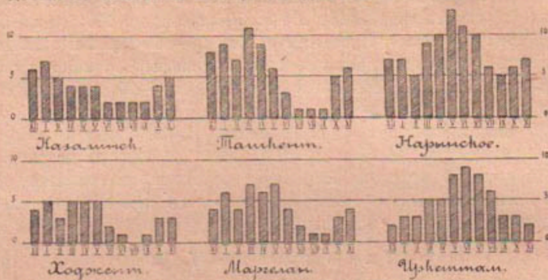
Черт. 9. Повторяемость осадков по месяцам.
