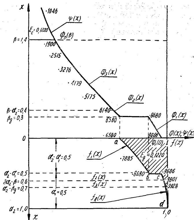
Рис. 2.3.10. Обобщенная водохозяйственная характеристика многолетнего регулирования стока для двух потребителей ( \beta=1,4 ; \beta_g=0,3 ; \alpha_2=1,0 ; \alpha_1=0,5 ; C_v \approx 0,71 )
