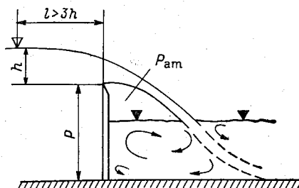
Рис. 8.6. Незаплавленный водослив с тонкой стенкой.
