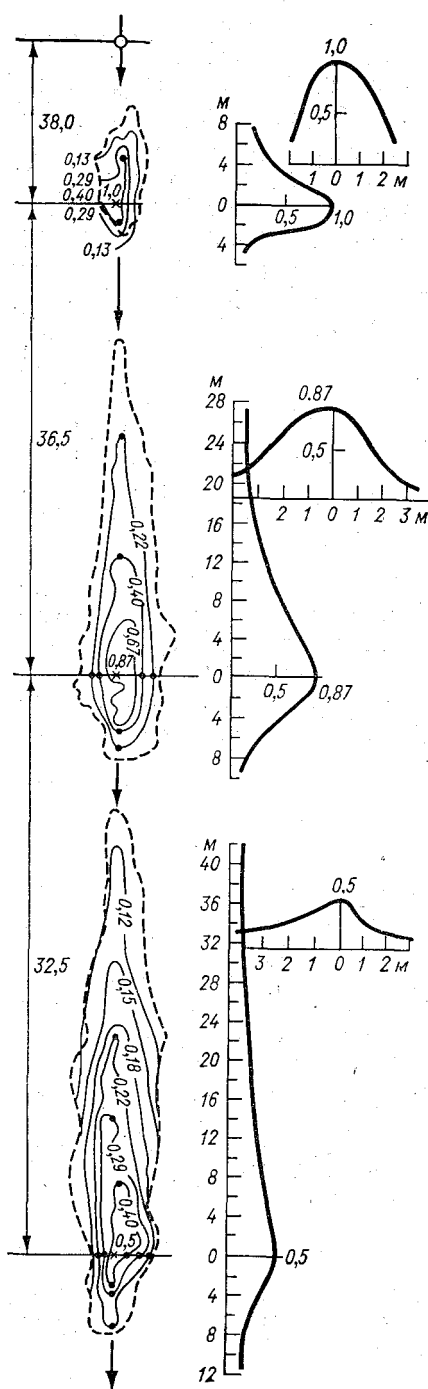
Рис. 5.13. Последовательное положение облаков раствора уранина на пойме р. Сожа. Аэрофотосъемка 1971 г. обработана В. В. Алексеевым [ГГИ].
