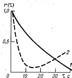
Рис. 5.4. Автокорреляционные функции средних скоростей на вертикалях. 1 — р. Сож, 2 — Большой Ставропольский канал.
