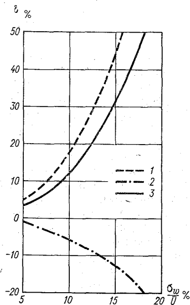
Рис. 4.12. Систематические погрешности измерения осредненной скорости турбулентного потока вертушкой ГР-55.
