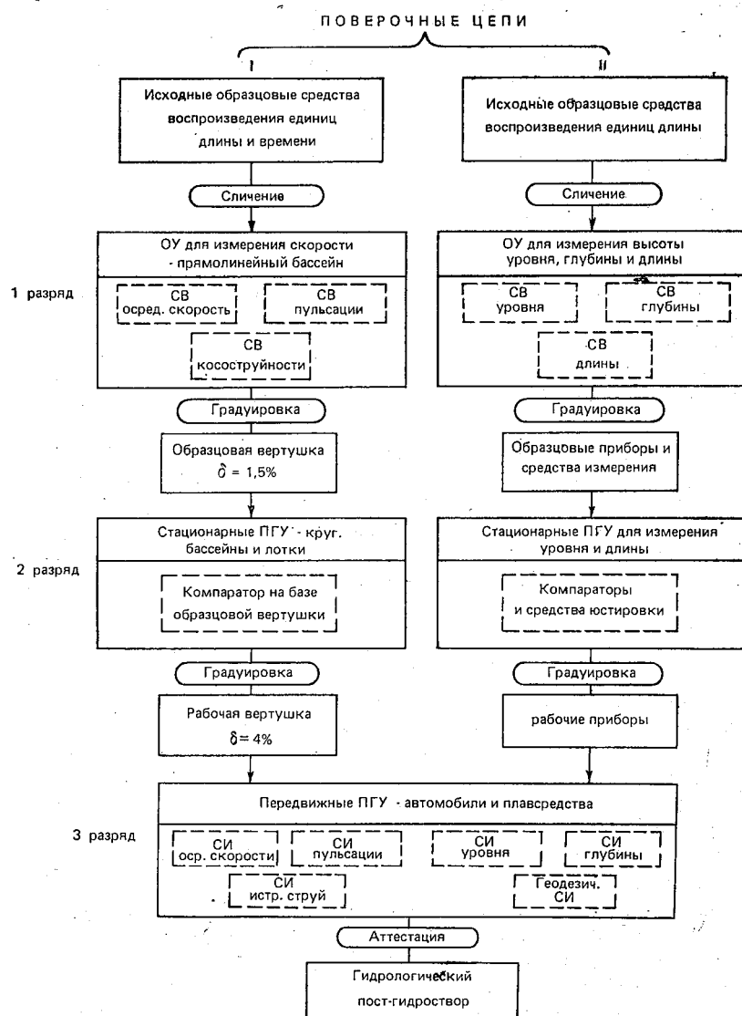
Рис. 9.5. Вариант поверочно-градуировочной системы и организации метрологического обеспечения гидрологических наблюдений.
