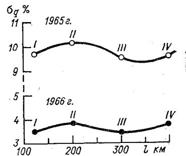
Рис. 7.1. Изменение тесноты связи расходов и уровней в сопряженных створах в зависимости от расстояний между ними в зоне подпора Куйбышевского водохранилища ниже г. Чебоксары.
