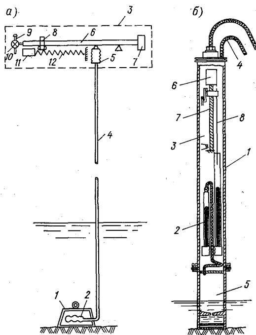
Рис. 2.8. Гидростатические уровнемеры.
