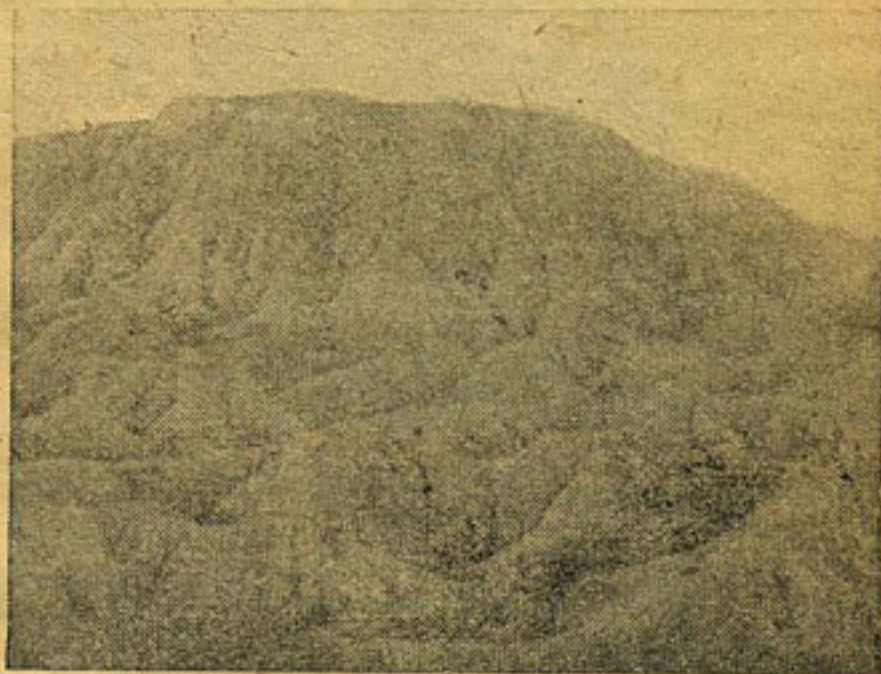
Рис. 4. Формы карстового размыва на Мадом Балахане—слепые овраги, оканчивающиеся поглощающими шахтами (по Нацкому)
