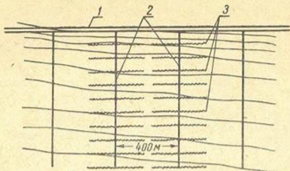
Рис. 3. Схема оросительной сети с закрытыми оросителями (полевыми трубопроводами): 1 — хозяйственный канал; 2 — закрытые оросители (полевые трубопроводы); 3 — гибкие поливные трубопроводы или борозды.
