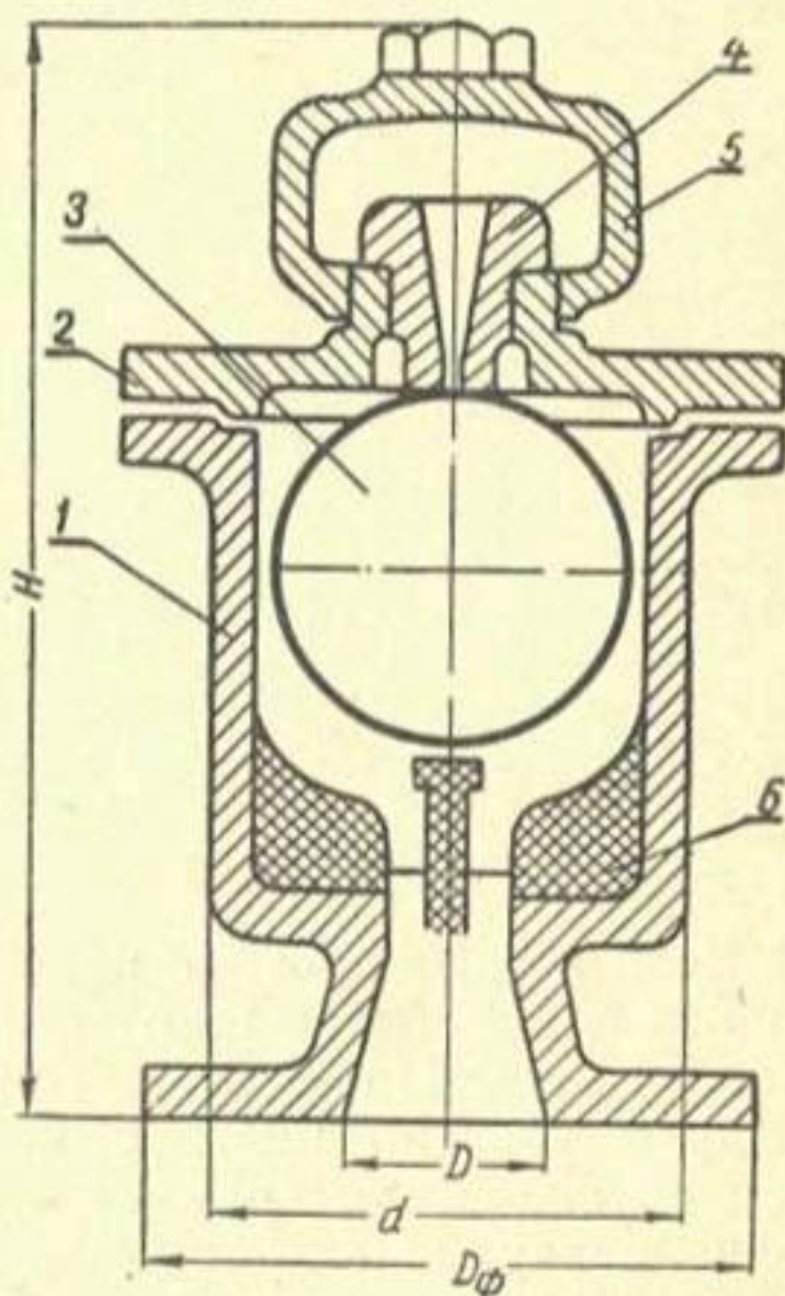
Рис. 57. Эксплуатационный вантуз:
