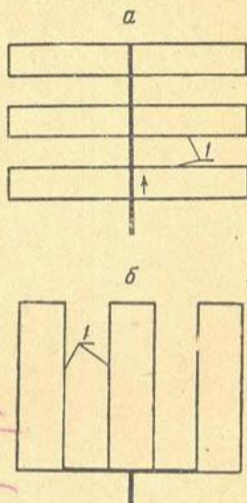
Рис. 4. Основные схемы закрытой оросительной сети с механической подачей воды: а — Т-образная; б — Ш-образная; 1 — полевые трубопроводы.
