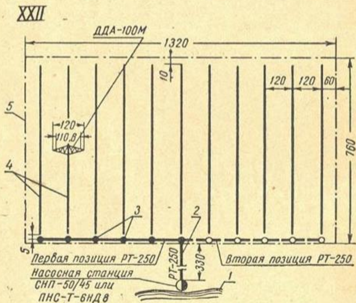
Рис. 10. Схемы орошения участков с помощью дождевального агрегата ДДА-100М: XXI—XXII — площадь орошения за сезон 100 га; 1 — водоем; 2 — подводящая часть трубопровода; 3 — труба-гидрант 250×180; 4 — открытые оросители; 5 — граница орошаемой площади.
