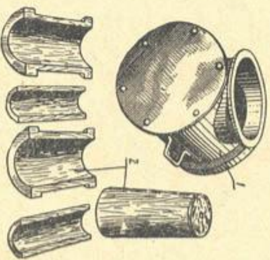
Рис. 55. Разборная опалубка: 1 — металлическая разъемная форма; 2 — резиновый сердечник.
