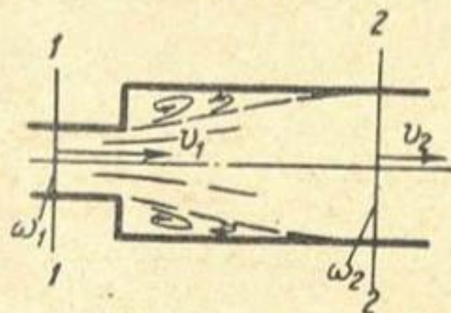
Рис. 35. Внезапное расширение.
