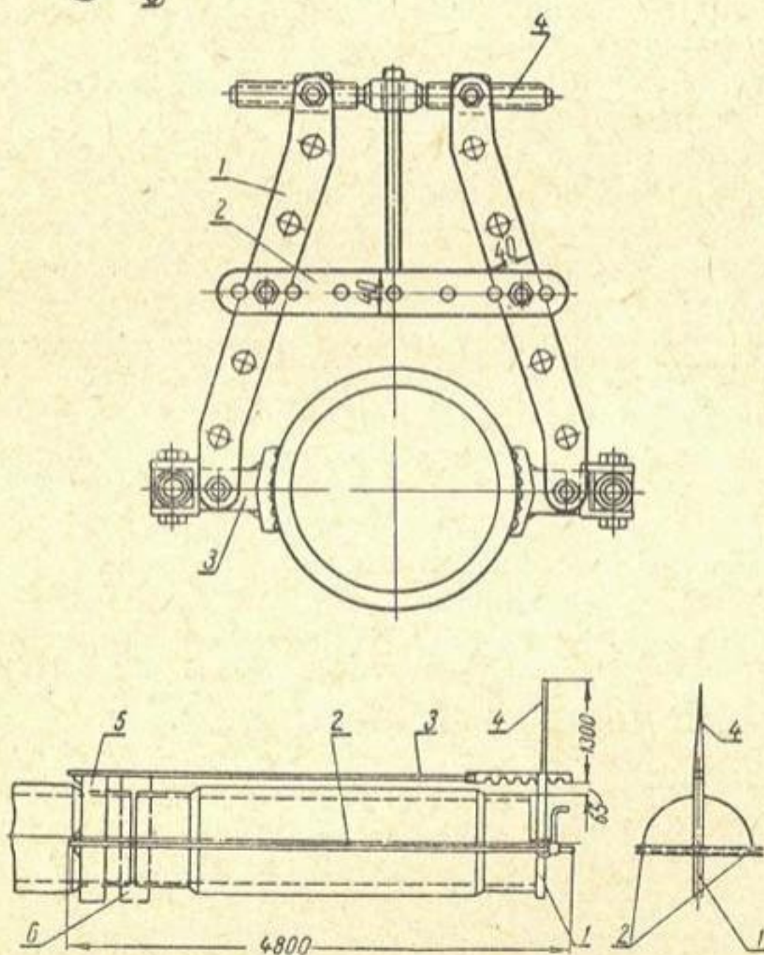
Рис. 77. Соединение труб больших диаметров винтовым домкратом:
