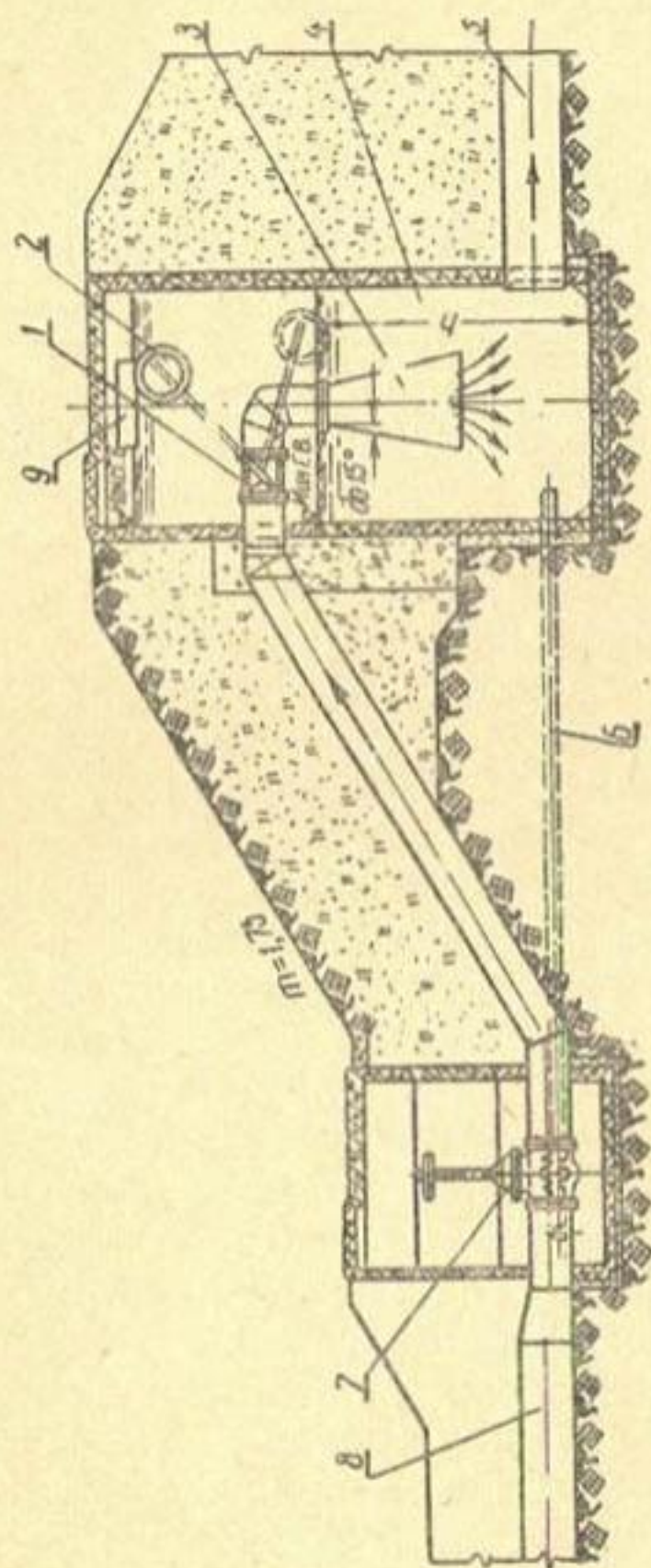
Рис. 66. Гаситель напора с дрессельным затвором: 1 — дрессельный затвор; 2 — поплавок; 3 — конусный выходной патрубок; 4 — колодец; 5 — нижерасположенный трубопровод; 6 — водовыпускная труба; 7 — задвижка; 8 — выше- расположенный трубопровод; 9 — водосливное отверстие.
