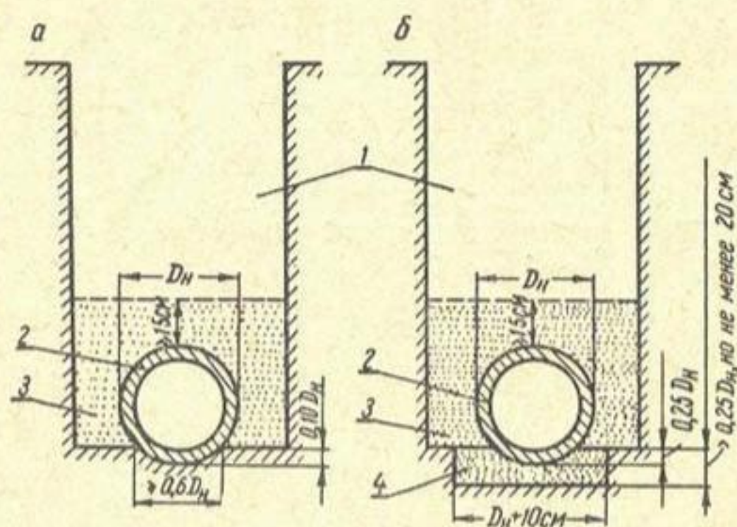
Рис. 72. Способы укладки напорных трубопроводов. а — на естественном основании; б — на песчаном основании; 1 — траншея; 2 — труба; 3 — утрамбованная засыпка; 4 — песчаное основание.
