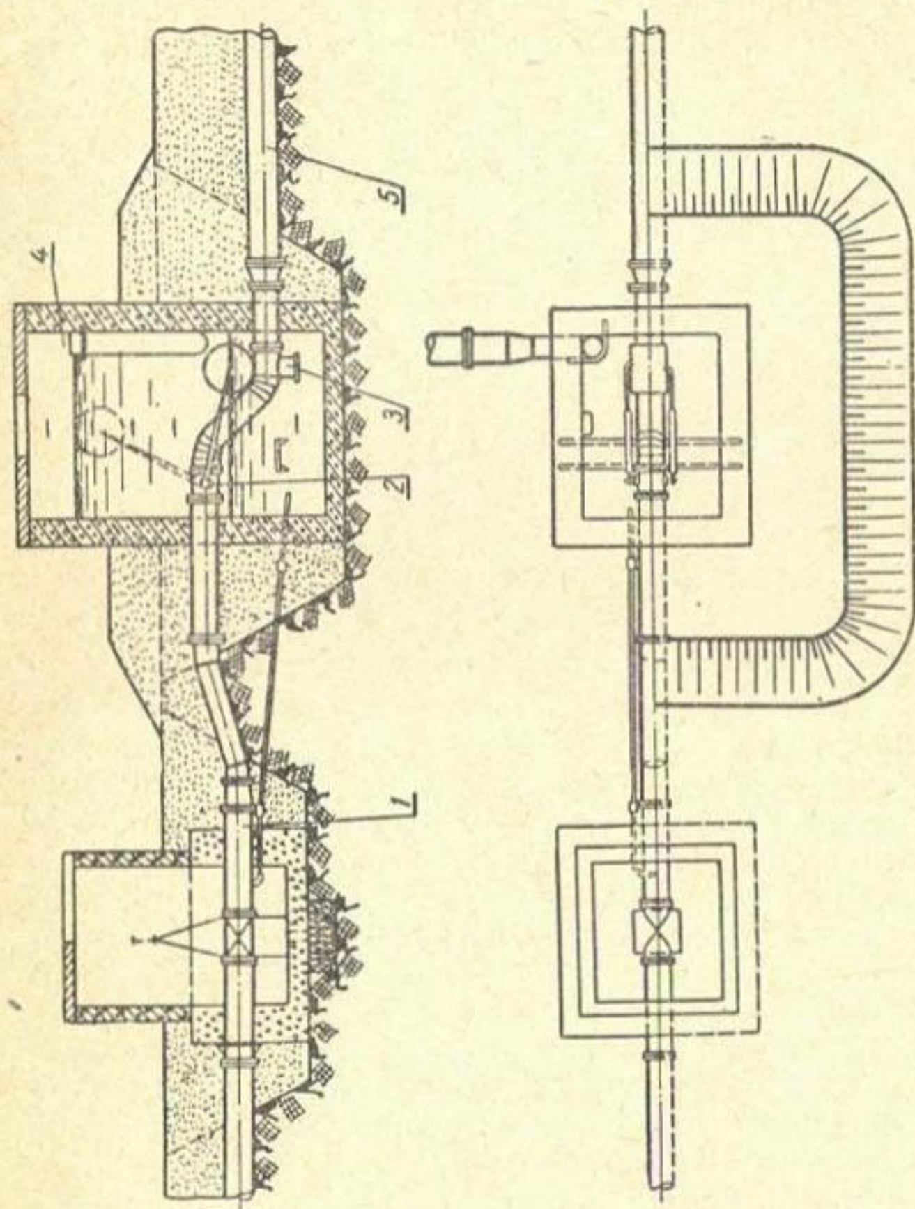
Рис. 67. Гаситель напора с патрубок-отводом: 1 — вышерасположенный трубопровод; 2 — дроссельный клапан; 3 — патрубок-отвод; 4 — ко- лдец; 5 — нижерасположенный трубопровод.
