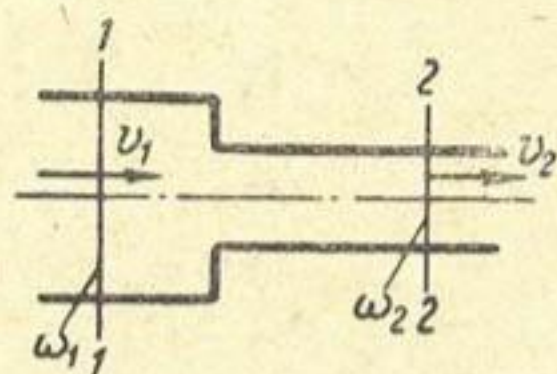
Рис. 36. Внезапное сужение.
