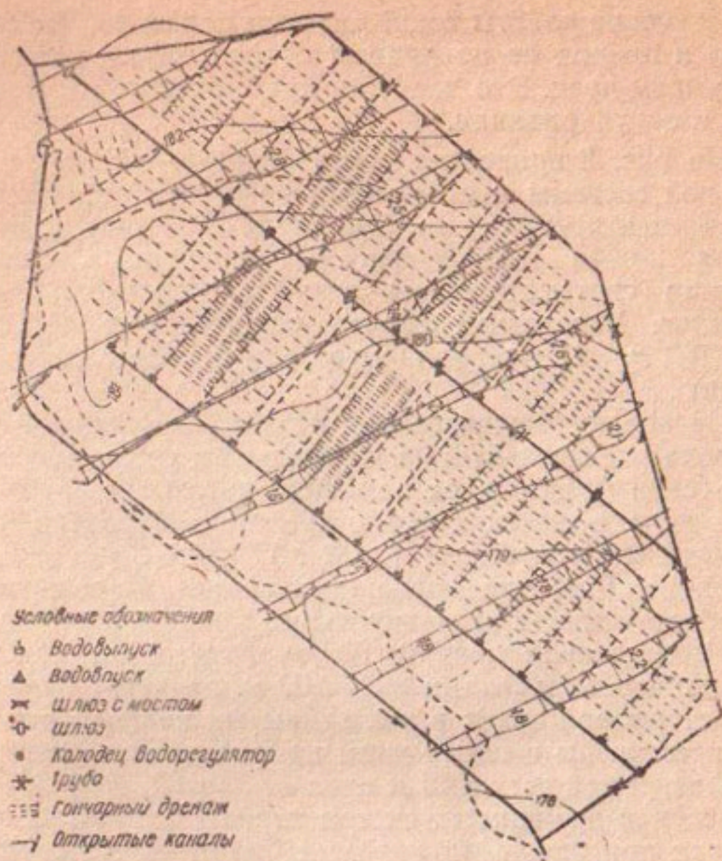
Рис. 1. Схема осушения гончарным дренажем двухстороннего действия торфяно-болотных почв.
