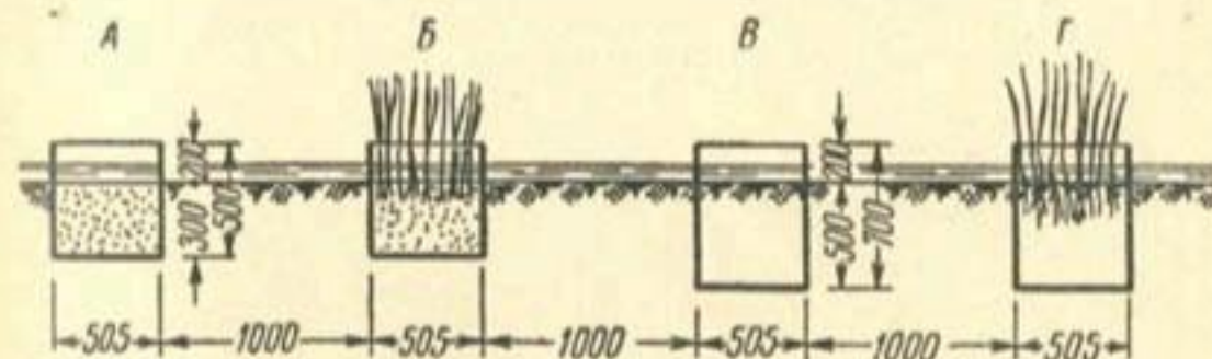
Рис. 31. Схема полевых вегетационных сосудов-испарителей.
