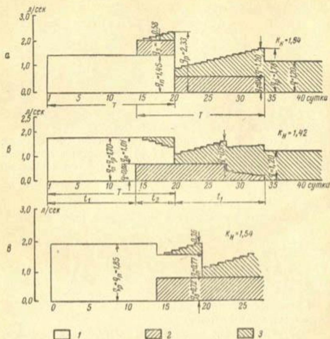
Рис. 37. График гидромодуля для периода первоначального затопления. Тип второй:
