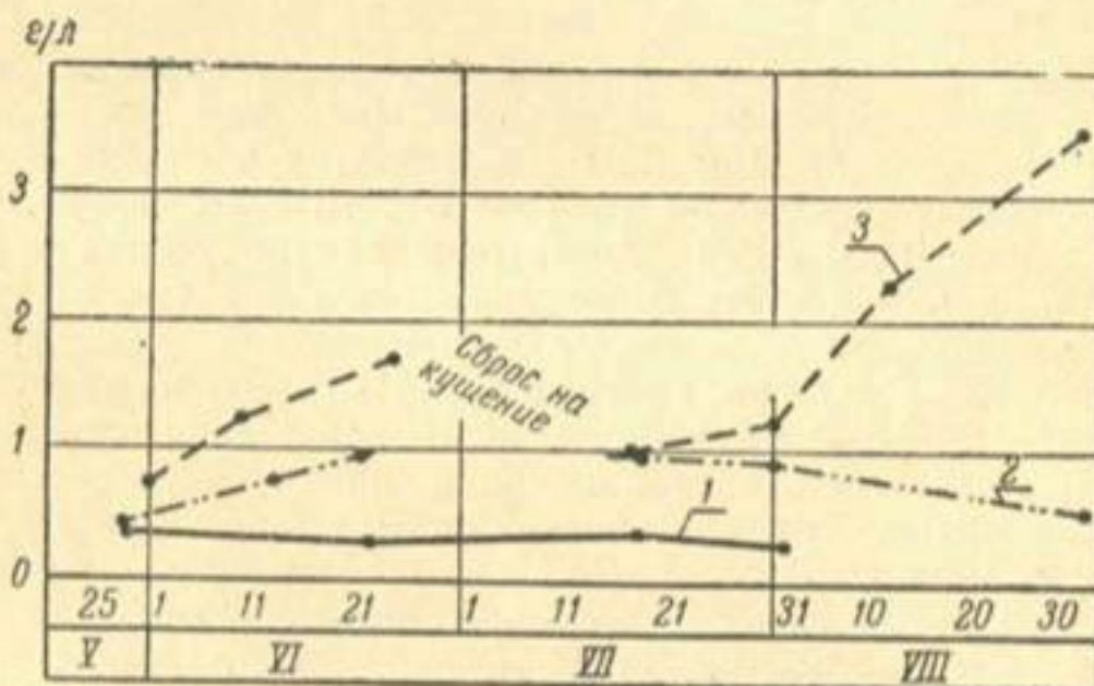
Рис. 13. Содержание солей (в г/л) в поливной воде и на чеках (дельта р. Терек): 1 — вода в оросителе; 2 — вода в проточном чеке; 3 — вода в непроточном чеке.
