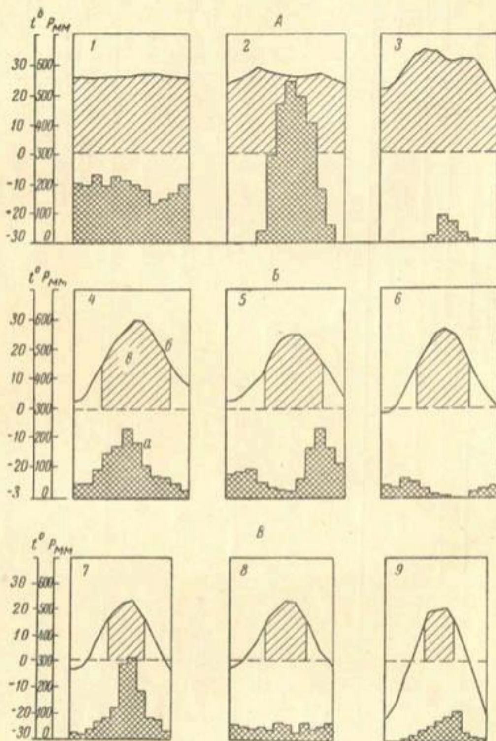
Рис. 1. Климатические диаграммы по районам рисосеяния: А — тропический пояс: 1 — Баликпалан (Индонезия), 1°17' ю.ш. Высота над уровнем моря (в м) H=5 ; 2 — Рангун (Бирма), 16°47' с.ш., H=13 ; 3 — Тимбукту (Мали), 16°43' с.ш., H=250 ; Б — субтропический пояс: 4 — Ханькоу (Китай), 30°35' с.ш., H=36 ; 5 — Ленкорань (СССР), 38°46' с.ш., H=19 ; 6 — Ташкент (СССР), 41°20' с.ш., H=479 ; В — умеренный пояс: 7 — Вонсан (Корея), 39°09' с.ш., H=0 ; 8 — Краснодар (СССР), 45°02' с.ш., H=34 ; 9 — Уссурийск (СССР), 43°47' с.ш., H=25 ; а — осадки; б — среднесуточные температуры; в — период возможной вегетации риса.
