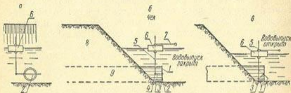
Рис. 64. Схема поплавкового водовыпуска-автомата системы Разоренова:
