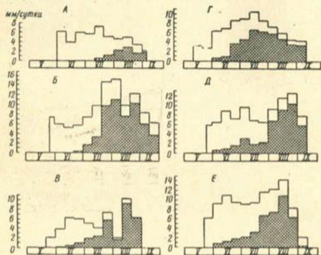
Рис. 38. Графики водопотребления:
