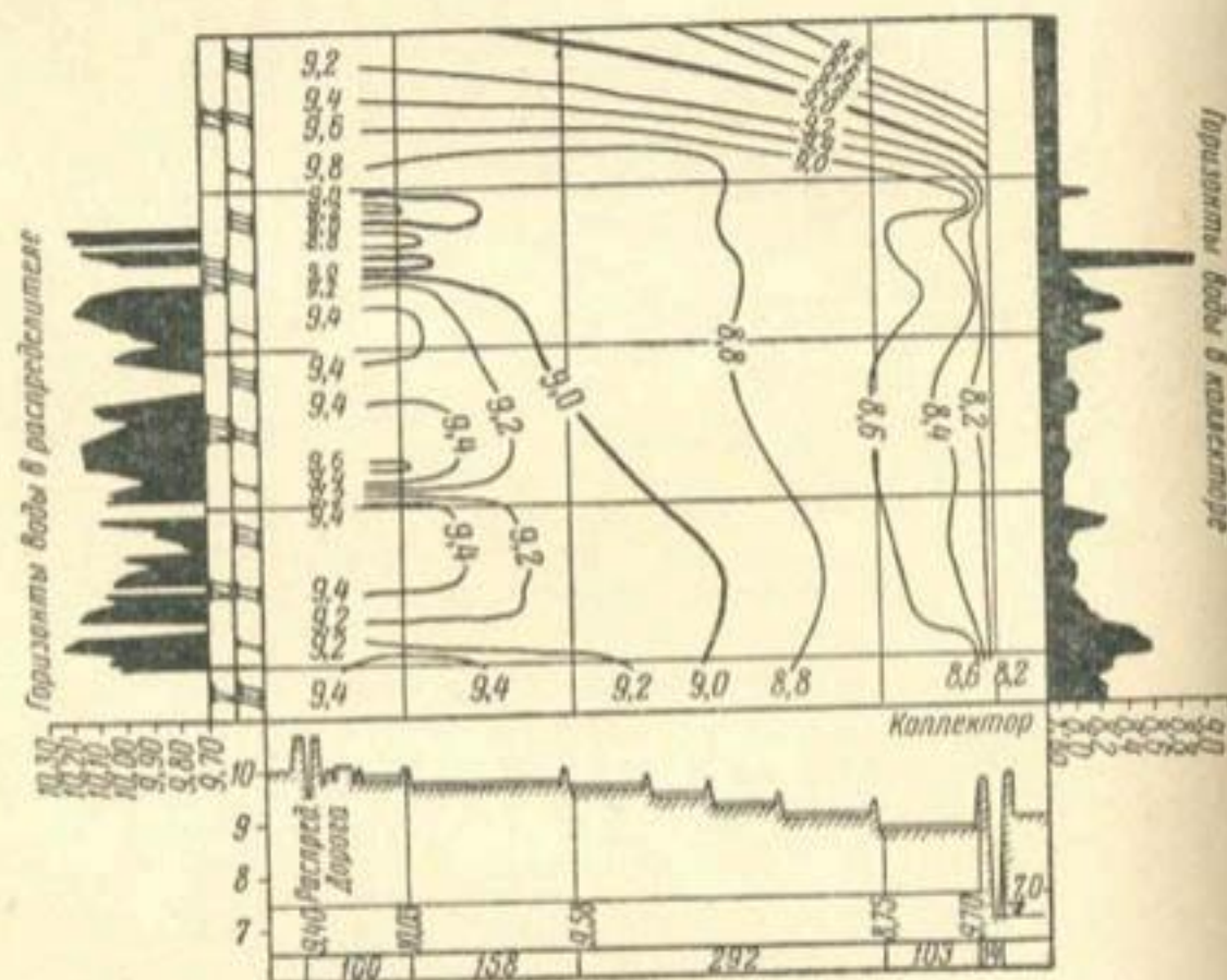
Рис. 23. Гидроизоплеты грунтовых вод. Створ вдоль карты (КубРОС, 1960 г.).
