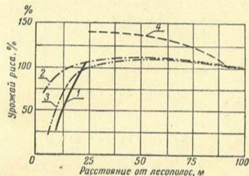
Рис. 68. Влияние лесополос на урожай риса: 1—Кубанская система (А. П. Джулай); 2—Красноармейский рисосовхоз (М. С. Родионов); 3—колхоз им. Ленина (М. С. Родионов); 4—Приморский край (Г. И. Подойницын).
