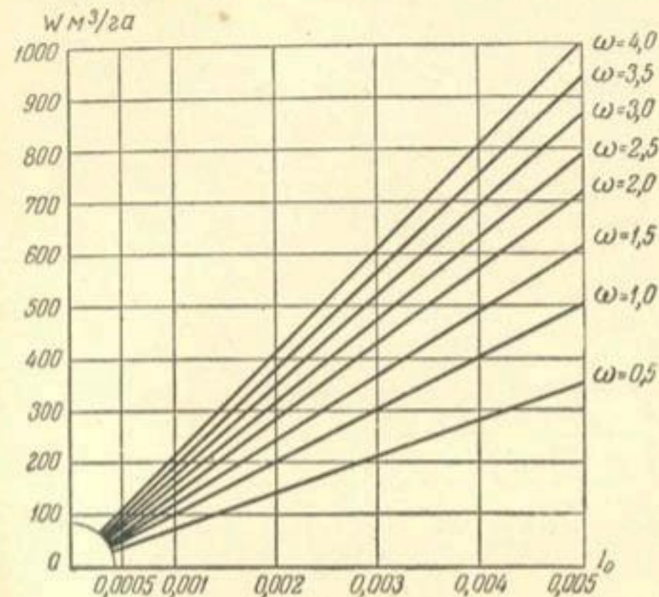
Рис. 49. График функции 10^5 I_o \sqrt{\omega} .
