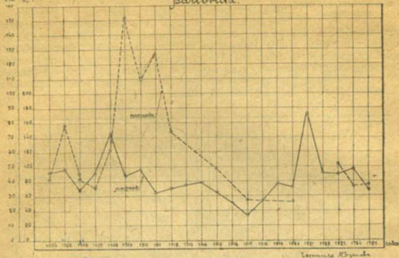
Кривые №1 зависимости числа действующих систем Нижне-Сыр-Дарьинского и Отрарского рай- онов от расхода в рене Сыр-Дарьи по планам.
