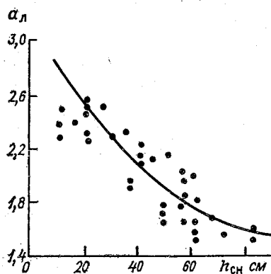
Рис. 4.1. Связь коэффициента a_{\text{л}} с толщиной слоя снега h_{\text{сн}} .
