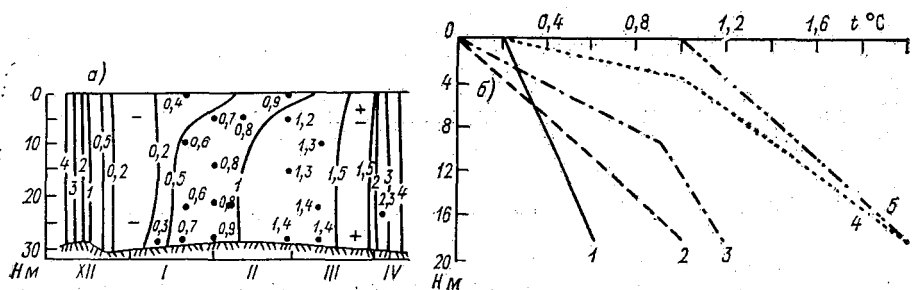
Рис. 7.6. Температура воды под ледяным покровом на Каховском (а) и Рыбинском (б) водохранилищах.
