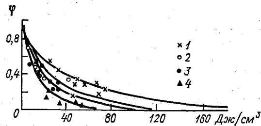
Рис. 5.1. Зависимость относительного разрушающего напряжения на изгиб образцов тающего льда от количества поглощенного им тепла солнечной радиации [35].
