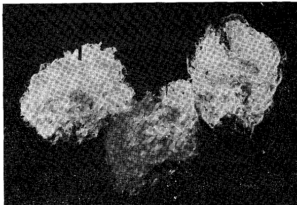
Рис. 2.3. Комья шуги.
