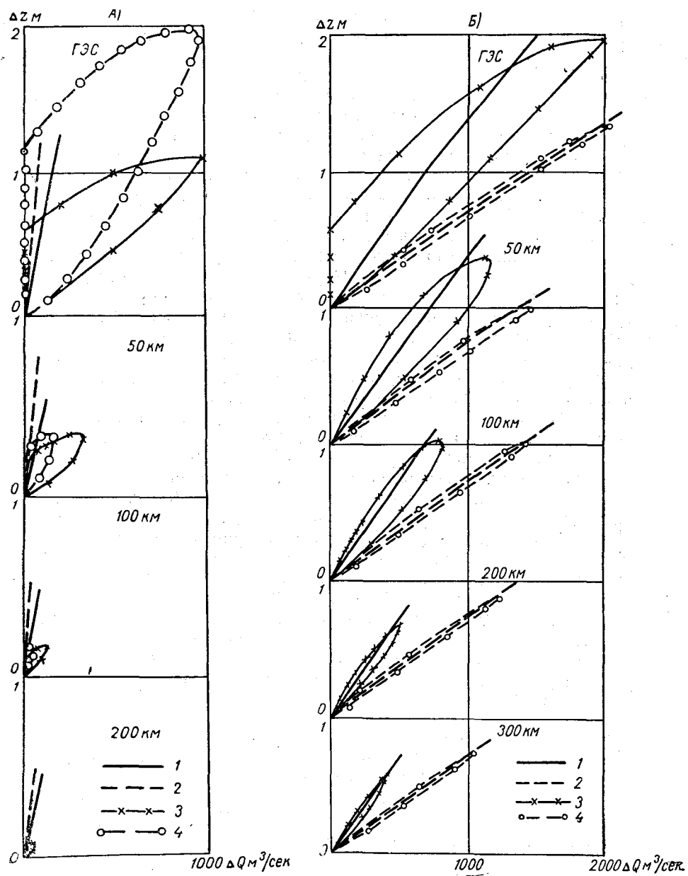
Рис. 10.17. А — влияние n на петли попусков при i_0=0,00001 . 1 и 2 — однозначные связи \Delta Q (\Delta z) , 3 и 4 — петли соответственно при n=0,02 и n=0,05 . Б — влияние i_0 на петли попусков при n=0,02 (1 и 2 — однозначные связи, 3 и 4 — петли соответственно при i_0=0,0001 и i_0=0,0004 ).
