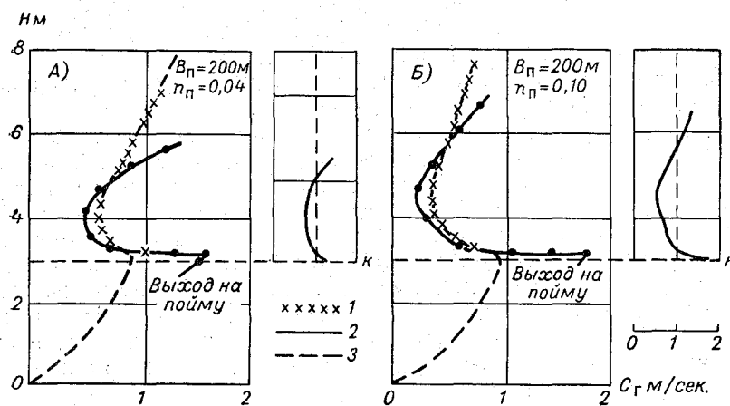
Рис. 10.24. Зависимости c_r и k от H при различной шероховатости поймы.
