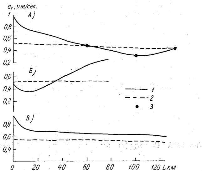
Рис. 10.28. Зависимости c_r и v от L . 1 — c_r , 2 — v_r , 3 — характерные створы.
