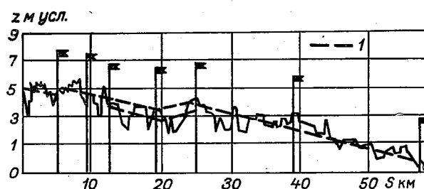
Рис. 7.2. Продольный профиль нижнего бьефа Ивановской ГЭС. 1 — линия фиктивного дна.
