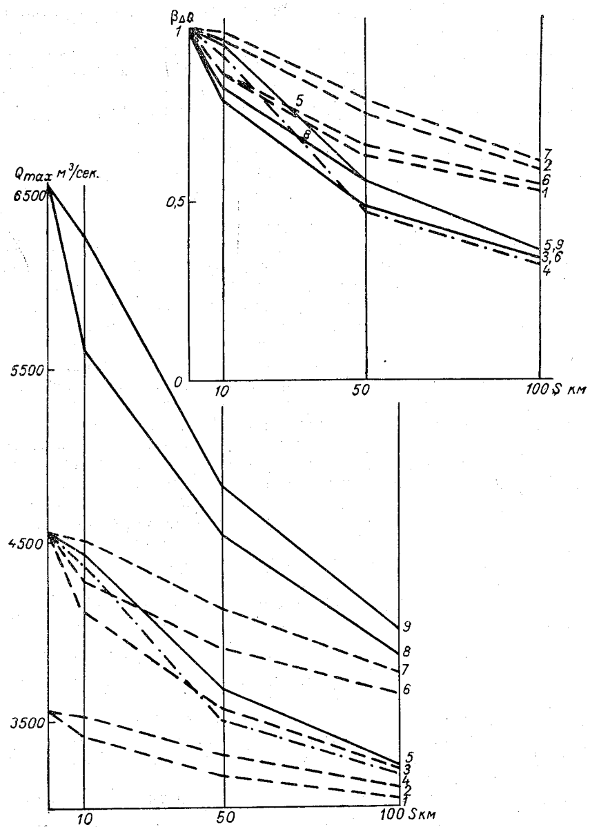
Рис. 10.18. Снижение Q_{max} и относительного приращения расходов над начальным по длине русла. Цифры у линий — номера попусков по рис. 10.14.
