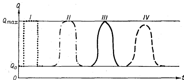
Рис. 12.1 Схема трансформации прямоугольного гидрографа.
