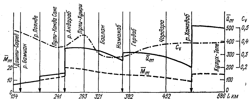
Рис. 6.5. Изменение характеристик максимальных расходов по течению р. Кундуз.
