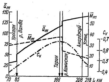
Рис. 6.15. Изменение характеристик максимальных расходов по течению р. Тарин.
