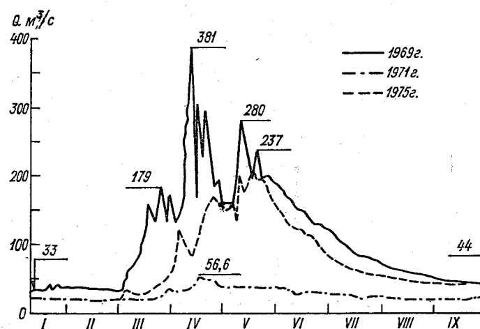
Рис. 5.12. Гидрографы расходов р. Мургаб — Каланиазхан.
