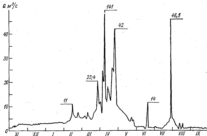
Рис. 5.5. Гидрограф р. Шомаль — Торатига за 1975-76 гидрологический год.
