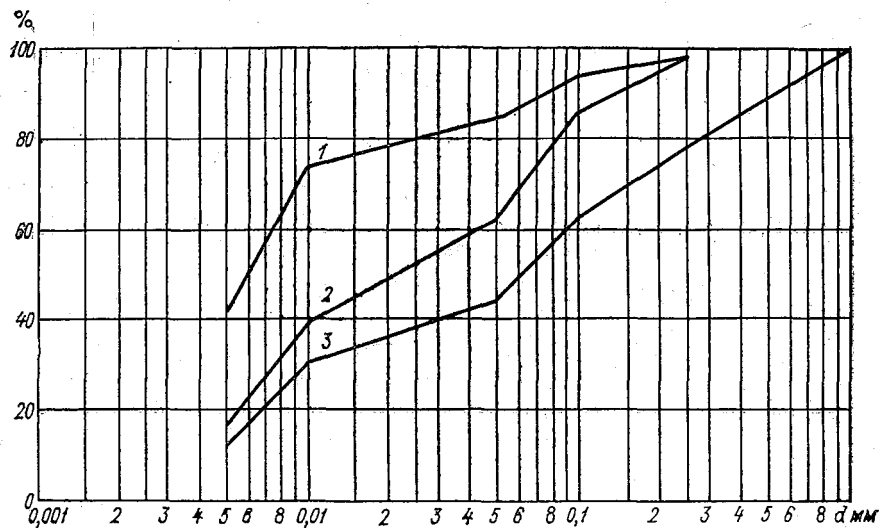
Рис. 8.7. Кривые гранулометрического состава наносов рек, осредненные за год (1957 г.).
