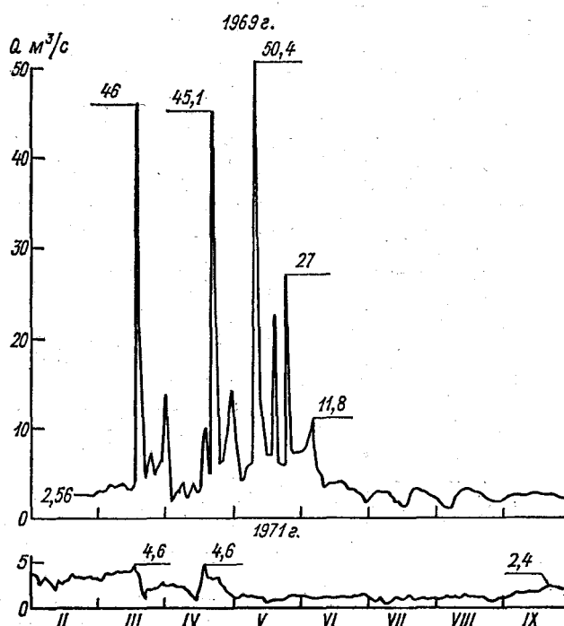
Рис. 5.8. Гидрографы р. Хульм — Танги-Ташкурбан.
