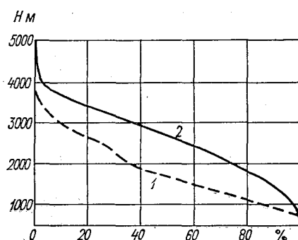
Рис. 3.3. Гипсометрические кривые бассейнов рек Гильменд (1) и Герруд (2).
