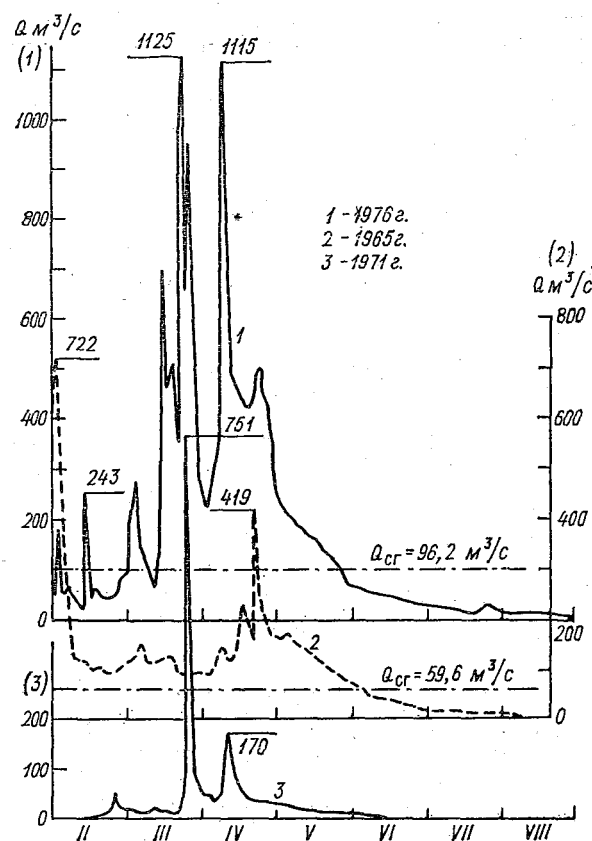
Рис. 5.16. Гидрографы р. Фарахруд — Петч-Танги.
