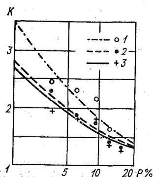
Характеристики максимальных расходов рек подзоны Б 1 (север)
