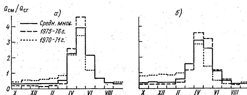
Рис. 5.18. Гидрографы среднемесечных расходов р. Гильменд за многоводный, маловодный годы и средний многолетний.
