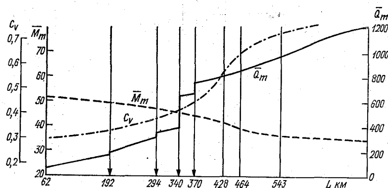
Рис. 6.13. Изменение характеристик максимальных расходов по течению р. Фарах-руд.
