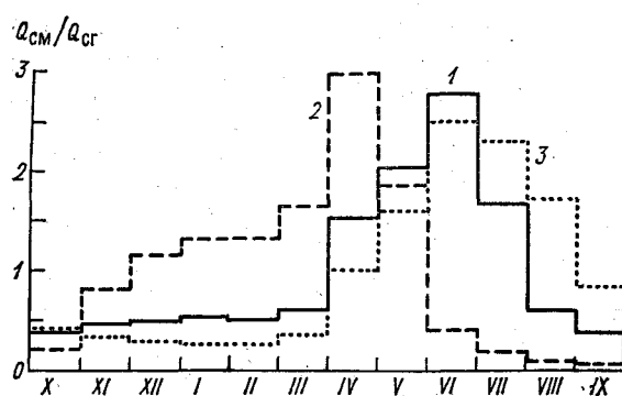
Рис. 5.1. Среднемноголетний гидрограф р. Кабул.
