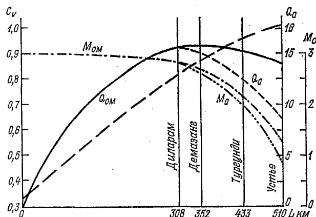
Рис. 4.31. Изменение основных характеристик р. Хашруд от истоков до устья.
