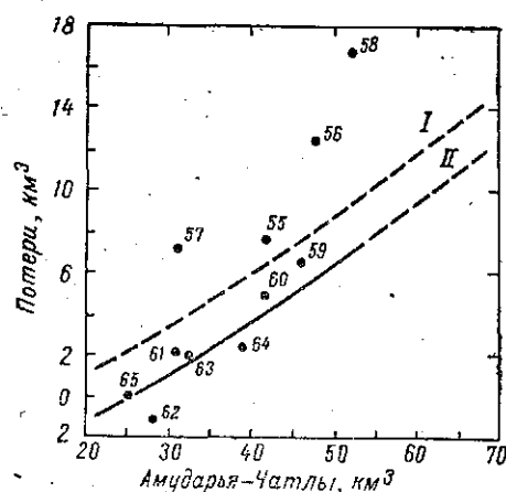
Рис. 2. Связь потерь стока в дельте Амударьи и ее стока у кишла. Чатлы за период 1955—65 гг.:
