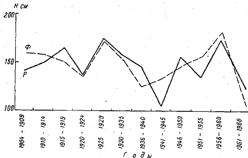
Рис. 2. Рассчитанные (Р) и фактические (Ф) средние уровни Аральского моря по 5-6-летиям со сдвигом на один год
