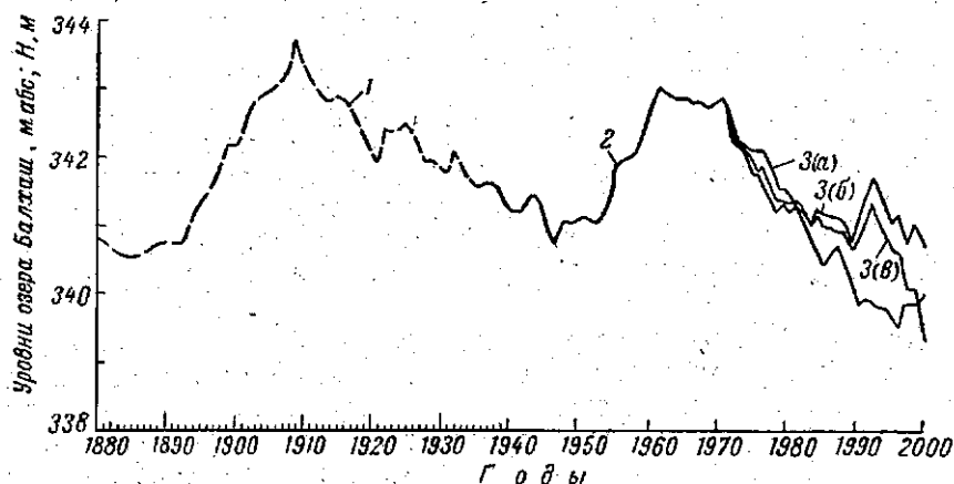
Рис. 7. Колебания уровня оз. Балхаш за период 1879—2000 гг.: 1 — восстановленные, 2 — наблюдаемые 3а, 3б, 3в — рассчитанные значения вариантов 1, 2, 3 соответственно
