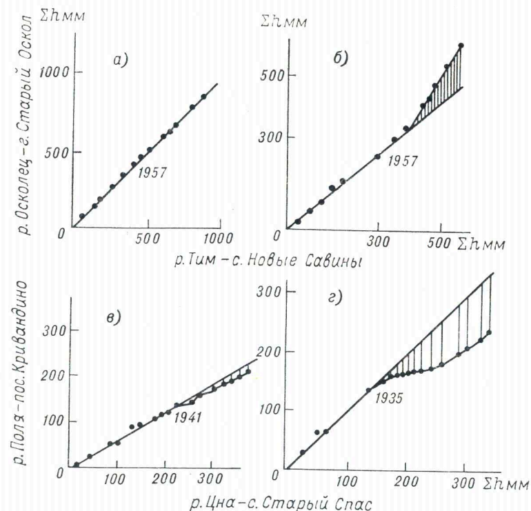
Рис. 58. Связь между интегральными суммами стока рек-аналогов и рек с нарушенным водным режимом для весеннего (а, в) и межennaleго (б, г) периодов.
