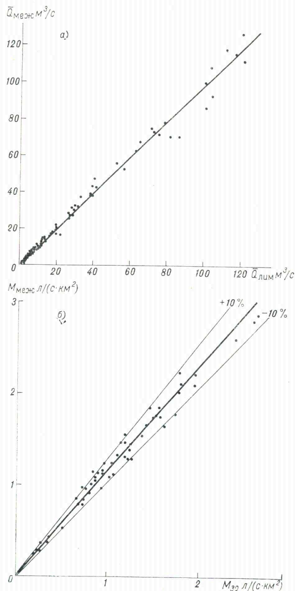
Рис. 40. Связь зимних межного и лимитирующего расходов воды (а), межного и минимального 30-дневного модулей стока (б).
