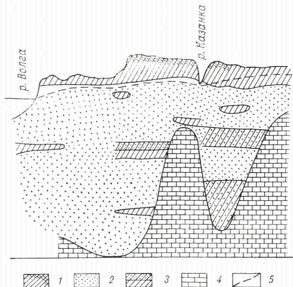
Рис. 8. Гидрогеологический профиль долины р. Казанки [98].
