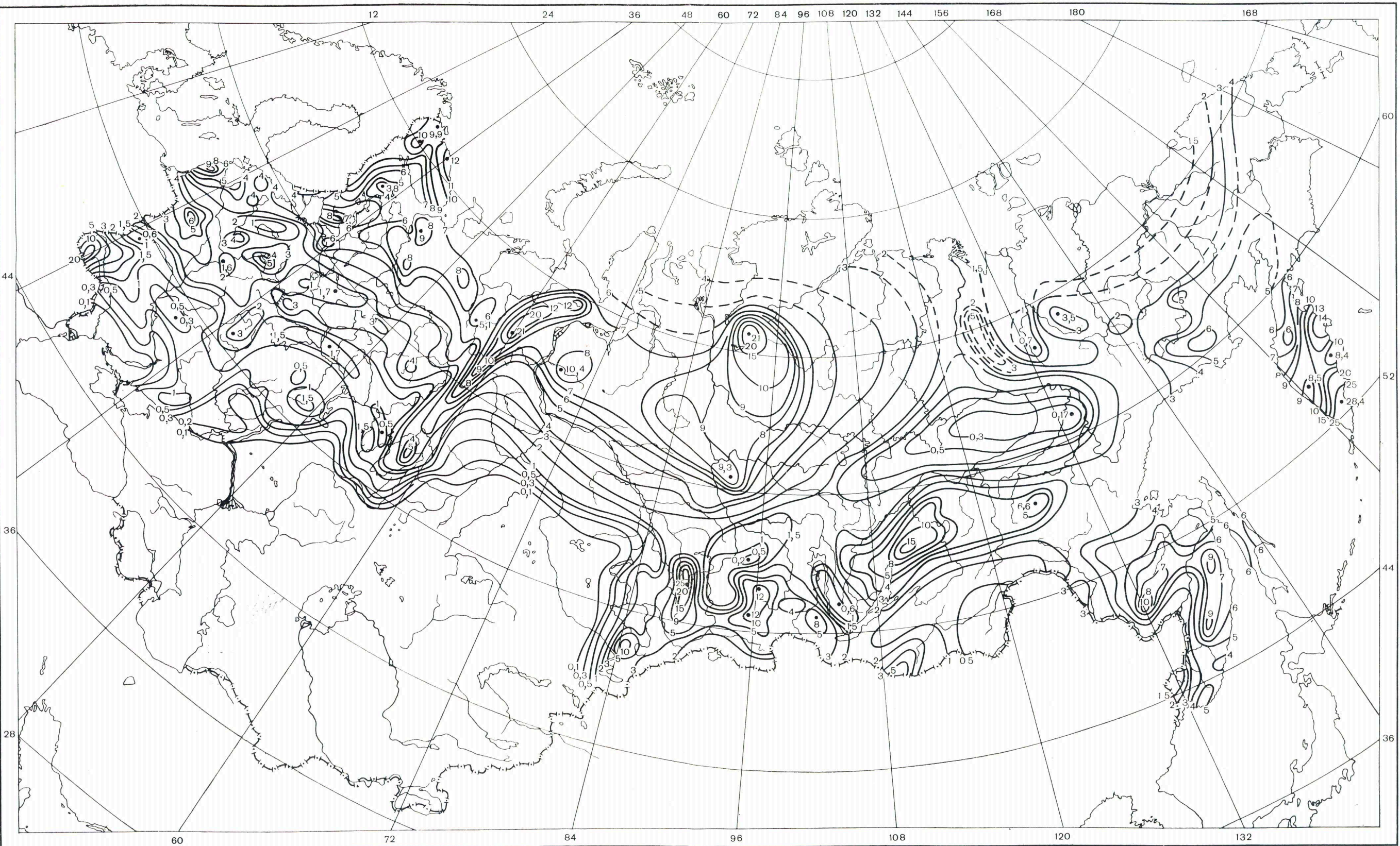
Рис. 37. Карта стока 75%-ной обеспеченности (л/(с·км²)) за маловодный сезон.
