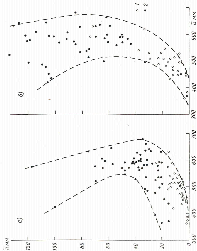
Рис. 5. Зависимость стока лимитирующего (а) и маловодного (б) сезонов от среднегодовой инфильтрации для ЕТС.
