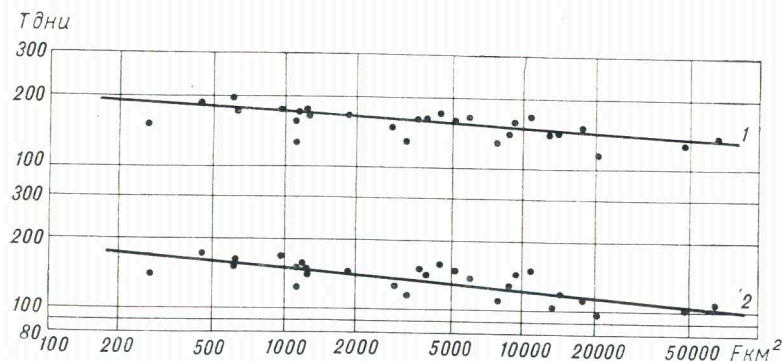
Рис. 61. Зависимость продолжительности ежегодного промерзания рек от размеров бассейна (бассейны рек Витим, Оленек). Продолжительность промерзания; 1 — наибольшая, 2 — средняя.
