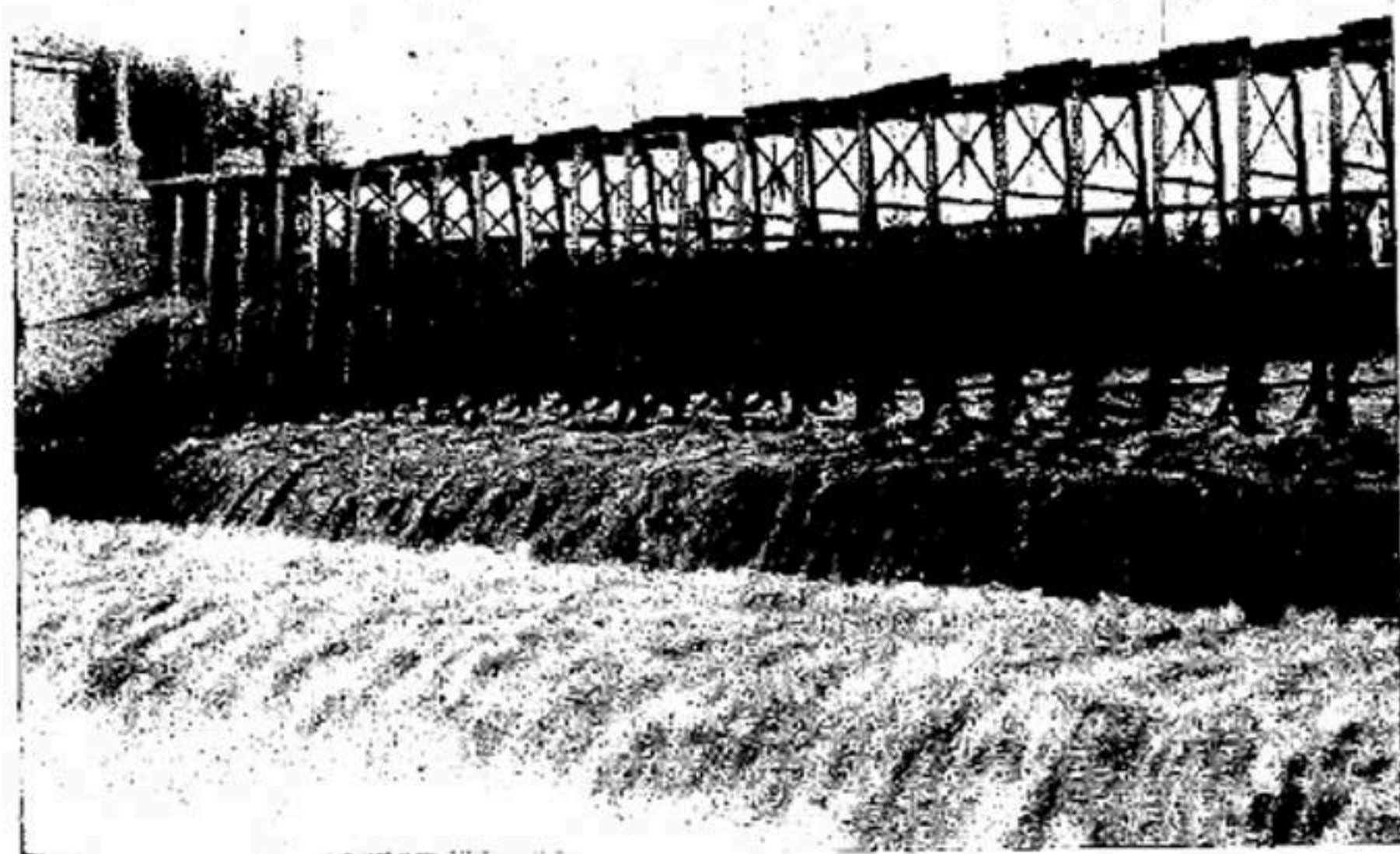
Гиндыкушская плотина.
