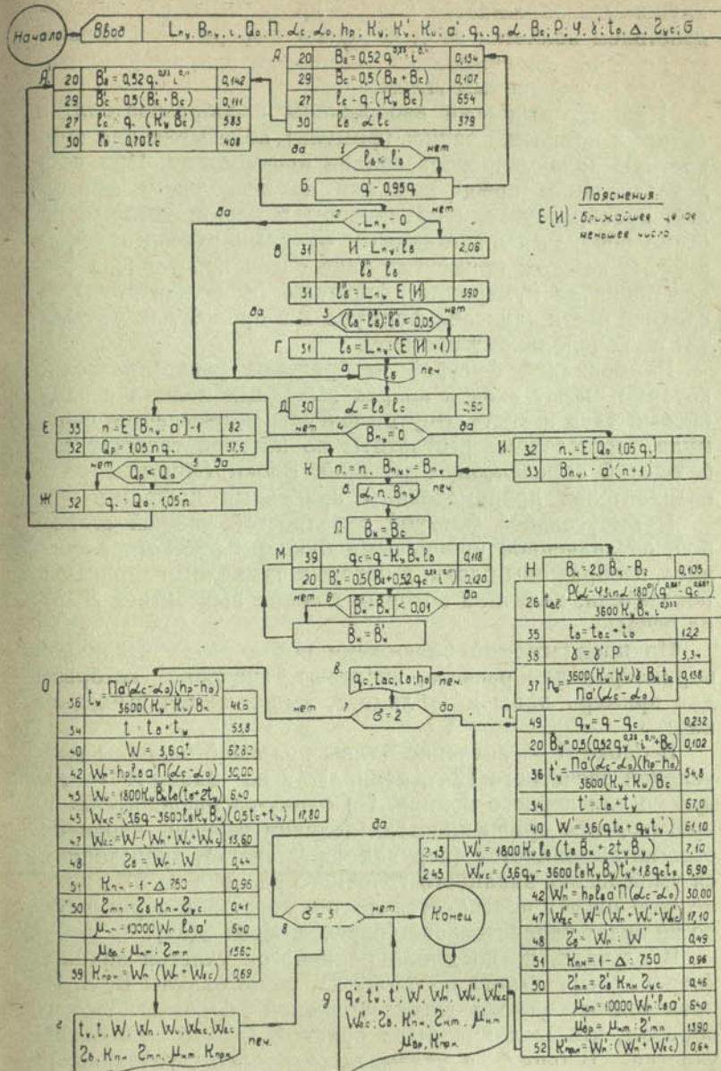
Рис. 15. Блок-схема порядка расчета элементов техники полива по бороздам.
