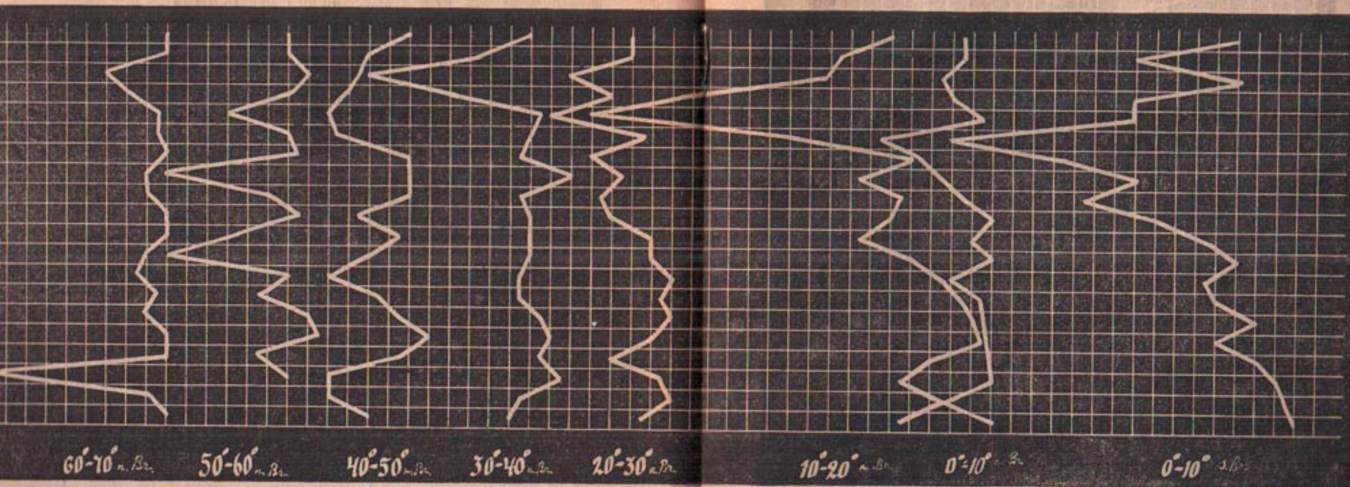
Рис. 4. Многолетний ход напряженности вулканизма, разложенный на пояса. Видно передвижение max. волны IV порядка от экватора к полюсу.
