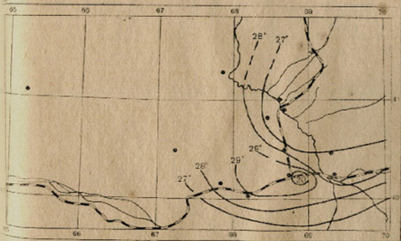
Рис. 12. Изотермы июля.
