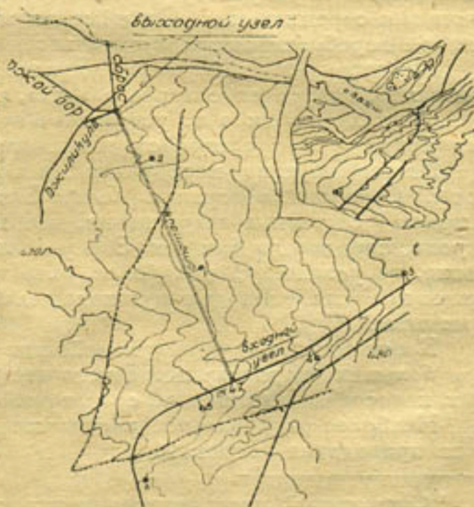
Рис. 1. План головного участка магистрального канала и Северной ветви.
