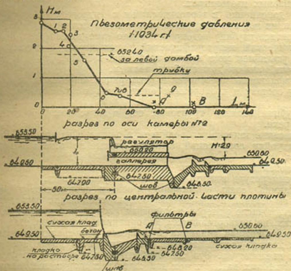
Рис. 9. Разрезы плотины и эюра пьезометрического уклона при H = 2,9 м. Крестиками показаны наблюдения для пьезометра № 9 и для погруженных в основание под плотиной в точках А и В.
