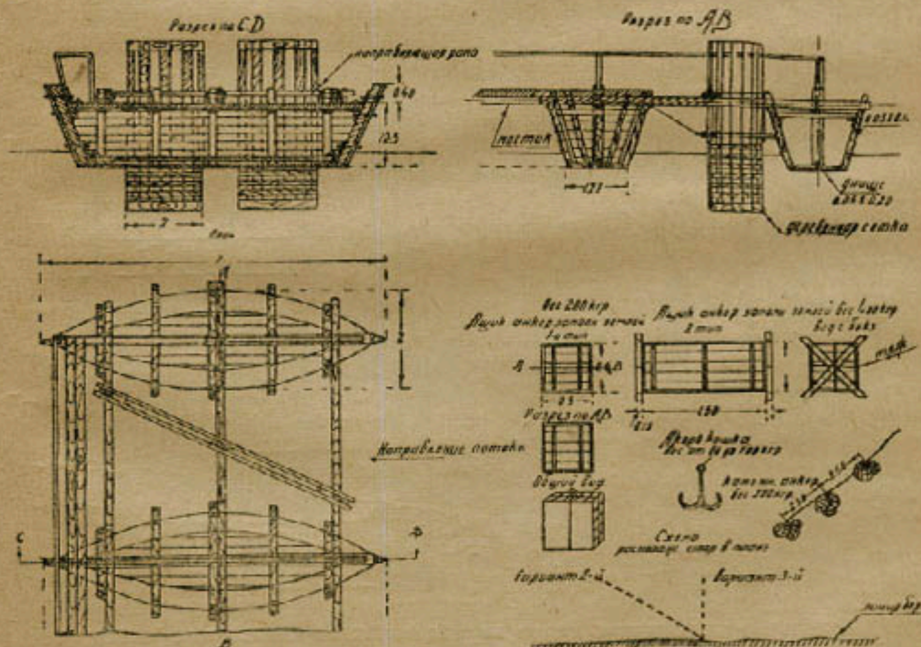
Рис. 1. ловушечный снаряд заилитель с выдвижными сетками конструкции Харлампиева
