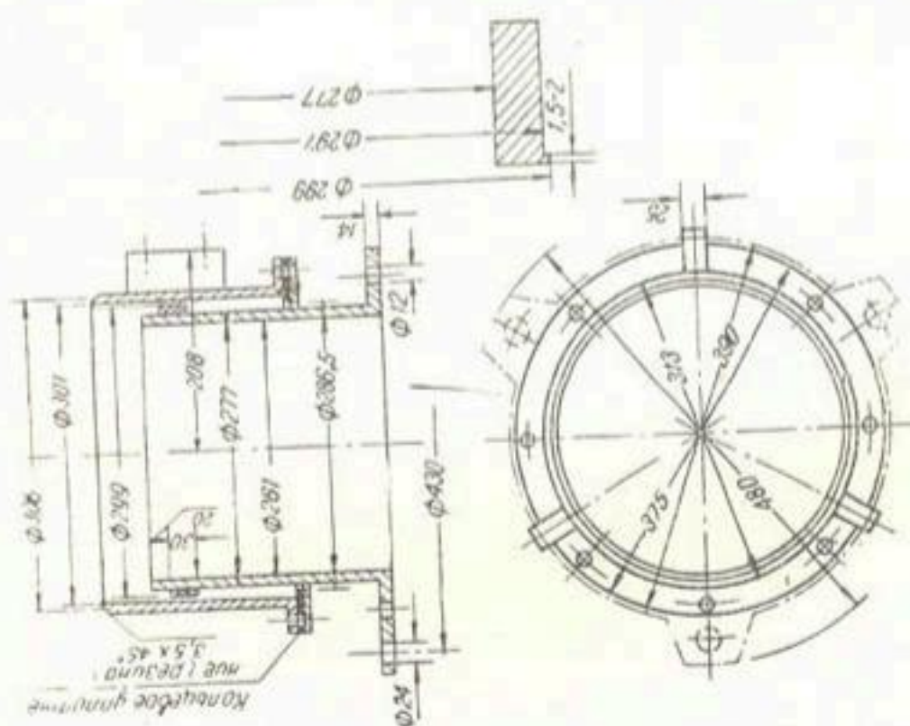
Рис. 3. Конструкция подвижного шлангра.
