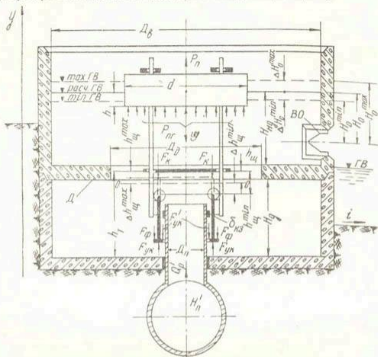
Рис. 2. Железобетонный подовыпуск и расчетная схема автомата-регулятора расхода.
