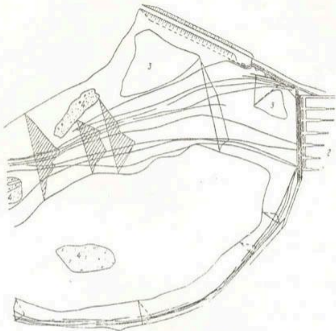
Рис. 6. Схема верхнего бьефа плотин во время его промыва с показанием движения поверхностных струй. 1—плотина, 2—камеры отстойника, 3—подводные отмели, 4—остров. Заштрихованы—строительные отвальные отмели.
