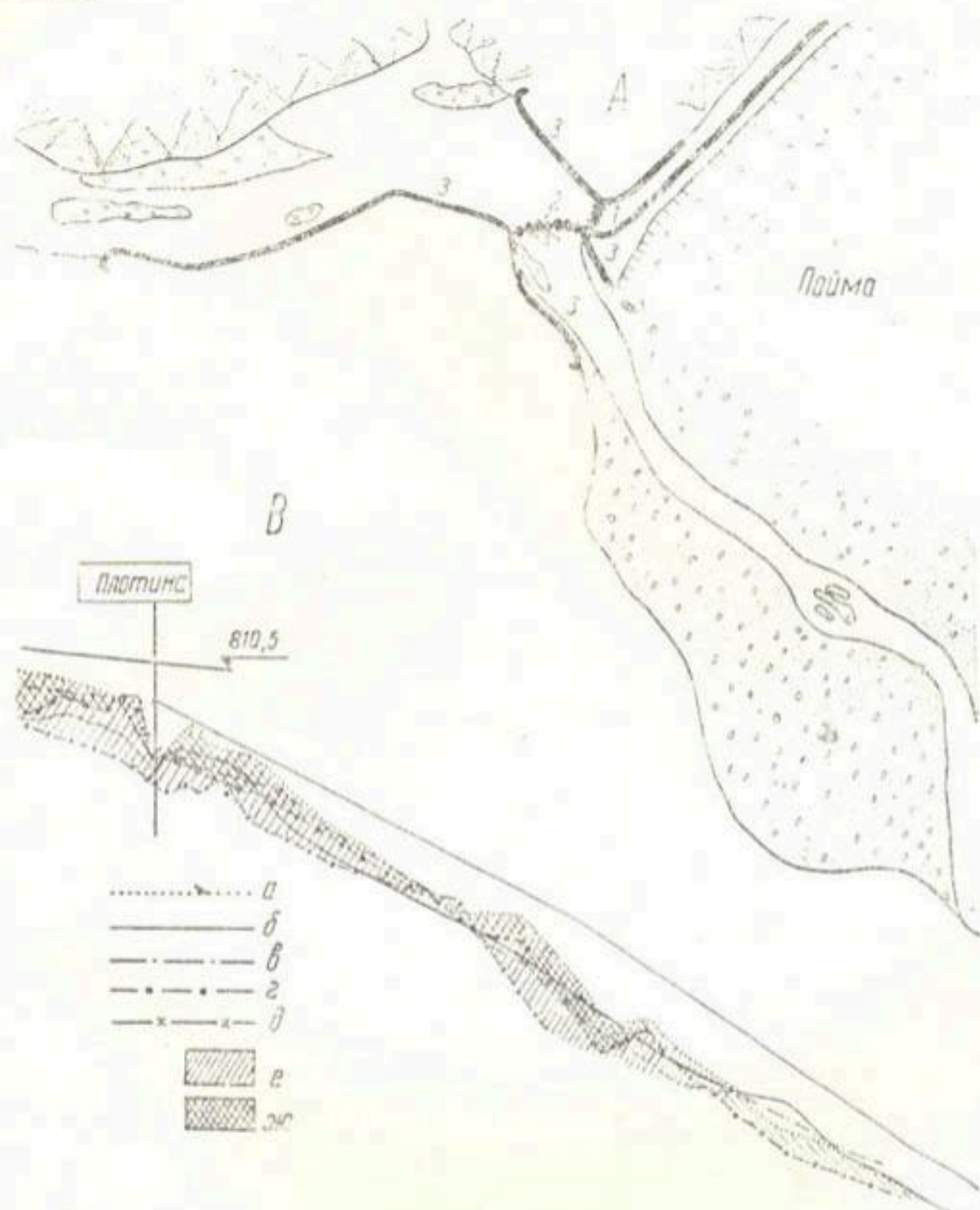
Рис. 11. Схема (А) и продольный профиль (В) русла р. Карадарьи у Камширраватской плотины (20.VII 1953), Q = 125 \text{ м}^3/\text{сек.}
