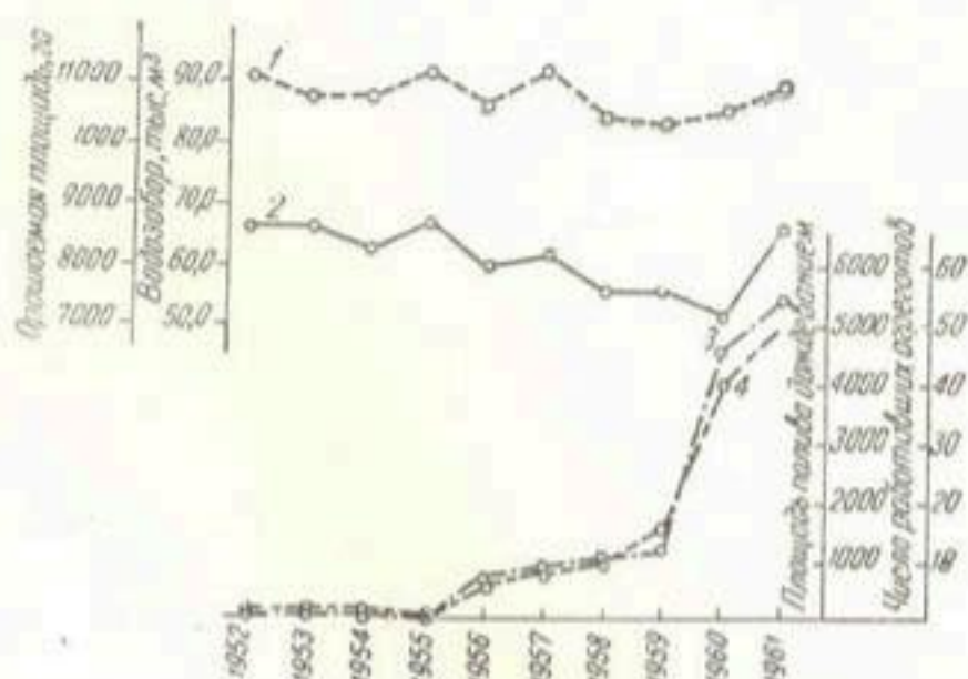
Рис. 3. Динамика водопользования при дождевании. 1—поливная площадь, га, 2—водозабор, тыс. м³, 3—площадь полива дождеванием, га, 4—количество работающих агрегатов ДДА-100 М.
