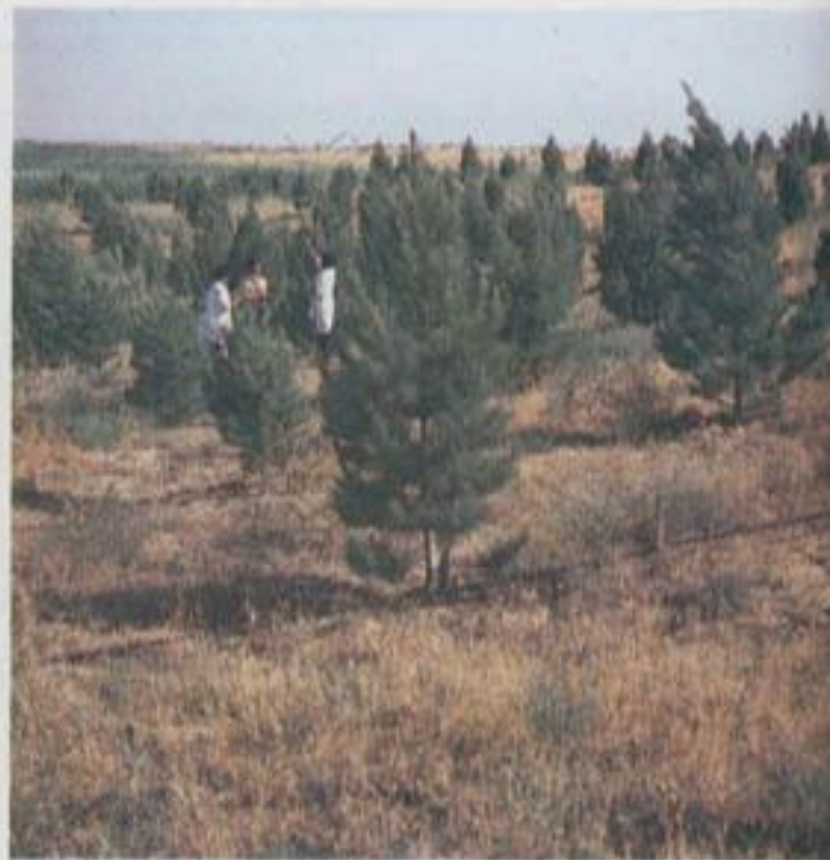
Капельное орошение — самый экономичный и эффективный способ орошения в условиях аридных районов
