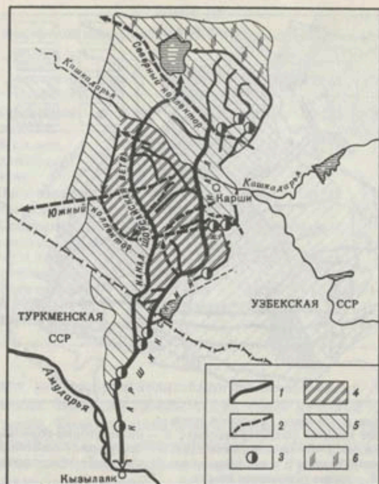
Рис. 17. Орошение Каршинской степи 1 — оросительные каналы (магистральные); 2 — коллекторно-сбросные (главные) каналы; 3 — насосные станции; 4 — земли первоочередного орошения; 5 — зона перспективного орошения
