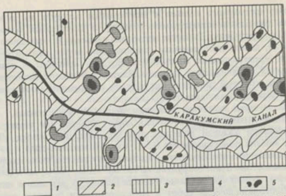
Рис. 10. Схема изменения природных условий в зоне Каракумского канала (по Н.Г. Харину, 1976) 1 - разбитые пески вдоль трассы канала, 2 - полувзрослые пески, 3 - заросшие пески, 4 - болота, 5 - фильтрационные озера
