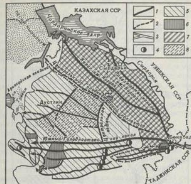
Рис. 16. Орошение и освоение Голодной степи 1 — оросительные каналы (магистральные); 2 — коллекторно-сбросные каналы; 3 — деривационный канал; 4 — насосные станции; 5 — хлопковые севообороты; 6 — овоще-кормовые севообороты и многолетние насаждения; 7 — существующее орошение (старая зона); 8 — вновь освоенные земли
