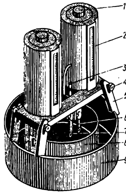
Рис. 14. Прибор ПВН-00 для определения водопроницаемости почв и грунтов: 1 – пробка; 2 – бачок; 3 – отвес; 4 – гайки; 5 – штатив; 6 и 7 – патрубков; 8 и 9 – рамы
