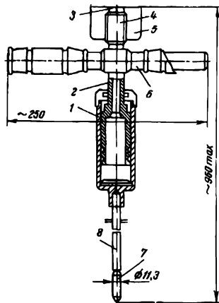
Рис. 12. Твердомер Алексеева:
