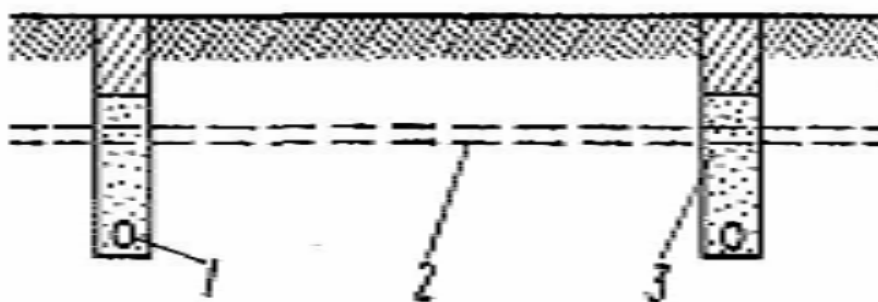
Рис.16.1 Комбинированный дренаж: 1 – гонимая дрена; 2 – кротовина, 3 – фильтрующая засыпка
