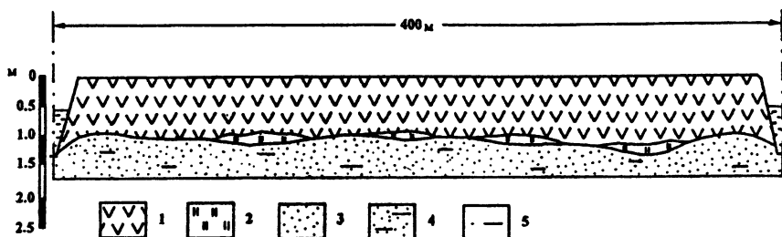
Рис. 3. Почвенно-литологический профиль польдера «Макеевский мыс». 1 — торф; 2 — сапропель; 3 — песок; 4 — включение тонких прослоек легкого суглинки; 5 — оси дренажных каналов
