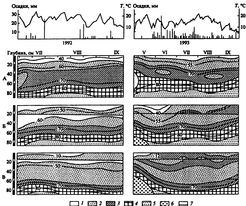
Рис. 20. Категории и хроноизоплеты влажности (в % от объема) осушенных торфяных почв полейдера «Макеевский мыс». Варианты А — черная культура (контроль); Б — пескование; В — покровная культура. Категория влаги: 1 — менее 0,7 НВ; 2 — 0,7 НВ—НВ; 3 — НВ—0,9 ПВ; 4 — 0,9 ПВ—ПВ; 5 — грунтовые воды; 6 — мерзлота; 7 — нижняя граница пахотного горизонта
