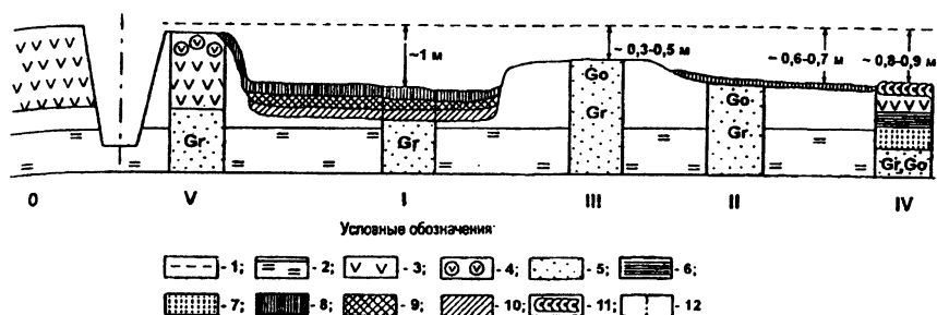
Рис. 11. Схематический профиль сгоревшего торфяного массива на территории пolderа «Макеевский мыс» и структура пирогенных образований.
