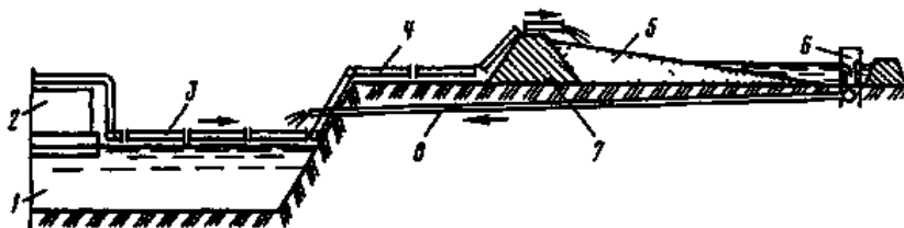
Рис. 4.17. Схема обустройства приканальных площадей при подготовке их для складирования наносов (грунта), удаленных из канала земснарядом: 1 – канал; 2 – земснаряд; 3 и 4 – плавучий и береговой пульпопроводы; 5 – отвал удаленных из канала наносов (грунта); 6 – водосбросной колодец; 7 – дамбы обвалования; 8 – водосбросная труба (лоток).
