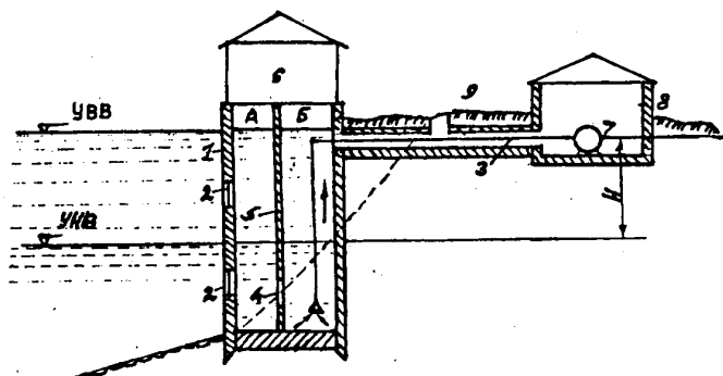
Рис. 7.2. Раздельный водоприемник берегового типа: А – водопроводное отделение; Б – всасывающее отделение; 1 – водоприемный колодец; 2 – водоприемные окна; 3 – всасывающие трубы; 4 – сетки; 5 – перегородка; 6 – служебный павильон; 7 – насосы; 8 – насосная станция; 9 – галерея.
