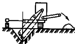
Рис. 4.8. Экскаватор ЭМ-152 Б с многоковшовым оборудованием (гусеницы машины расположены по обеим сторонам канала).
