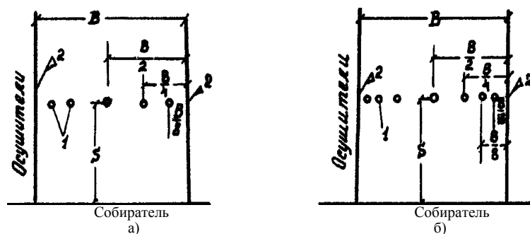
Рис. 2.4. Схемы расположения наблюдательных колодцев в гидрометрическом створе: а – при пяти колодцах; б – при семи колодцах; 1 – наблюдательные колодцы; 2 – вспомогательные гидрометрические посты на открытом канале-осушителе.
