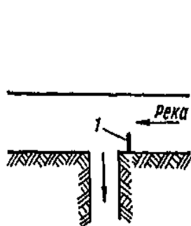
Рис. 5.12. Донный порог (1) перед головной частью магистрального канала.
