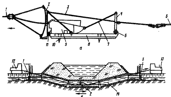
Рис. 4.22. Ковш-рыхлитель КР-2 для очистки дюкеров (а) и (б) схема его рабочих перемещений: 1 и 5 – тяговые тросы; 3 и 7 – растяжки; 4 – рычаг; 6 и 11 – шарниры; 8 – рама; 9 – полость; 10 – рыхлящие зубья; 12 и 13 – тракторы; 14 – дюкер.
