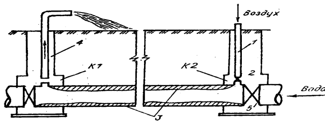
Рис. 7.9. Схема гидropневматической промывки трубопровода: 1 – воздухопровод; 2 – задвижка для впуска воздуха в промываемый участок; 3 – отложения на стенках трубы; 4 – отвод промывной воды; 5 – задвижка.
