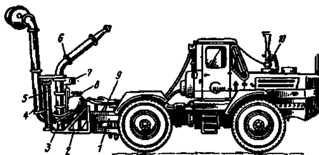
Рис. 5.8. Дальнеструйный навесной дождеватель ДДН-100 на тракторе Т-150 К: 1 – разгрузочные цепи; 2 – рама; 3 – насос-редуктор; 4 – всасывающий трубопровод; 5 – гидроцилиндр; 6 – ствол; 7 – механизм поворота ствола; 8 – приспособление для внесения удобрений; 9 – карданный вал с кожухом; 10 – газоструйный вакуум-аппарат.
