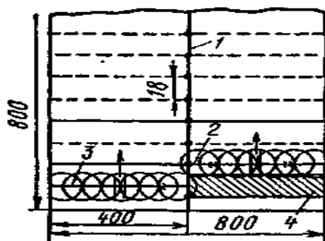
Рис. 5.3. Технологическая схема работы дождевальной машины “Волжанка”: 1 – закрытый или разборный оросительный трубопровод; 2, 3 – первое и второе крылья; 4 – поливаемая площадь (размеры в м).
