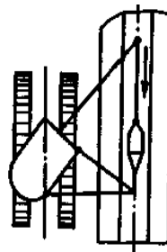
Рис. 4.10. Схема работы экскаватора с оборудованием боковой драглайн.
