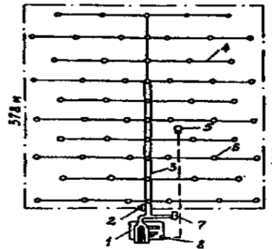
Рис. 5.11. Схема синхронного импульсного дождевания: 1 – насосная станция; 2 – гидроподкормщик; 3 – 4 – трубопроводная сеть; 5 – датчик; 6 – аппараты импульсного дождевания; 7 – генератор командных сигналов; 8 – пульт управления.
