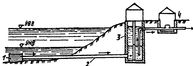
Рис. 7.3. Русловой водоприемник: 1 – оголовок; 2 – самотечная линия; 3 – береговой колодезь; 4 – насосная станция.
