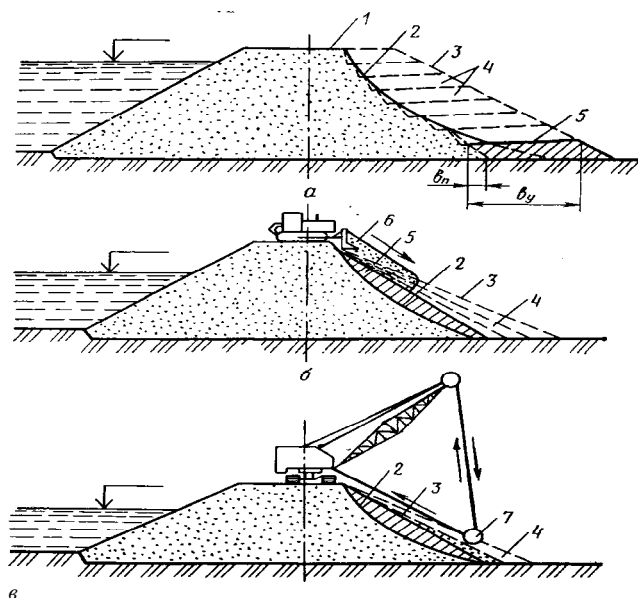
Рис. 9.3. Схема уширения и улоаживания откосов грунтовых плотин: а и б – продольный и поперечный способы; в – уплотнение грунта катком; 1 – гребень плотины; 2 – низовой откос до ремонта; 3 – проектный откос; 4 – слой отсыпки и уплотнение грунта; 5 – уплотненный грунт; 6 – грунт, разравниваемый бульдозером; 7 – каток.
