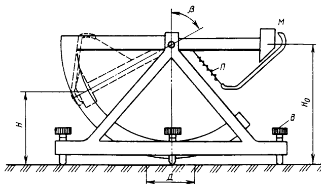
Рис. 6.13. Прибор для определения сцепления колес автомобиля с покрытием: М – груз; В – регулировочный винт; П – пружина; H_0 – начальная высота подъема груза; D – диаметр следа колеса; \beta – угол отклонения маятника.
