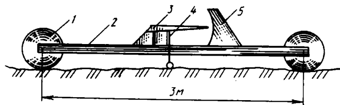
Рис. 6.6. Колесная рейка: 1 – опорное колесо; 2 – рейка; 3 – стрелка; 4 – шток с контрольным колесиком; 5 – шкала.
