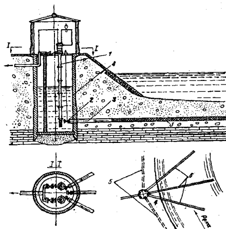
Рис. 7.1. Подрусловой лучевой дозатор: 1 – вертикальный насос; 2 – задвижка; 3 – фильтровая перфорированная труба; 4 – водосборная шахта; 5 – береговые лучи; 6 – речные
