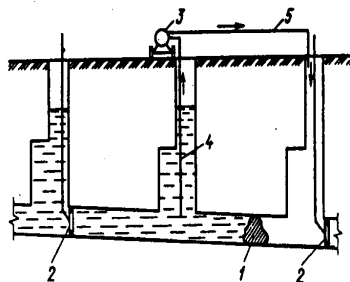
Рис. 7. 16. Схема удаления засора методом обратного давления: 1 – засор; 2 – щитовые пробки; 3 – насос; 4 – всасывающий трубопровод; 5 – подающий трубопровод.
