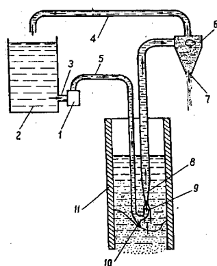
Рис. 7.4. Схема гидромеханической очистки шахтного колодца: 1 – насос; 2 – бак-отстойник; 3 – всасывающая труба насоса; 4 – сливная труба; 5 – напорный трубопровод; 6 – гидроциклон; 7 – отверстие для сброса песка; 8 – гидроэлеватор; 9 – насадка гидроэлеватора; 10 – размывающая насадка; 11 – очищаемый колодец.
