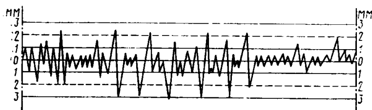
Рис. 6.8. Профиль, снятый виографом, и схема его анализа.
