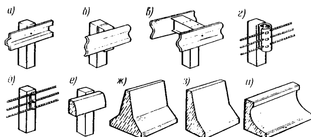
Рис. 6.16. Конструкция ограждающих устройств на автомобильных дорогах: а, б, в – из стальных профилей полос; г, д – тросовые; е, ж, з – бетонные; и – железобетонные парапетного типа.
