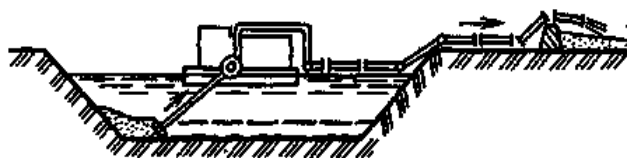
Рис. 4.16. Удаление наносов плавучей землесосной установкой.
