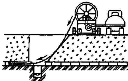
Рис. 4.18. Промывка дренажных и коллекторных труб от наносов дренажно-промывочной машиной (Д-910, ПДТ-125 и др.).
