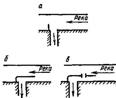
Рис. 5.13. Водозахватная шпора: а – простая; б – улучшенная; в – с промывным отверстием.
