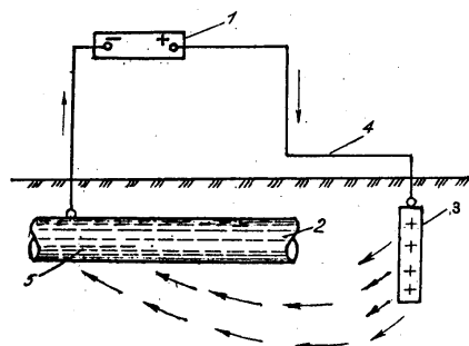
Рис. 7.10. Схема катодной защиты трубопровода от коррозии: 1 – источник постоянного тока; 2 – стальная труба; 3 – заземление (аноды); 4 – соединительные провода; 5 – катодная зона.
