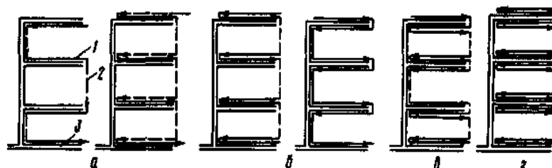
Рис. 4.4. Схемы рабочих перемещений экскаваторов и каналоочистителей: а, б, в, г – соответственно при одном, двух, трех и четырех проходах; 1 и 2 – рабочее и транспортное перемещения; 3 – канал.
