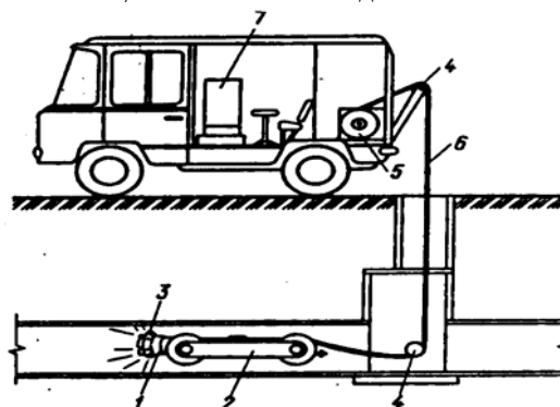
Рис. 7.11. Схема обследования канализационной сети телевизионной установкой: 1 – телекамера; 2 – самоходная тележка; 3 – осветительная насадка; 4 – направляющие ролики; 5 – лебедка; 6 – телекабель; 7 – пульт.
