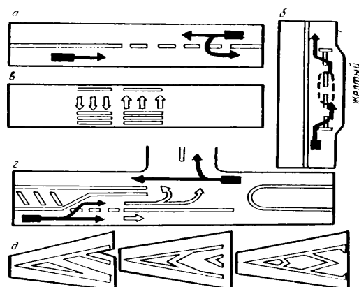
Рис. 6.19. Разметка проезжей части: а – направление движения; б – остановка автомобилей; в – пешеходный переход; г – перестроение потоков; д – направление движения по полосам.
