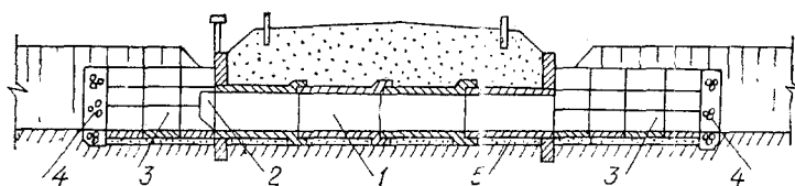
Рис. 2.23 - Шлюз-регулятор с переездом на осушительном канале:
