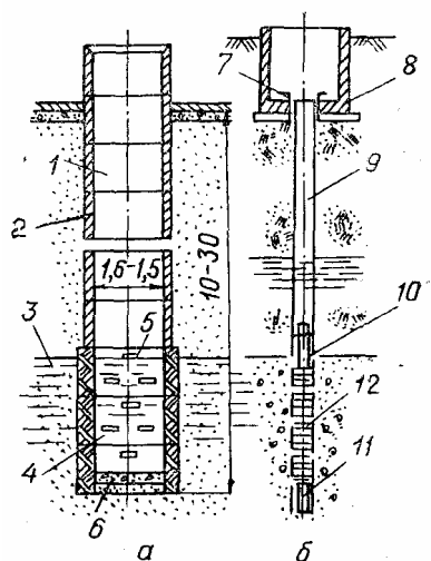
Рис. 2.53 - Схемы шахтного (а) и трубчатого (б) колодцев:
