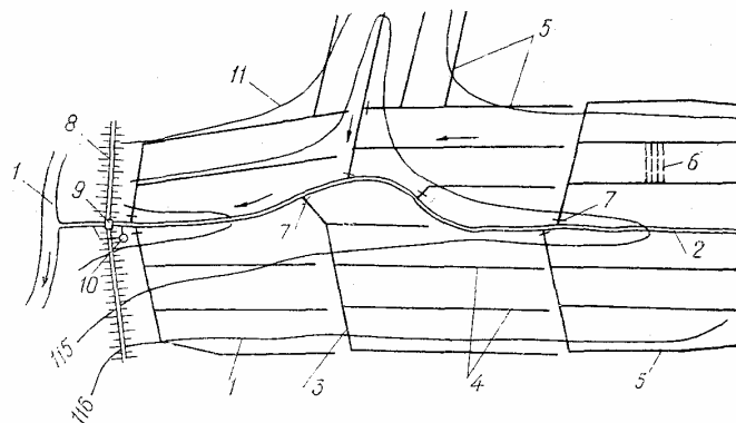
Рис. 2.1 - Схема полевой осушительной системы на пойменных землях:
