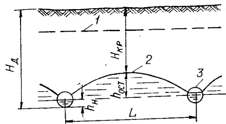
Рис. 2.63 - Схема понижения уровня грунтовых вод горизонтальным дренажом: 1,2 - уровень грунтовых вод соответственно до и после строительства дренажа; 3 - горизонтальные дренажи; H_d - глубина заложения дренажа; H_{кр} - критическая глубина залегания грунтовых вод; h_{ост} - остаточная глубина залегания грунтовых вод; h_n - глубина наполнения дренажа
