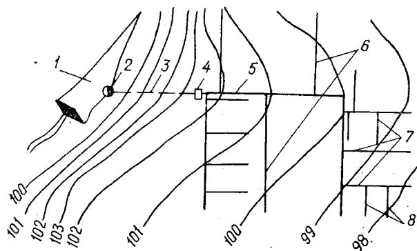
Рис. 2.38 - Схема расположения межхозяйственной сети на водораздельной равнине:
