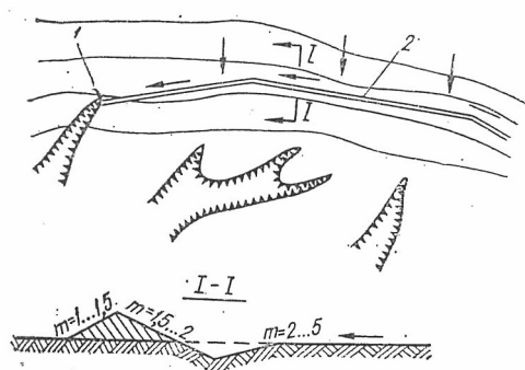
Рис. 3.15 - Водоотводящие валы-канавы: 1 – водосбросное сооружение; 2 – водоотводящий вал-канавы
