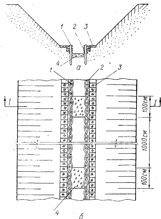
Рис. 2.21 - Крепление канала плетнем с отсыпкой щебнем по дну: а - сечение I-I; б - план; 1 - кольца d = 5...10 см, длиной 80...100 см; 2 - плетневая стенка высотой 30...50 см; 3 - дрен; 4 - отсыпка щебнем слоем 10 см
