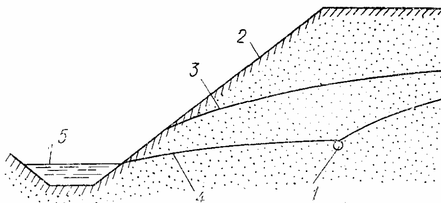
Рис. 2.22 - Схема работы разгрузочной дрены: 1 – разгрузочная дрена; 2 – откос канала; 3- депрессионная кривая до устройства разгрузочной дрены; 4 - депрессионная кривая при наличии разгрузочной дрены; 5- уровень воды в канале
