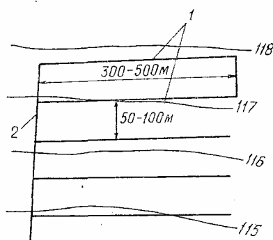
Рис. 2.18 - Расположение в плане открытых собирателей: 1 - открытые собиратели; 2 - проводящий канал
