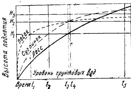
Рис. 28. Схематические кривые капиллярного подъема грунтовой воды различными грунтами (по С. И. Тюрменву)
