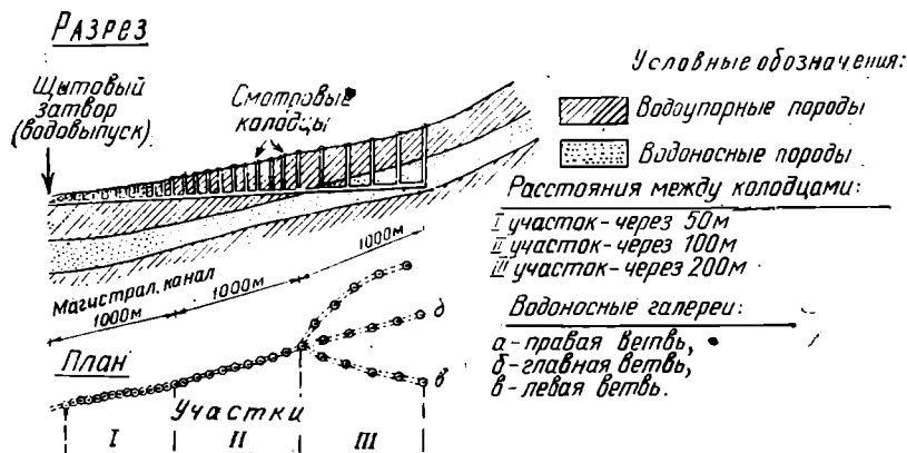
Рис. 35. Кяриз (схема устройства). По Б. Я. Стрелковскому
