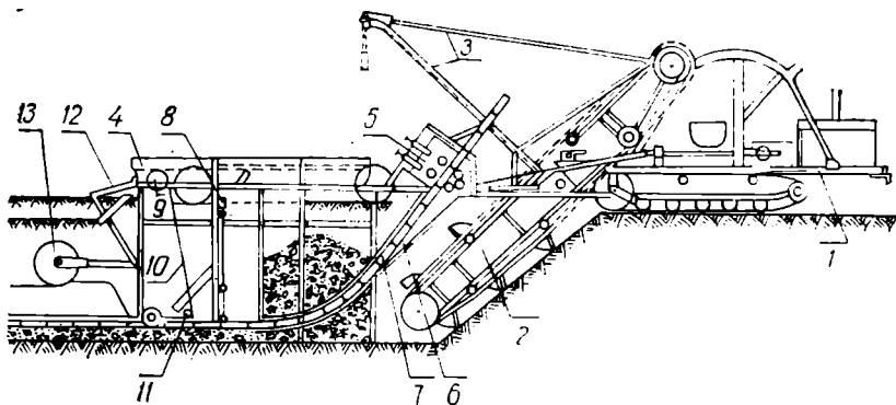
Рис. 76. Схема дренаукладчика:
