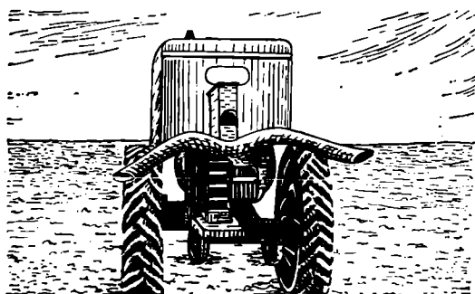
Рис. 110. Эжекторная сеялка СЭК-Т конструкции СредазНИИЛХ
