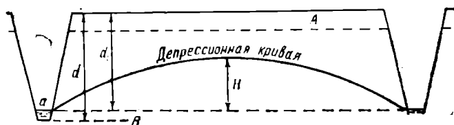
Рис. 64. Влияние дренажа на грунтовые воды:
