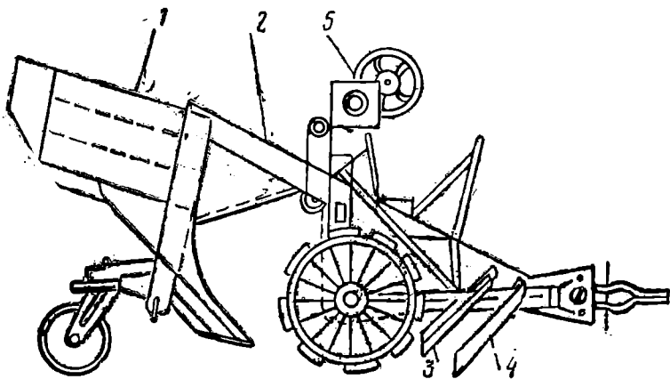
Рис. 68. Канавокопатель КМ-80У:
