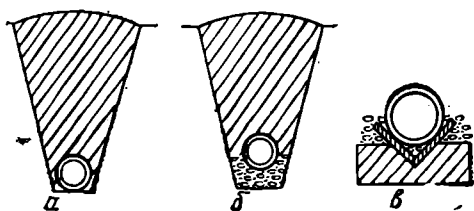
Рис. 71. Укладка дренажных труб:
