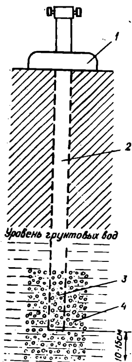
Рис. 29. Скважина для наблюдений за уровнем залегания грунтовых вод:
