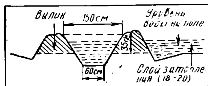
Рис. 55. Временный ороситель (ок-арык), устроенный палоделателем за два параллельных прохода
