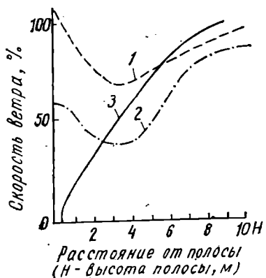
Рис. 45. Ослабление ветра лесными полосами различной ветропроницаемости (по П. А. Воронцову):
