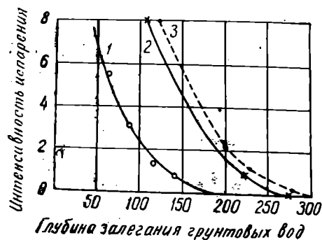
Рис. 6. Зависимость интенсивности испарения грунтовых вод от глубины их залегания (по В. А. Ковда):
