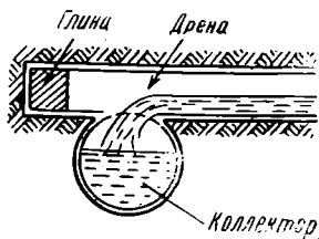
Рис. 73. Сопряжение трубы дрены и коллектора
