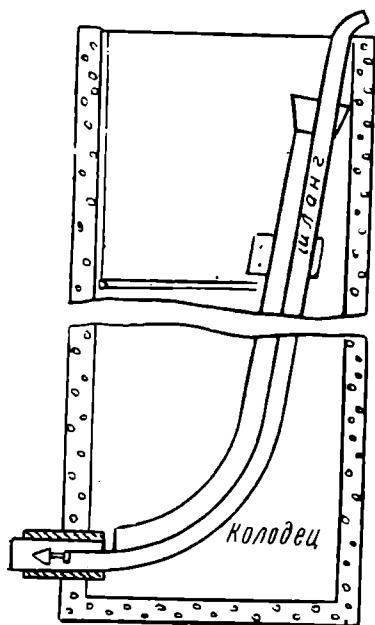
Рис. 79. Устройство для промывки закрытых дрен
