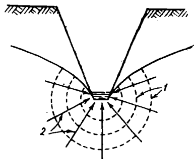
Рис. 63. Схема движения грунтовых вод к дренажу:
