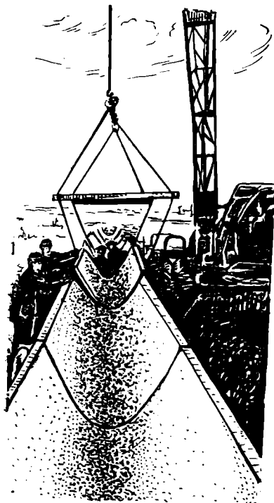
Рис. 32. Лотковый оросительный канал (установка лотков на опоры)
