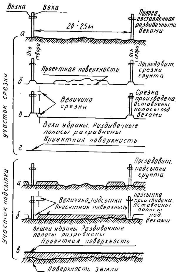
Рис. 38. Последовательность разработки полосы при ее планировке (по схеме „Узгипроводхоза“)
