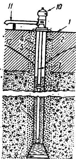
Рис. 82. Схема скважины вертикального дренажа:
