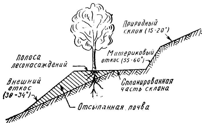
Рис. 99. Профиль террасы, построенной грейдером Д-20А
