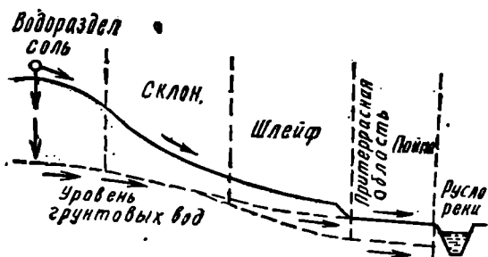
Рис. 3. Схема перераспределения солей по геоморфологическому профилю (по Л. П. Розову)
