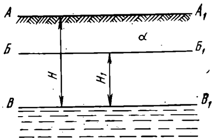
Рис. 27. Схема условий критического уровня минерализованных грунтовых вод (по Б. Б. Полюнову):
