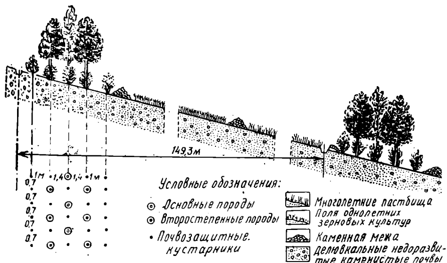
Рис. 96. Схема размещения лесных полос и водозадерживающих канав при севообороте с многолетними травами на богарных почвах при склоне 15^\circ (по ВНИАЛМИ)
