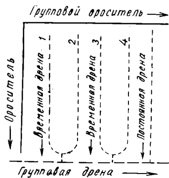
Рис. 69. Расположение временных мелких и постоянных глубоких дрен
