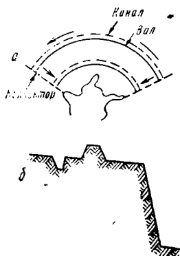
Рис. 100. Защита головы оврага: а — план; б — разрез
