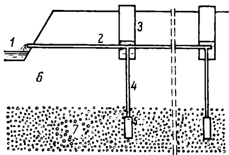
Рис. 75. Закрытая дрена со скважинами-усилителями:
