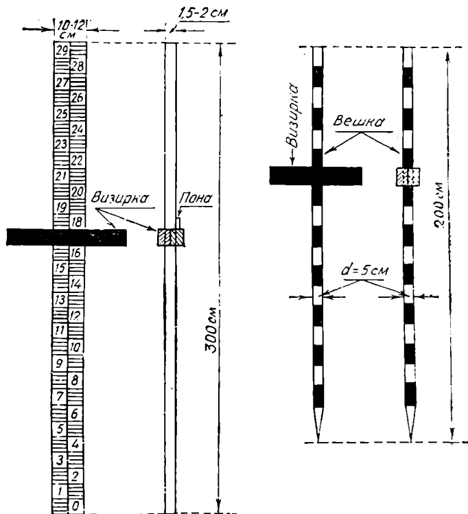
Рис. 39. Визирки для высотных отметок при планировочных работах
