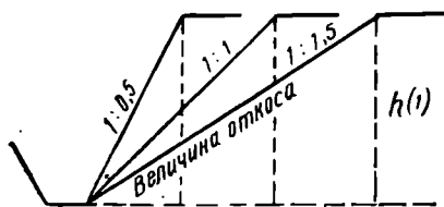
Рис. 62. Величина откосов: h — глубина дрены
