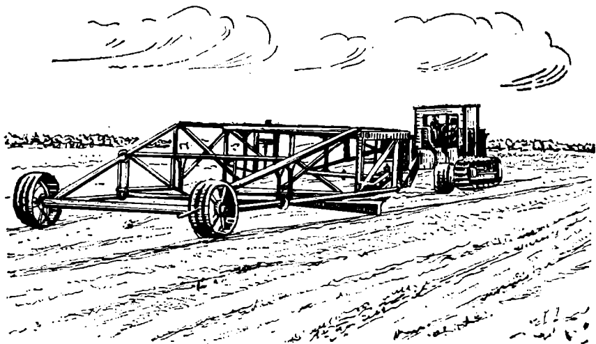
Рис. 44. Длиннобазовый планировщик
