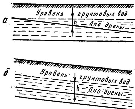
Рис. 66. Схема работы «перехватывающей» (а) и продольной б) дрен
