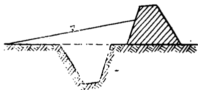
Рис. 101. Поперечное сечение канавы и вала
