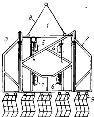
Рис. 43. Планировщик-разравниватель ПР-5:
