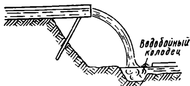
Рис. 102. Консольный перепад
