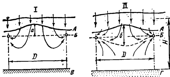
Рис. 70. Схемы отвода грунтовых вод закрытым дренажем (по С. Ф. Аверьянову):
