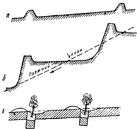
Рис. 97. Виды террас:
