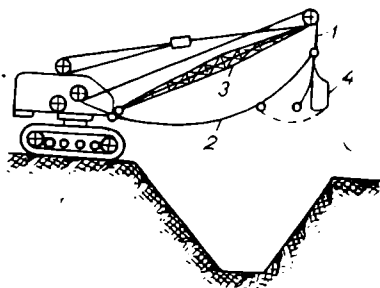
Рис. 61. Экскаватор драглайн: 1 и 2 — подъемный и тяговый канаты; 3 — стрела; 4 — ковш
