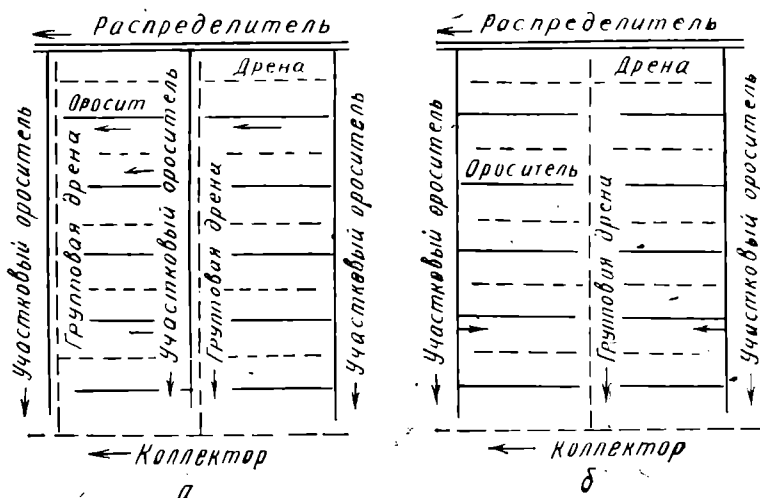
Рис. 67. Расположение оросительной и коллекторно-дренажной сети при одностороннем (а) и двустороннем (б) командовании участковых оросителей
