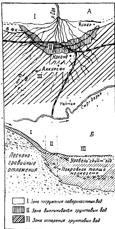
Рис. 4. Гидрогеологические зоны земель системы р. Сох (А — план; Б — в разрез)
