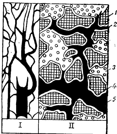
Рис. 7. Сеть крупных и мелких капилляров почвы (по Н. А. Качинскому):
