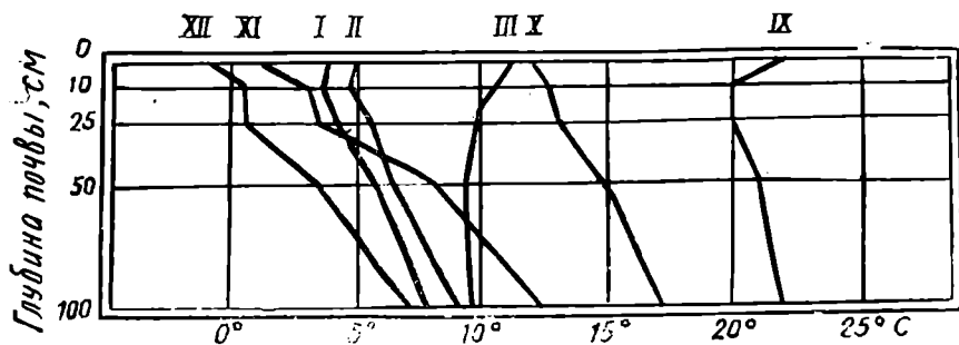
Рис. 52. Температуры почвы Голодностепской опытной станции (средние за месяц)
