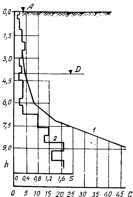
Рис. 60. Рассоление почв, грунтов и грунтовых вод под действием промывок и дренажа (Н. А. Беседнов):
