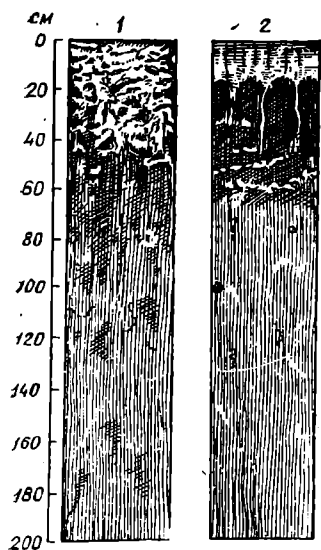
Рис. 13. Профили засоленных почв (по Г. Н. Самбуру):
