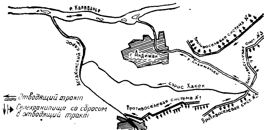
Рис. 103. Схема противоселевых сооружений у гор. Андижана
