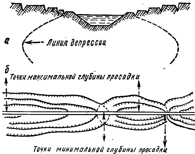
ис. 89. Схема образования (а) и планового расположения (б) просадок на канале
