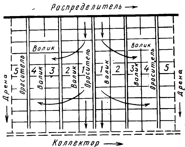
Рис. 56. Очередность промывки (1, 2, 3, 4, 5) и направление оттока солей к дренам и коллектору
