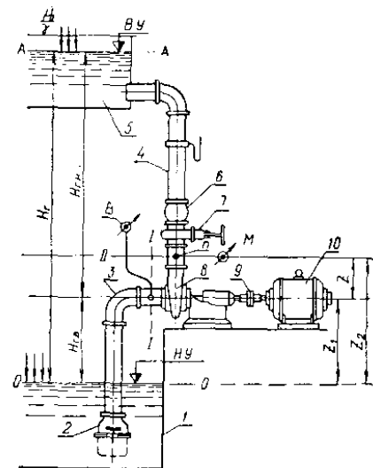
Рис. 15. Схема оборудования насосной установки: 1 — приемный резервуар; 2 — приемный клапан; 3 — всасывающий трубопровод; 4 — напорный трубопровод; 5 — напорный резервуар; 6 — обратный клапан; 7 — задвижка; 8 — насос; 9 — перекачка; 10 — двигатель.
