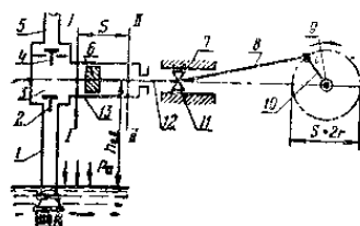
Рис. 13. Схема установки поршневого насоса одностороннего действия с кривошипным механизмом:
