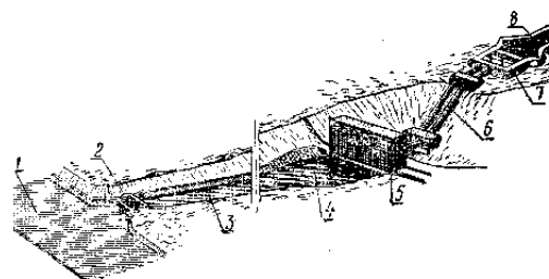
Рис. 8. Схема сооружений насосной станции: 1 — канал; 2 — водозаборное устройство; 3 — подводящий канал; 4 — аванкамера; 5 — здание насосной станции; 6 — напорный трубопровод; 7 — напорный бассейн; 8 — магистральный машинный канал.
