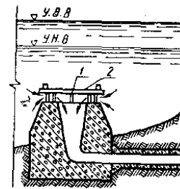
Рис. 50. Водозаборный оголовок крупных насосных станций: 1 — стойка; 2 — плита.
