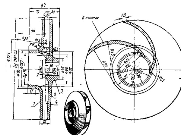
Рис. 28. Рабочее колесо с односторонним входом: 1 — средний диск; 2 — ступица; 3 — задний диск; 4 — лопасть.
