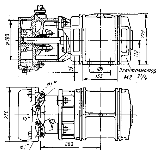
Рис. 101. Водокольцевой вакуум-насос КВН.
