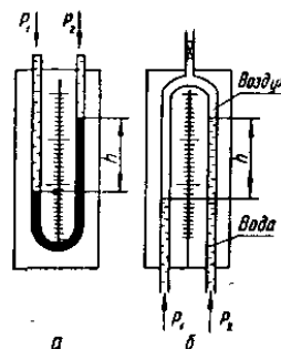
Рис. 91. Дифференциальные манометры: а — ртуть; б — вода.
