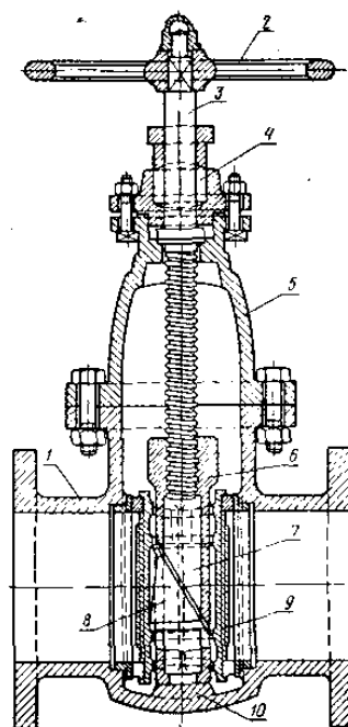
Рис. 78. Параллельная задвижка с неведвигимым шпинделем: 1 — корпус задвижки; 2 — маховик; 3 — шпиндель; 4 — сальник; 5 — крышка задвижки; 6 — гайка; 7, 8 — верхний и нижний клинья; 9 — диск; 10 — выступ корпуса.
