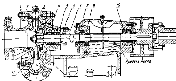
Рис. 17. Центробежный насос консольного типа: 1 — крышка; 2 — корпус; 3 — рабочее колесо; 4 — сальник; 5 — набивка; 6 — крышка сальника; 7 — вал; 8 — стойка; 9, 10 — подшипники; 11 — задний диск; 12 — отверстие; 13 — уплотнение.
