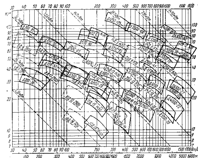
Рис. 16. Сводный график для подбора насосов типа Д и НД (ГОСТ 10272-73).
