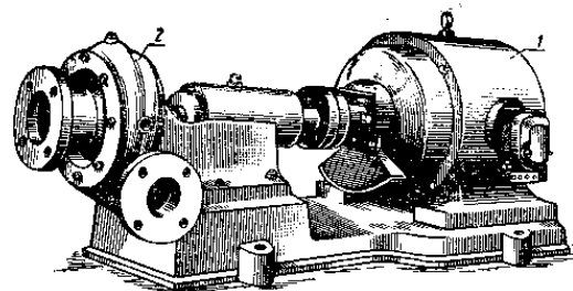
Рис. 99. Насос типа К на фундаментной плите: 1 — электродвигатель; 2 — насос.
