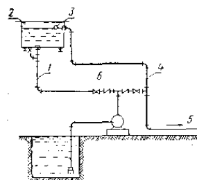
Рис. 100. Схема автоматического залива насоса из напорного бака:
