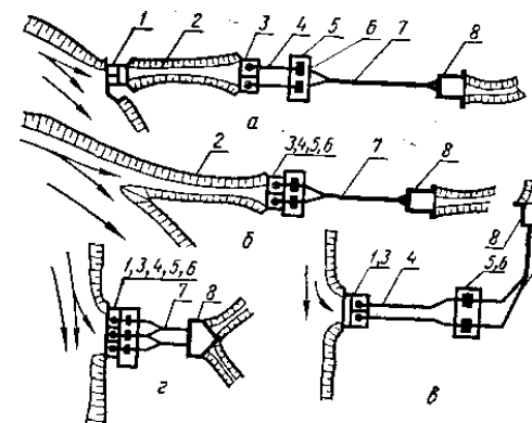
Рис. 49. Типичные схемы оросительных насосных станций: а и б — схемы насосной станции на отводящем (деривационном) канале; а — схема береговой насосной станции с раздельно устроенным зданием; б — схема береговой насосной станции с совмещенными сооружениями.
