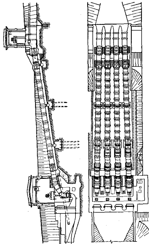
Рис. 55. Современное здание станции блочного типа с коленчатым водопроводом.
