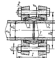
Рис. 74. Соединение асбестоцементных труб чугунной болтовой муфтой: 1 — чугунная муфта; 2 — резиновые кольца; 3 — резиновые кольца.
