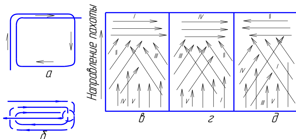
Рисунок 2.23 – Схемы движения планировщиков а – кольцевая; б – загонная; в, г, д – соответственно на 1, 2 и 3 участках; I – V – направление проходов планировщика
