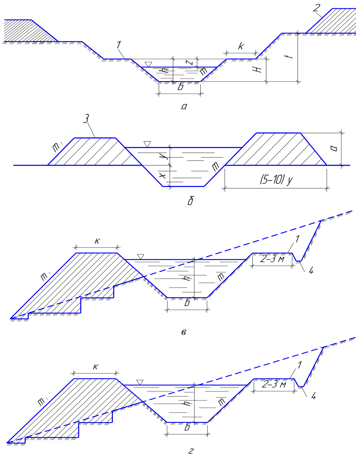
Рисунок 3.19 – Конструкции каналов
