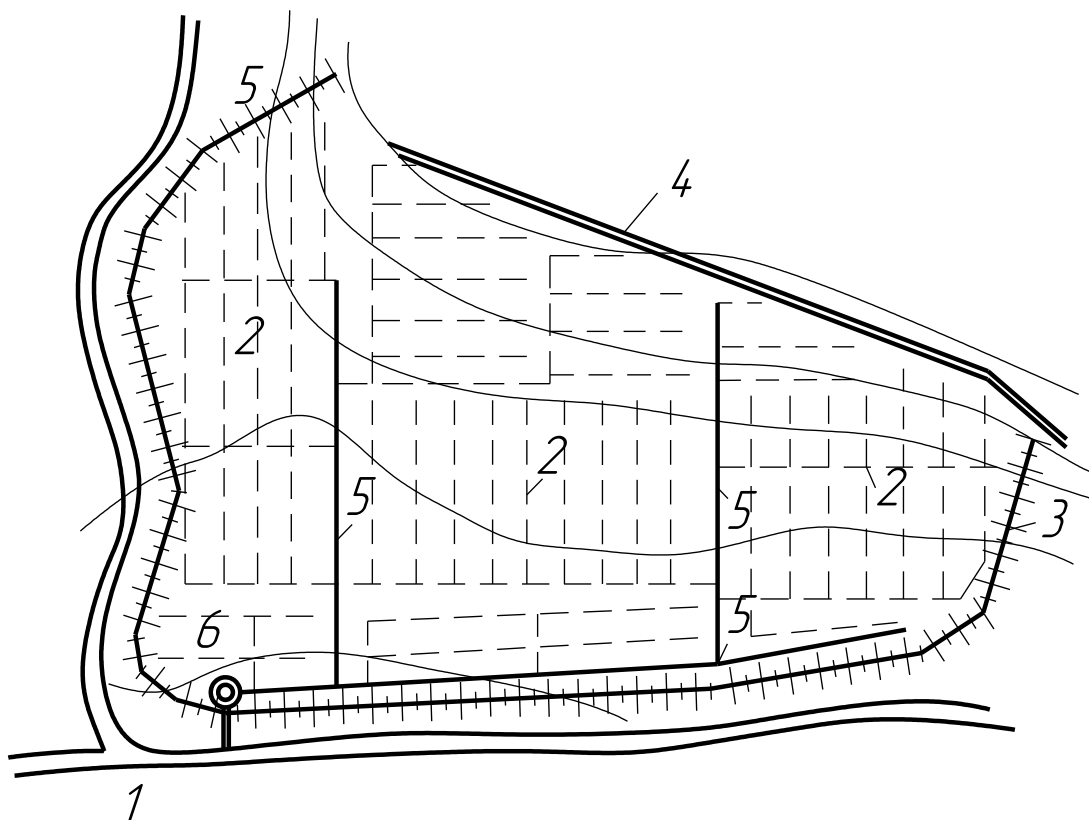
Рисунок 2.17 – Пolderная система осушения
