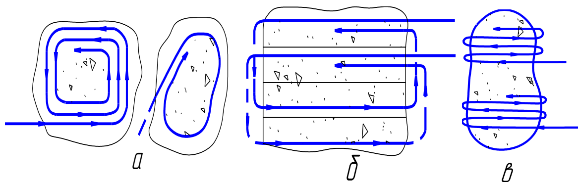
Рисунок 2.21 – Схемы работы кустореза а – спиральная; б – загонная; в – челночная
