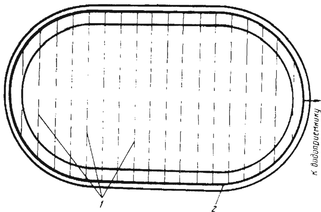
Рис. 54. Схема дренажирования стадиона: 1- дрены-осушители; 2- коллектор
