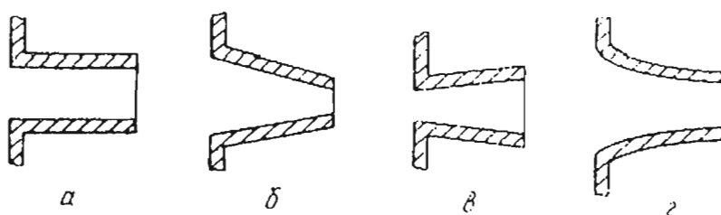
Рис. 8. Типы насадков
