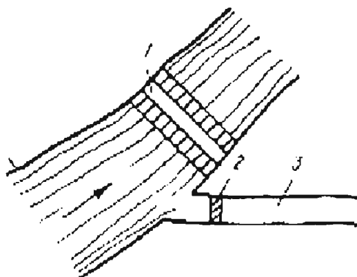
Рис. 81. Схема плотинного водозабора:
