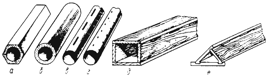
Рис. 46. Типы дренажных труб: а, б — гончарные; в, г — пластмассовые; д, е — деревянные
