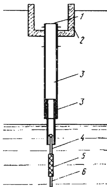
Рис. 72. Трубчатый колодец:
