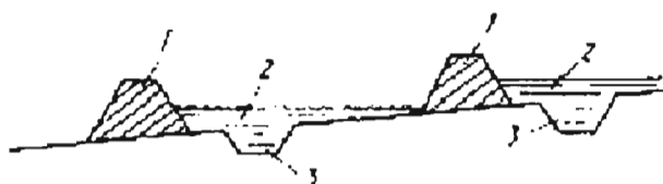
Рис. 95. Схема размещения лиманных дамб:
