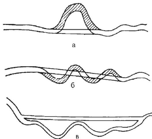
Рис. 57. Регулирование водоприемников: а- частичное спрямление русла; б- решительное спрямление русла; в- разгрузка реки водоприемника
