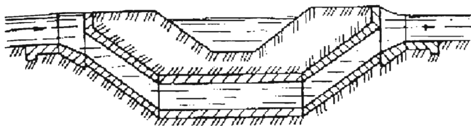
Рис. 84. Дюкер
