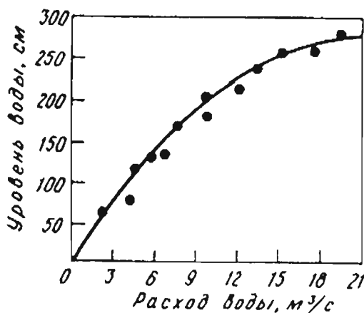
Рис. 19. Кривая расходов
