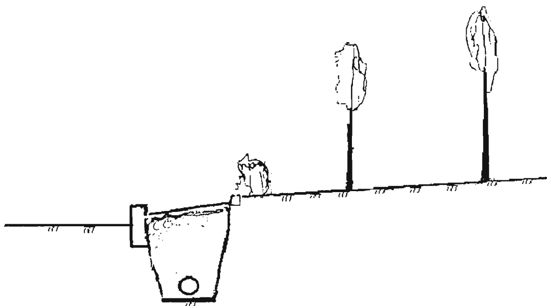
Рис. 55. Защитная зона с дренажем вдоль бульвара
