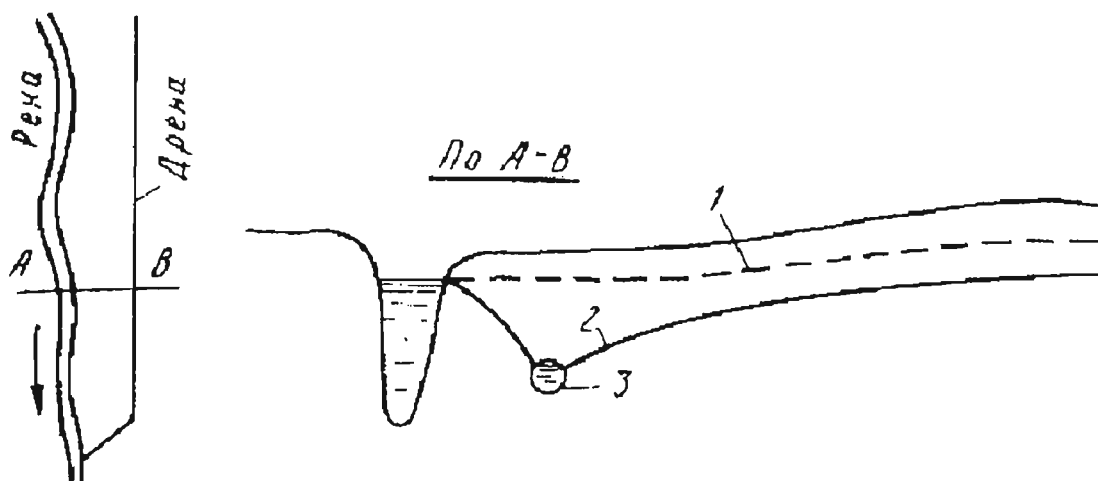
Рис. 56. Береговой дренаж:
