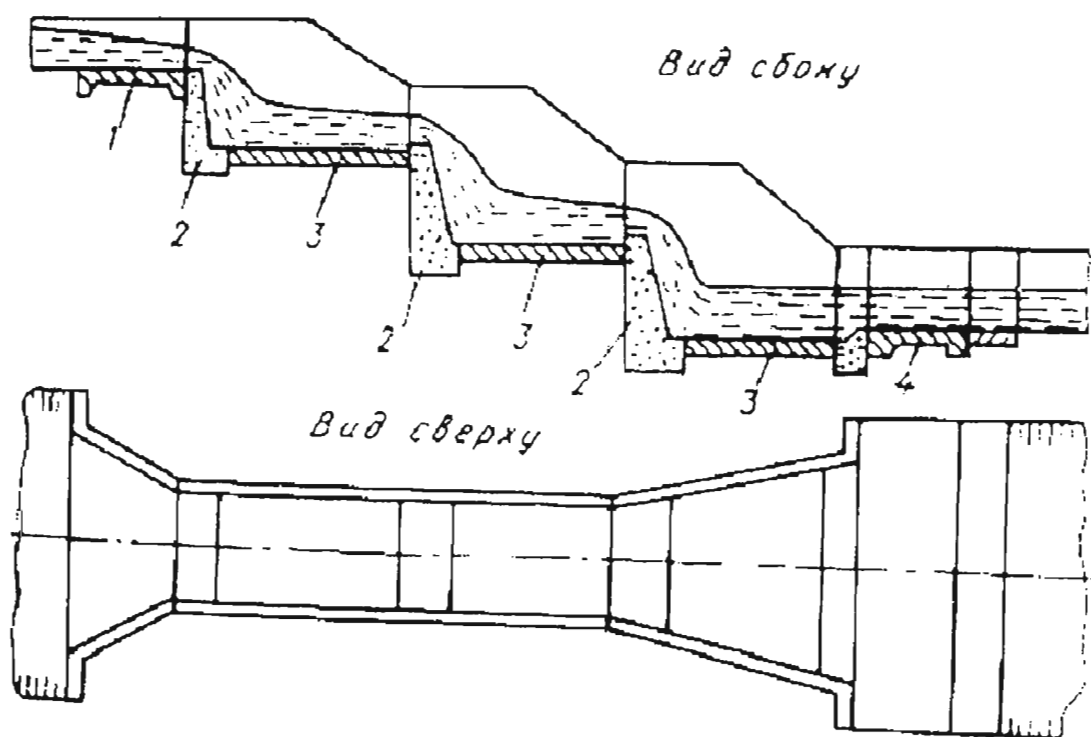
Рис. 43. Ступенчатый бетонный перепад: 1- понур; 2- стенки падения; 3- водобойная плита; 4- выход
