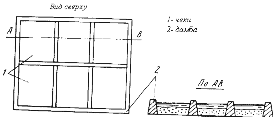
Рис. 50. Схема кольматажа
