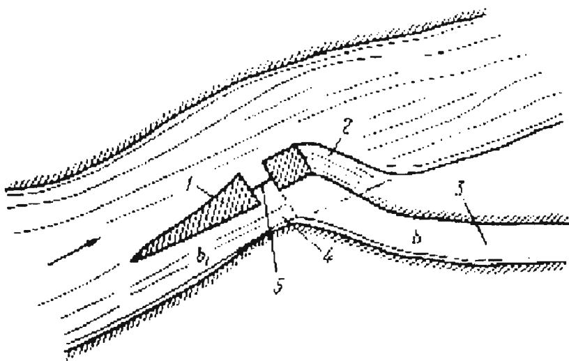
Рис. 80. Схема бесплотинного водозабора на реке:
