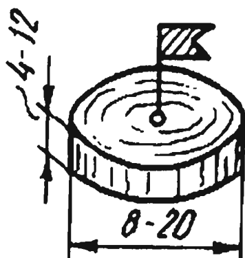
Рис. 16. Поплавков
