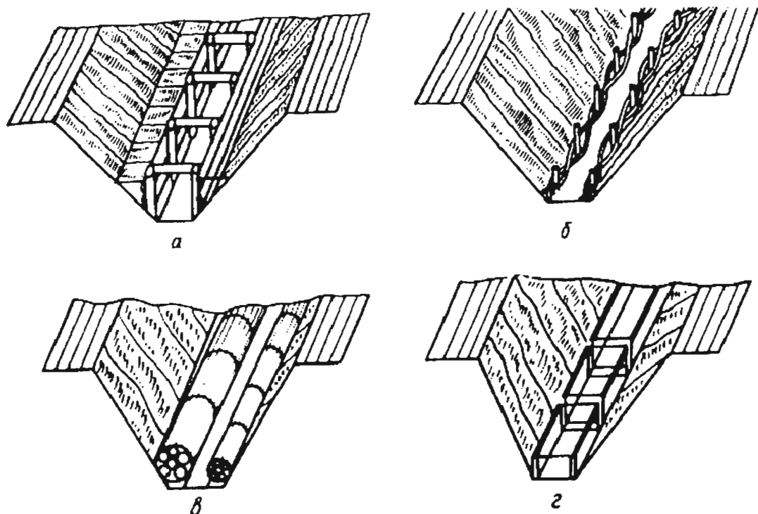
Рис. 38. Крепление откосов:
