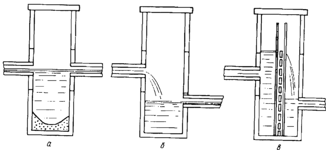
Рис. 49. Типы смотровых колодцев
