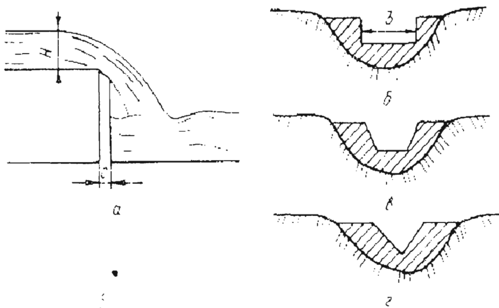
Рис. 9. Водосливы:
