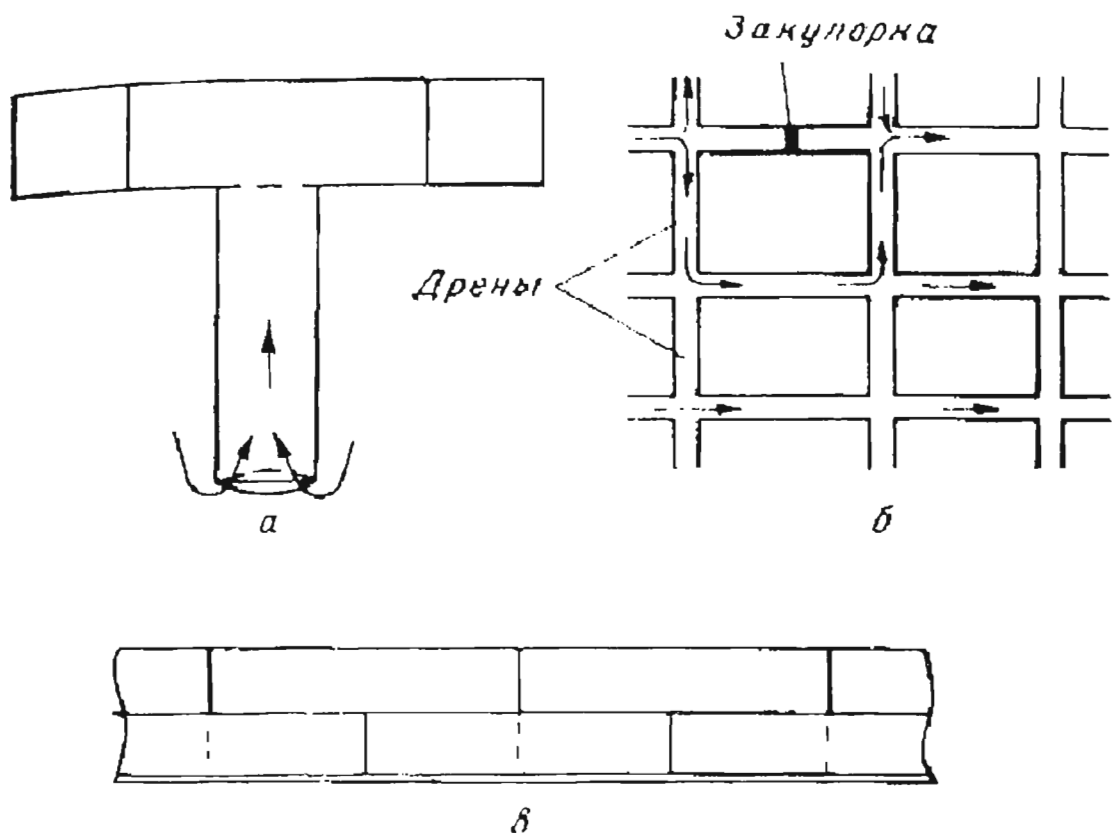
Рис.53. Схемы дренажирования садов и парков: а- дренаж Реролле; б- перекрестный дренаж; в- двойной дренаж
