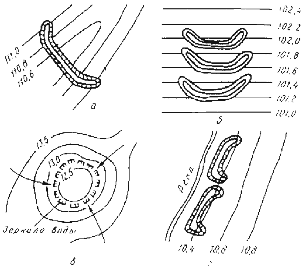
Рис. 96. Виды лиманов:
