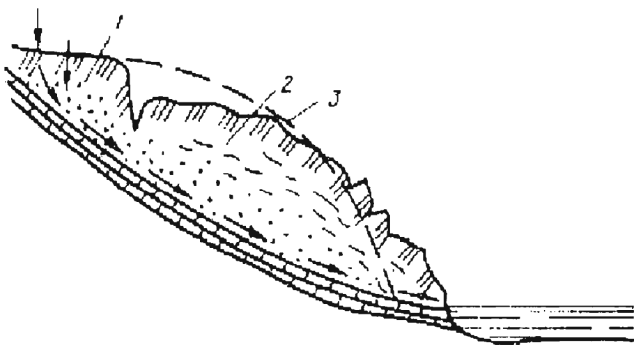
Рис. 105. Оползень:
