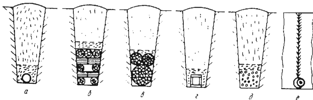
Рис. 45. Виды дренажа:
