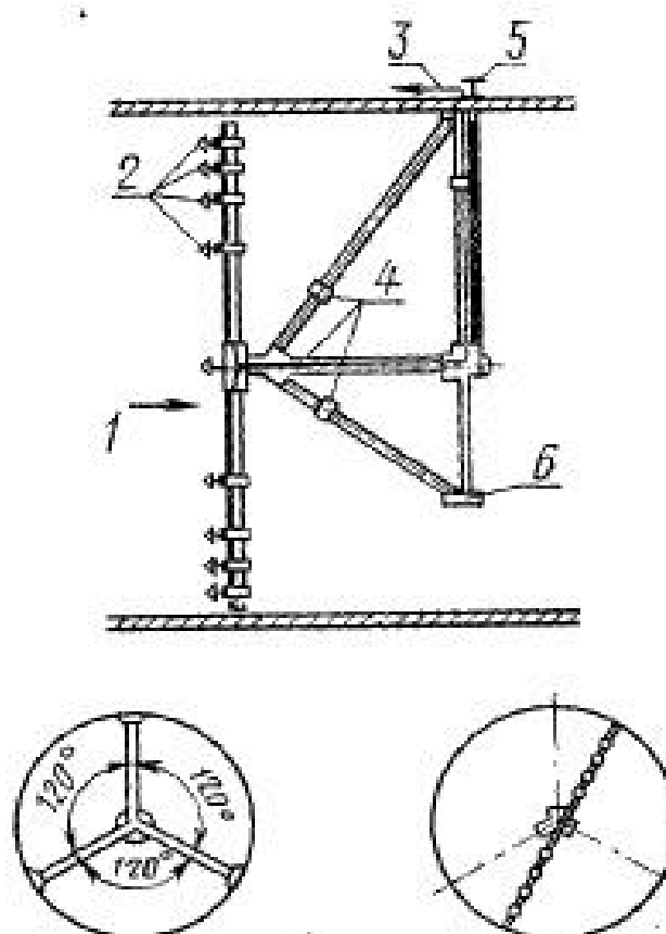
1—направление течения; 2—гидрометрические вертушки; 3—линия к хронографу; 4—держатель треноги; 5—привод штанги; 6—опорная пята треноги
