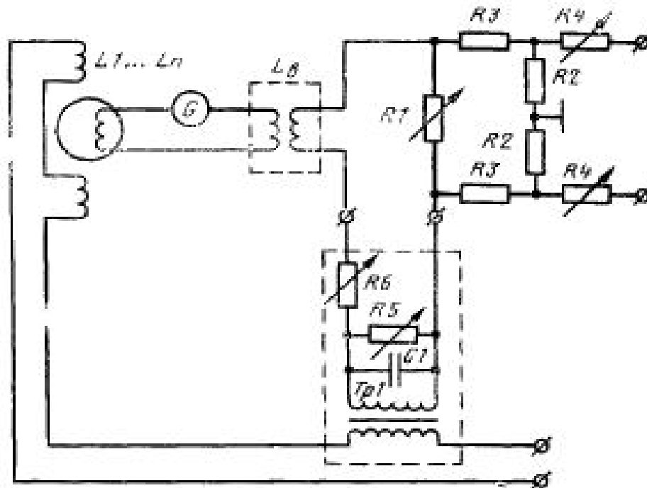
R — регулировочное сопротивление; G — емкость; Tr1 — трансформатор; L1 \dots Ln — набор регулировочных индуктивностей
