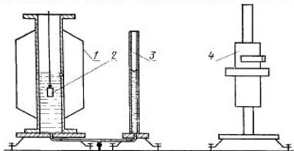
1 — преобразователь расхода, 2 — груз, 3 — калиброванный стеклянный сосуд; 4 — катетометр
