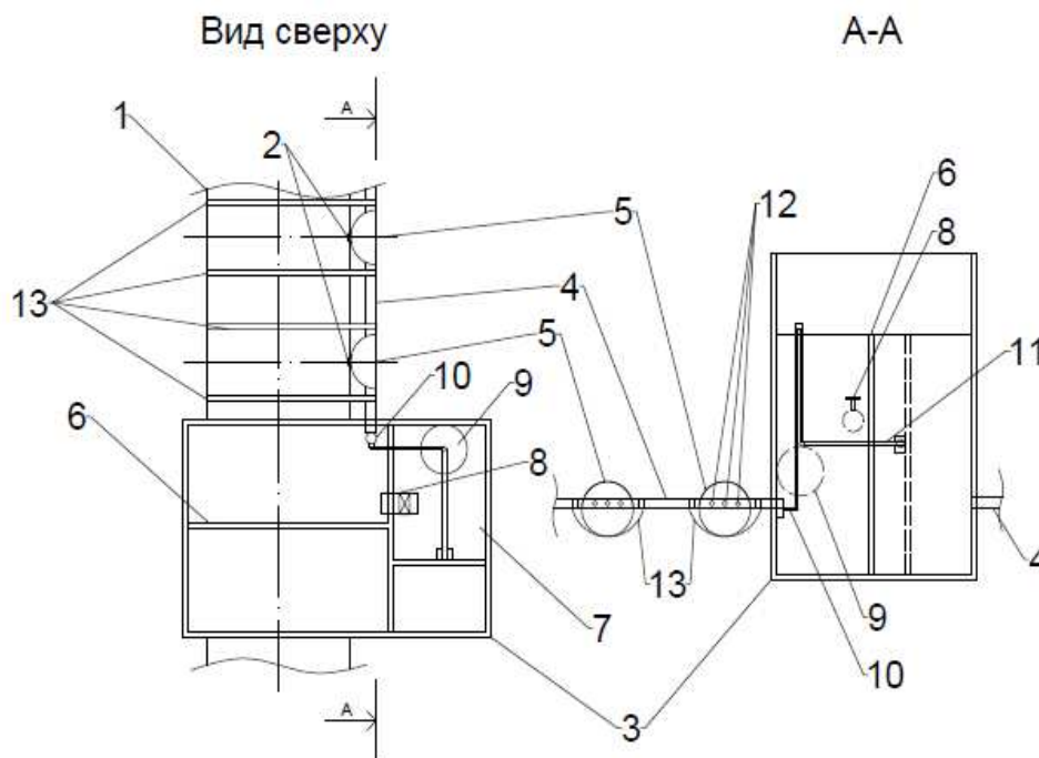
Рисунок 1 – Поливное звено:
