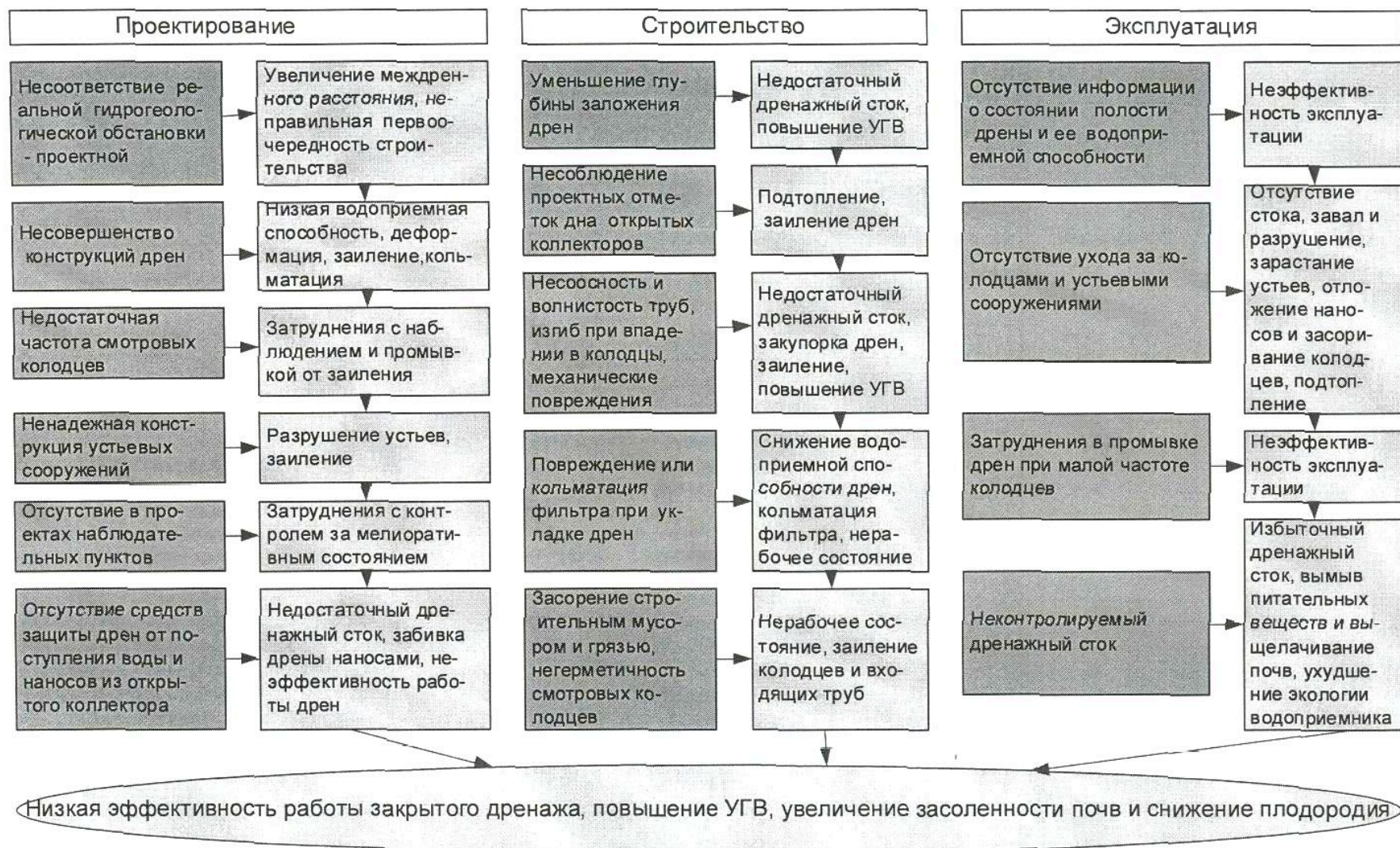
Рис. 1. Схема причинно-следственных связей, обуславливающих неудовлетворительную работу закрытого дренажа
