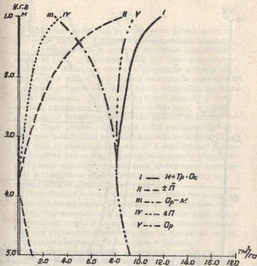
Рис. 1. Сравнительные зависимости оросительных норм, суммарного водопотребления и их элементов для Голодной степи при C_{\text{ср}} = 7 г/л
