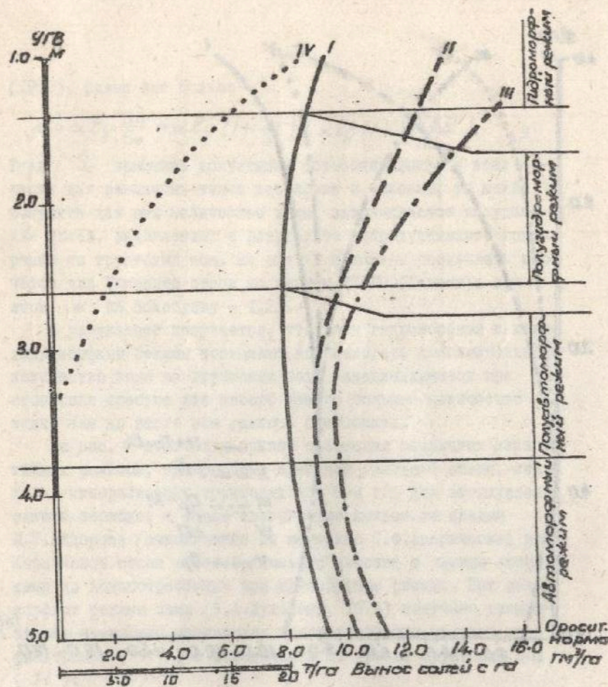
Рис. 2. Зависимость оросительных норм от различных мелиоративных режимов и влияние их на загрязнение стока рек; I - оросительные нормы для Голодной степи; II - то же для Каршинской степи (И.П. Айдаров); III - то же для Кашибадамского массива (И.П. Айдаров, Э.К. Каримов); IV - вынос солей с га по Голодной степи.
