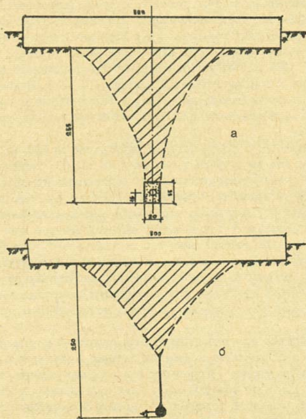
Рис. I. Пластмассовая дренажная труба \varnothing 75 мм, \varnothing 63 мм с песчано-гравийным фильтром (а); та же труба с напроновым фильтром (б).
