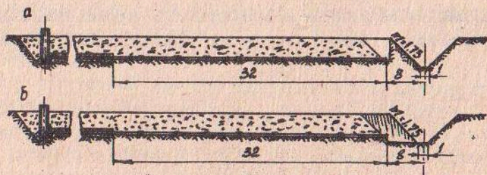
Рис. I. Технология поэтапного строительства закрытых горизонтальных дрен (размеры в м): а — I этап; б — 2 этап.
