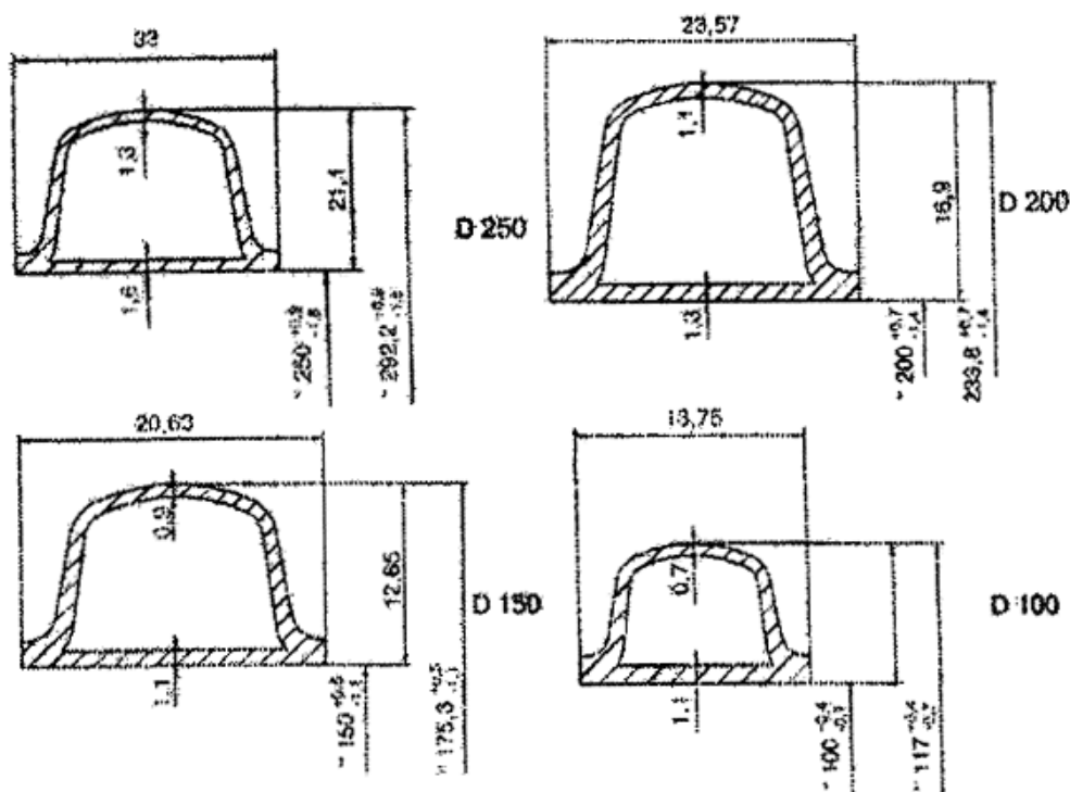
Рис. 2. Полые гофры двухслойных дренажных труб
