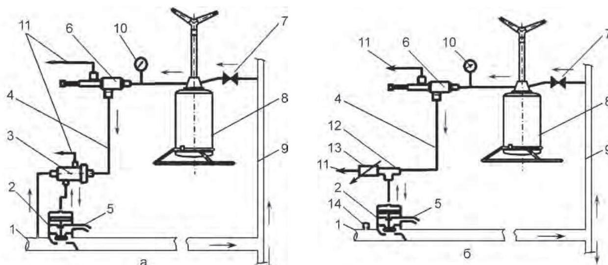
Рис. 6.6. Схемы управляющего узла – генератора командных сигналов для КСИД-1: а – с уклонами более 0,05; б – с уклонами до 0,05; 1 – распределительный трубопровод; 2 – клапан гидроуправляемый; 3 – клапан-распределитель; 4 – канал управления; 5 – сбросная труба; 6 – реле давления; 7 – кран дросселирующий; 8 – командный импульсный дождеватель; 9 – поливной трубопровод; 10 – манометр; 11 – слив в атмосферу; 12 – тройник 1/2"; 13 – дроссель; 14 – заглушка 1/2"
