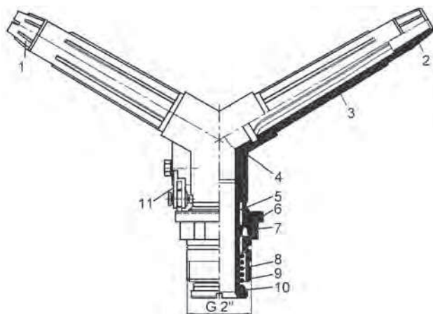
Рис. 6.3. Среднеструйный дождевальный аппарат: 1, 2 – сопла; 3 – ствол; 4 – корпус; 5 – втулка; 6 – колесо храповое; 7 – манжета; 8 – пружина; 9 – втулка в сборе; 10 – шайба; 11 – механизм шаговый храповой
