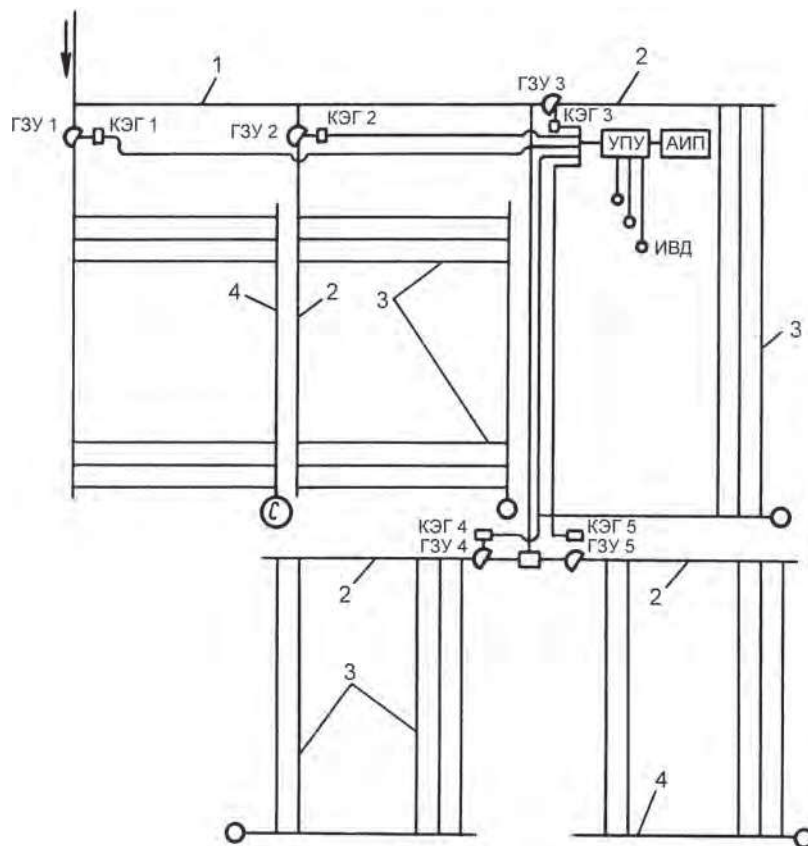
Рис. 10.3. Схема оросительно-увлажнительной сети и электрических линий управления: 1, 2 – распределительный и оросительный трубопроводы; 3 – полиэтиленовые увлажнители; 4 – водосборно-сбросной трубопровод; ГЗУ – гидроуправляемое запорное устройство; КЭГ – электрогидроуправляемый клапан; УПУ – устройство программного управления; ИВД – индикатор давления почвенной влаги; АИП – аккумуляторный источник питания
