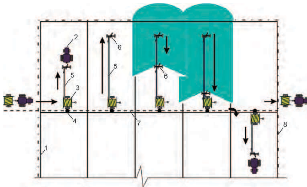
Рис. 4.2. Технологическая схема полива ШДБТ: 1 – граница орошаемого участка; 2 – трактор; 3 – шланговый дождеватель; 4 – гидрант оросительной сети; 5 – полиэтиленовый шланг; 6 – дождевальная консоль; 7 – оросительная сеть; 8 – грунтовые дороги
