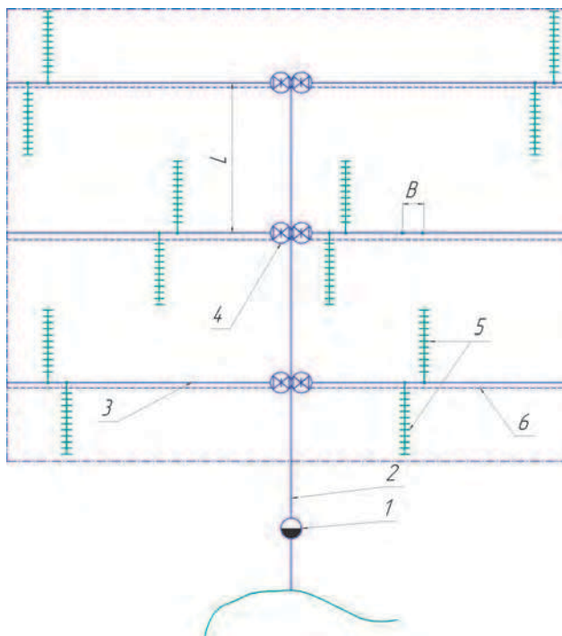
Рис. 3.33. Схема оросительной системы с колесными дождевателями: 1 – насосная станция; 2 – магистральный трубопровод; 3 – распределительный трубопровод с гидрантами; 4 – распределительный колодец с задвижками; 5 – поливные крылья колесного дождевателя; 6 – эксплуатационные дороги; 7 – граница орошаемой площади; L – расстояние между оросителями; B – расстояние между гидрантами
