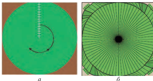
Рис. 3.6. Схема движения ЭДМ: а – классическая с поливом в движении по кругу; б – с использованием углового плеча на классической схеме движения
