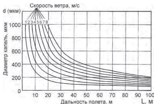
Рис. 6.15. Зависимость дальности полета капли от ее диаметра и скорости ветра (по данным А.М. Шарко, М.М. Османова, 1986)
