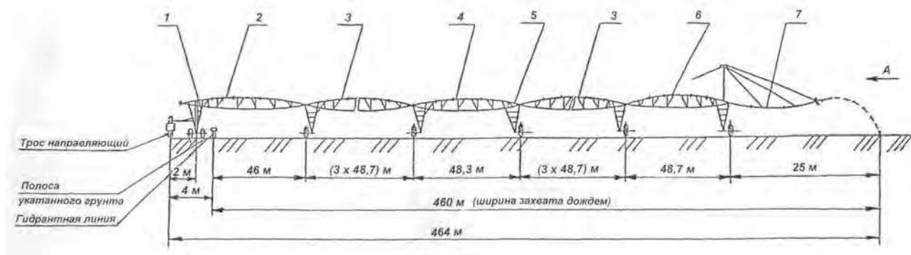
Рис. 3.11. Схема общего вида расположения основных элементов дождевальной машины «Ладога»: 1 – главная тележка; 2 – головная ферма; 3, 4 – фермы; 5 – опорная тележка; 6 – предконсольная ферма; 7 – консоль
