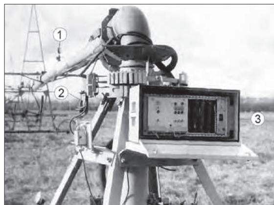
Рис. 3.29. Устройство локальной системы управления на неподвижной опоре ДМ «Фрегат»: 1 – датчик давления (ЭКМ); 2 – датчик начального положения машины; 3 – шкаф управления ЛСАУ
