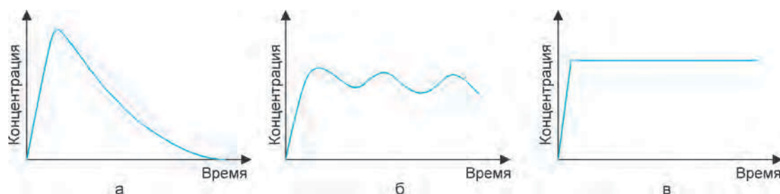
Рис. 8.9. Процесс поддержания концентрации раствора удобрений в оросительной воде при введении его через удобрительную емкость (а), насос-инжектор (б) и порционный насос-дозатор типа «Дозатрон» (в)
