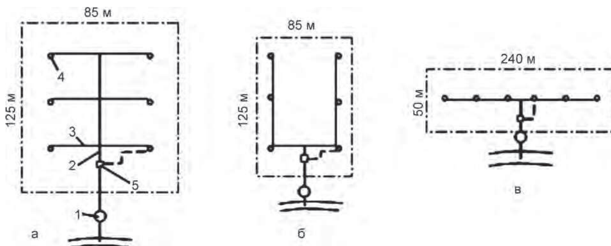
Рис. 6.5. Варианты схем расположения сети комплекта КСИД-1: а, б, в – возможные схемы трубопроводной сети; 1 – насосный агрегат; 2 – распределительный трубопровод; 3 – поливные трубопроводы; 4 – импульсный дождеватель; 5 – управляющий узел (генератор командных сигналов)
