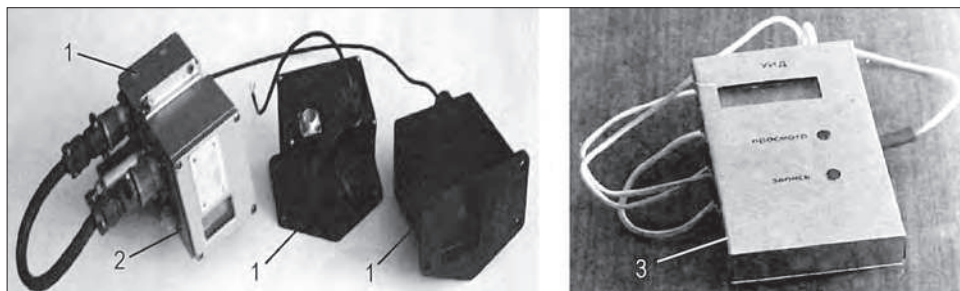
Рис. 1.12. Конструкция микроконтроллерного комплекса измерения и регистрации:
