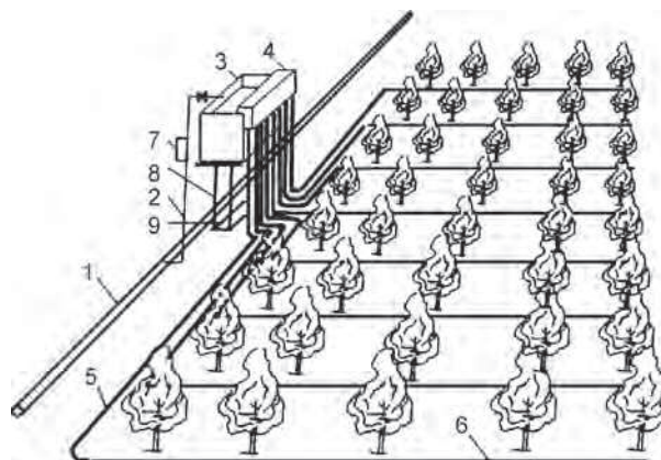
Рис. 8.10. Принципиальная схема модуля мелкоструйчатого импульсно-локального орошения садов:
