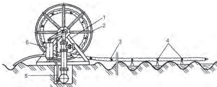
Рис. 9.3. Конструктивная схема поливного шлангового устройства (АШУ): 1 – рама; 2 – барабан; 3 – шланг; 4 – водовыпуск; 5 – линия управления от командного генератора; 6 – гидравлический привод барабана
