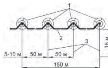
Рис. 9.13. Схема передвижного поливного комплекта ППК-25:
