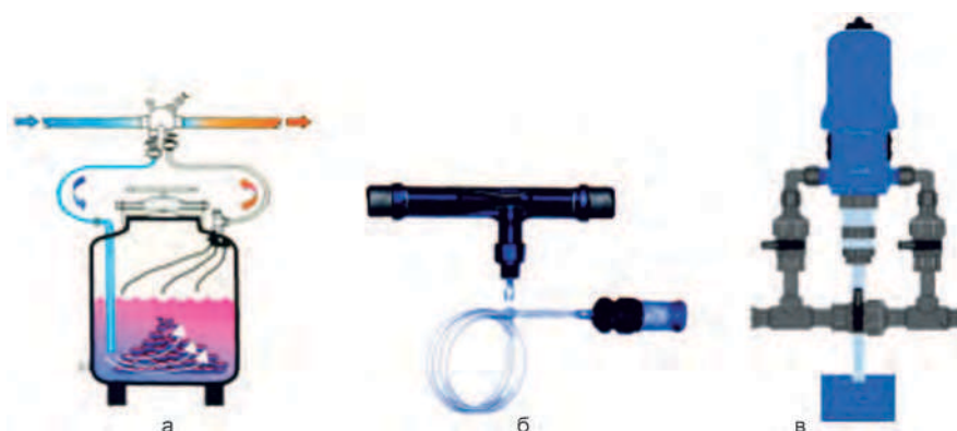
Рис. 8.8. Типы устройств для ввода растворов удобрений в поливную воду: а – емкость для растворимых удобрений; б – инжекторный насос «Вентури»; в – насос-дозатор «Дозатрон»
