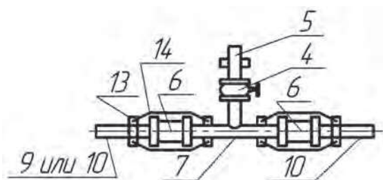
Узел подсоединения тройника
