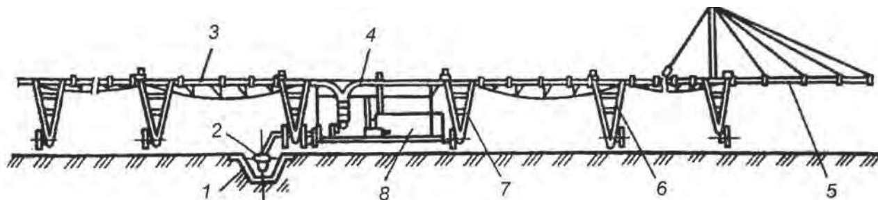
Рис. 3.16. Схема многоопорной самоходной машины типа «Кубань-Л»: 1 – канал; 2 – плавающий водозаборный клапан; 3, 4, 5 – соответственно промежуточная, центральная и консольная фермы; 6, 7 – промежуточная и центральная тележки; 8 – насосно-энергетическая установка (двигатель-насос-генератор)
