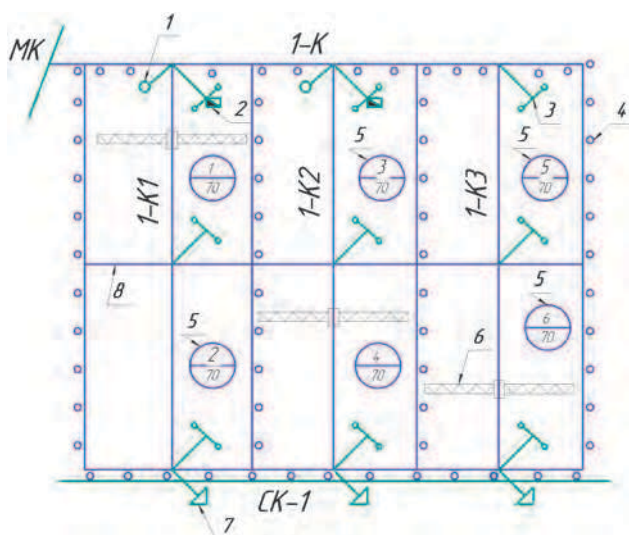
Рис. 3.17. Оросительная сеть на шестипольном севооборотном участке при поливе ЭДМФ «Кубань-Л»: 1 – водовыпуск; 2 – вододеливатель; 3 – трубчатый переезд; 4 – лесополосы; 1-6 – № поля и площадь брутто, га; 5 – ЭДМФ «Кубань-Л»; 7 – концевой сброс; 8 – дорога; МК – магистральный канал; 1-К – севооборотный канал; 1-К1-1-К3 – участковые каналы; СК-1 – сбросный канал
