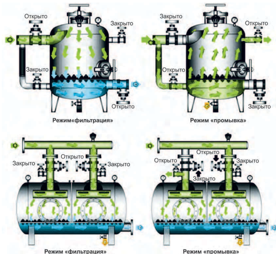
Рис. 8.6. Схемы промывки песчано-гравийной фильтростанции однокамерного и двухкамерного типов
