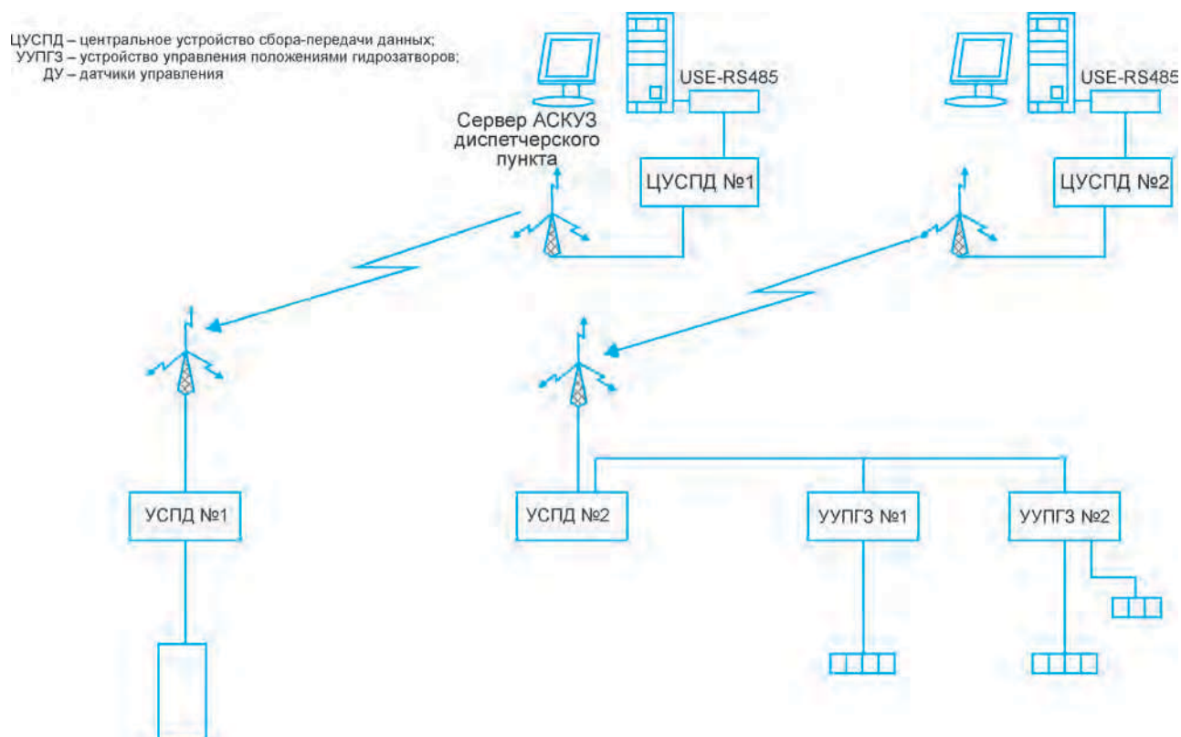
Рис. 12.2. Структурная схема управления гидрозадвижками, учета расхода электроэнергии и подачи воды
