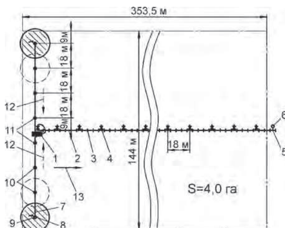
Рис. 4.5. Схема полива участка шланговым дождевателем с комплектом разборного трубопровода \varnothing 75 мм: 1 – шланговый дождеватель; 2 – полиэтиленовая труба, l = 6 м, \varnothing 75 мм; 3 – муфта \varnothing 75 мм; 4 – тройник с вентилем Ду 65; 5 – входной патрубок; 6 – манометр; 7 – трубопровод дождевателя; 8 – дождевальный аппарат (Д.А.) на опоре; 9, 10, 11 – позиции Д.А. при поливе; 12 – направление перемещения аппарата; 13 – направление перемещения шлангового дождевателя вдоль трубопровода
