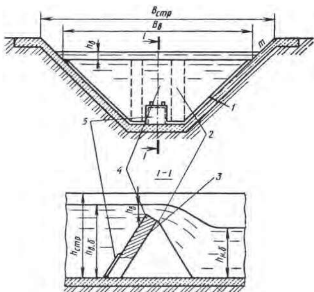
Рис. 3.18. Схема стационарной перемычки на каналах-оросителях для ЭДМФ «Кубань-Л» на уклонах до 0,003: 1 – цементный раствор; 2 – упорный блок; 3 – закладные детали (сварка); 4 – блок-перемычка; 5 – затвор (заслонка) для очистки канала
