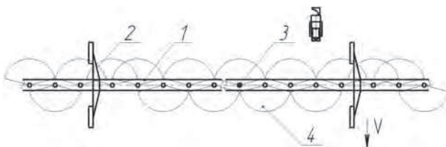
Рис. 3.21. Схема расстановки дождеобразующих устройств: 1 – трубопровод дождевальной машины; 2 – ходовая тележка; 3 – местоположение дождеобразующих устройств; 4 – формирование фронта дождя насадками; V – направление рабочего движения машины
