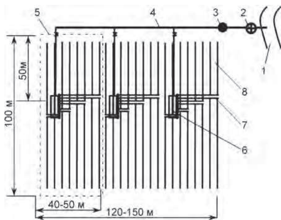
Рис. 8.11. Схема МИЛОС-М-1,0 на площади 1 га: 1 – водосточник; 2 – насосная станция; 3 – гидроподкормщик; 4 – напорный трубопровод; 5 – блок МИЛОС-М; 6 – накопительно-распределительный узел; 7 – распределительный трубопровод; 8 – поливной трубопровод
