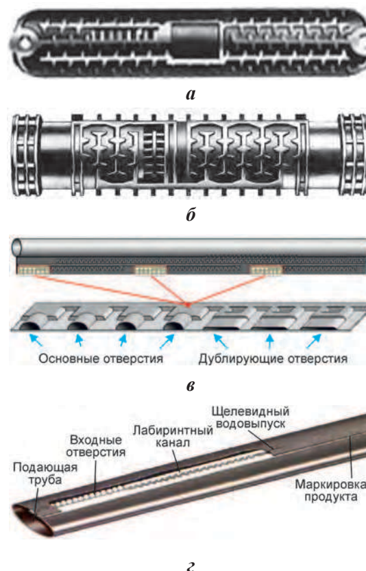
Рис. 8.2. Типы встраиваемых капельных водовыпусков: а – плоский эмиттер; б – цилиндрический эмиттер; в – щелевые «мягкие» водовыпуски
