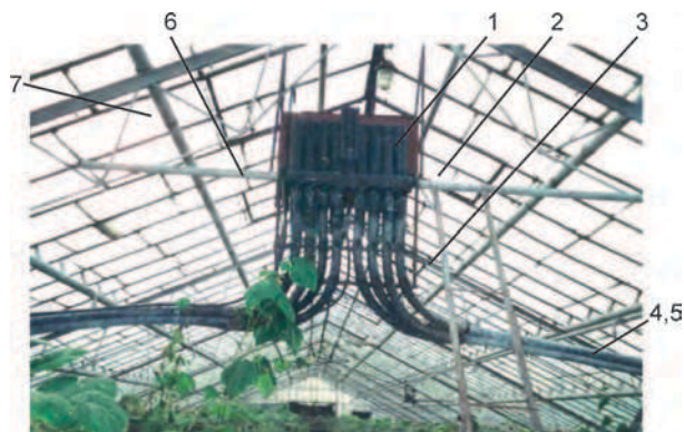
Рис. 8.14. Узел автоматизированного распределения водоподдачи в ангарной теплице:
