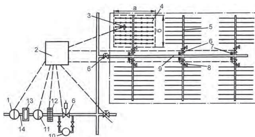
Рис. 8.1. Принципиальная схема системы капельного орошения:
