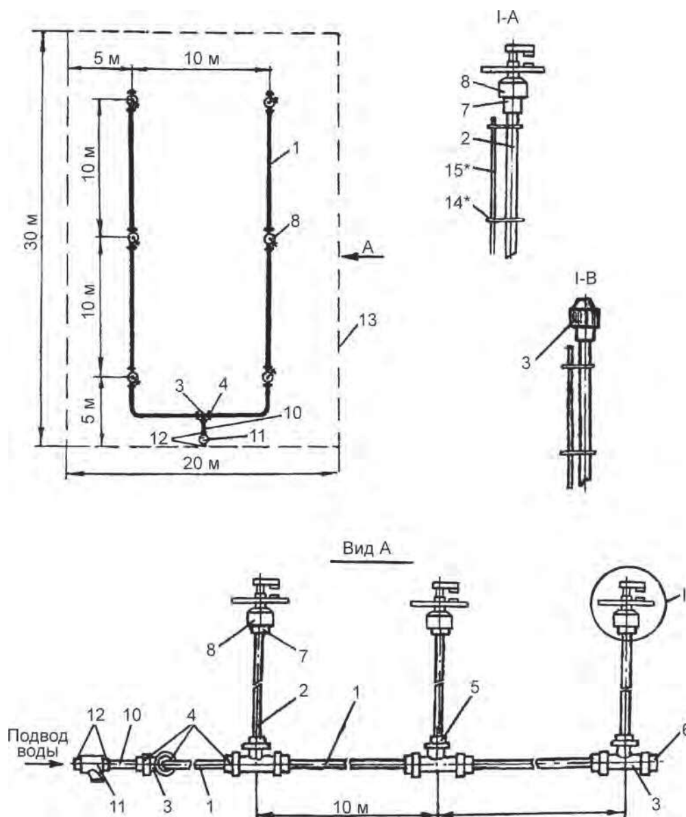
Рис. 7.12. Схема расположения оборудования: 1 – распределительный трубопровод ПНД-20; 2 – поливной трубопровод (стояк) ПВД-16; 3 – тройник; 4 – муфта М36х20; 5 – муфта М36х16; 6 – муфта-заглушка М36; 7 – штуцер G1/2"; 8 – малорасходный дождевальная аппарат (МДА); 9 – заглушка поливного трубопровода G1/2"; 10 – патрубок подсоединительный ПНД-20; 11 – фильтр ФММ-20; 12 – штуцер G3/4"; 13 – граница модульного участка; 14* – шпигат крепежный; 15* – стойка
