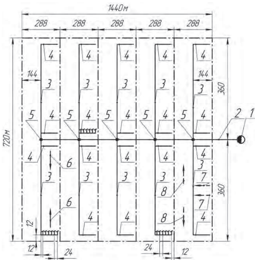
Рис. 5.20. Схема орошения участка десяти комплектами КИ-10 ( S=103,68 га, расход 100-110 л/с): 1 – насосная станция; 2 – магистральный трубопровод закрытой оросительной сети; 3 – распределительный трубопровод \Phi 110 мм, l = 348 м комплекта КИ-10; 4 – дождевальное крыло \Phi 75 мм, l = 132 м; 5 – гидрант с узлом подсоединения распределительных трубопроводов двух комплектов КИ-10; 6, 7, 8 – направления перемещения дождевальных крыльев
