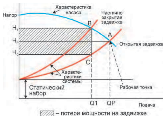
Рис.12.4. Характеристика насоса при регулировании подачи воды в оросительную систему задвижкой
