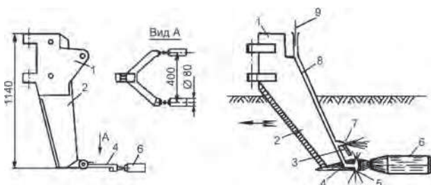
Рис. 10.8. Схемы рабочих органов кротователя КТД-0,45 для нарезки кротовых увлажнителей в грунтах при влажности не менее 21-30% и 15-21% от массы сухой почвы:
