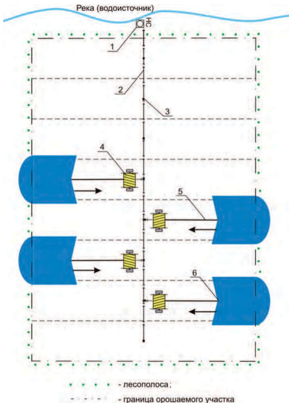
Рис. 4.14. Комплект мобильного ирригационного оборудования: 1 – передвижная насосная станция; 2 – быстросборный трубопровод; 3 – гидрант с задвижкой; 4 – ШДБТ; 5 – ПЭТ шланг; 6 – дождевальная аппаратура на штативе
