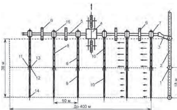
Рис. 9.14. Трубопровод колесный поливной ТКП-ПР:
