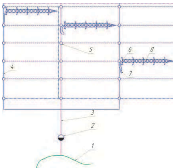
Рис. 3.14. Схема оросительной системы с дождевальной шланговой машиной «Ладога»:
