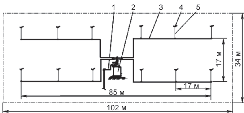
Рис. 6.8. Принципиальная схема комплекта КСИД-Р: 1 – подводящий трубопровод; 2 – пневмогидроаккумулятор импульсный; 3 – поливной трубопровод; 4 – дождевательный аппарат; 5 – стойка
