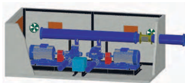
Рис.12.6. Общий вид насосной установки типа «Волга» на базе насосов типа Д
