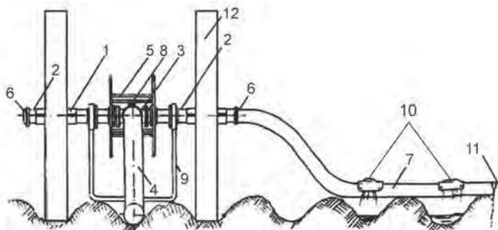
Рис 9.12. Унифицированная тележка передвижного поливного комплекта ППК-25:
