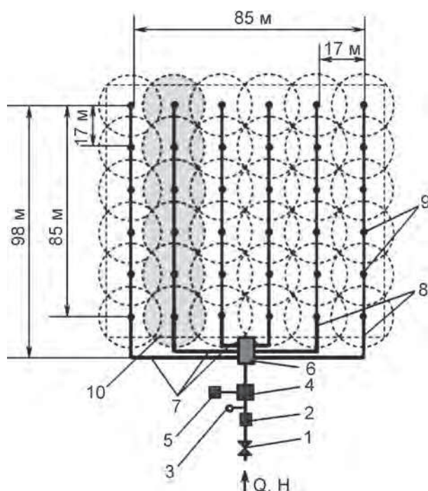
Рис. 6.12. Принципиальная схема сети комплекта КИД-1: 1 – входной кран; 2 – фильтр; 3 – манометр; 4 – электромагнитный клапан; 5 – контроллер; 6 – распределительный клапан; 7 – распределительные трубопроводы; 8 – поливные трубопроводы; 9 – стояк с дождевальным аппаратом; 10 – зона полива
