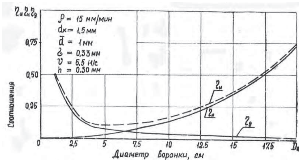
Рис. 1.3. Зависимости раздробленных и «налагаемых» капель от диаметра воронки: \eta_o — раздробленных; \eta_n — «налагаемых»; \eta_u — суммарных
