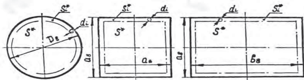
Рис. 1.2. Форма приемной площади прибора
