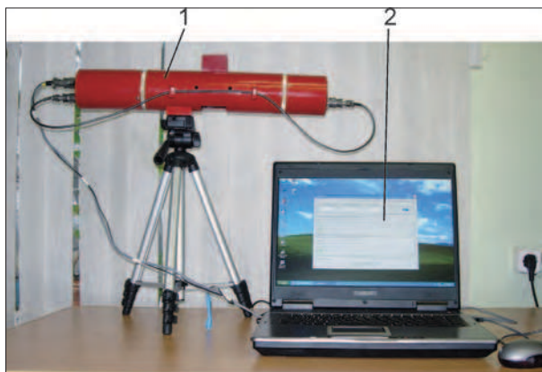
Рис. 1.6. Система «Спектр-4М»: 1 – фотоэлектрический датчик ФД-1М; 2 – переносной компьютер
