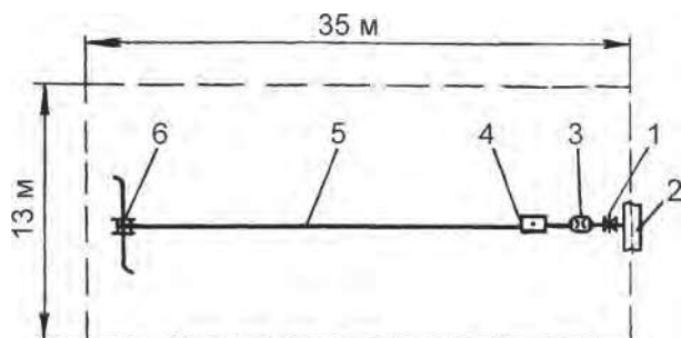
Рис. 7.6. Схема расположения оборудования на позиции: 1 – вентиль; 2 – трубопровод подводящий; 3 – разъем; 4 – якорь и отсекающий; 5 – водопроводящий шланг; 6 – дождеватель шланговый
