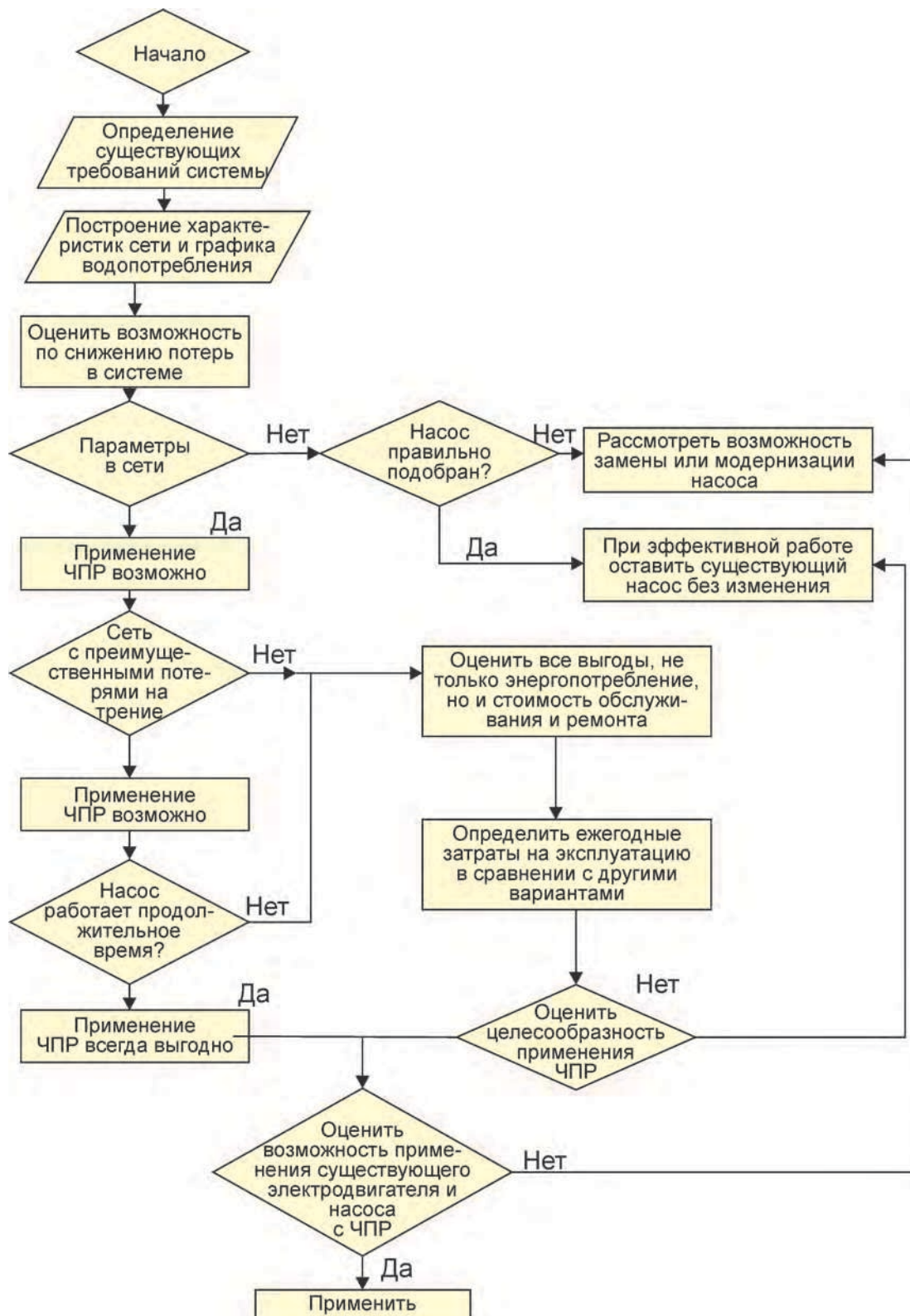
Рис.12.5. Блок-схема принятия решения о применении частотного привода
