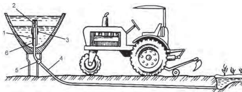
Рис. 9.2. Автоматизированный поливной лоток (АПЛ): 1 – сифонный водовыпуск; 2, 5 – втулки для настройки водовыпуска на заданный расход и подсоединения шланга; 3 – поплавок; 4 – полиэтиленовый шланг; 6 – стакан
