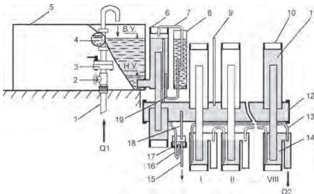
Рис. 8.15. Принципиальная гидравлическая схема сифонного узла автоматического распределения водоподдачи:
