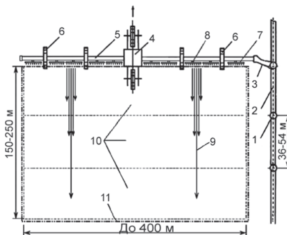
Рис. 9.16. Технологическая схема полива по бороздам по продольной схеме с применением колесного трубопровода ТКП-П (одно крыло):
