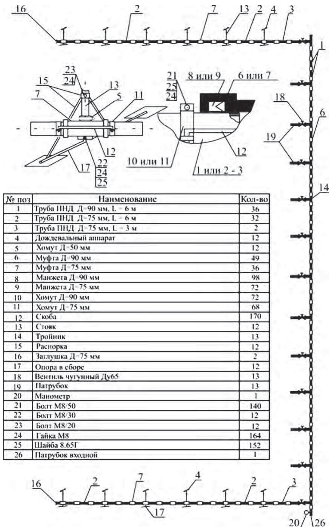
Рис. 5.2. Монтажная схема комплекта КИ-5
