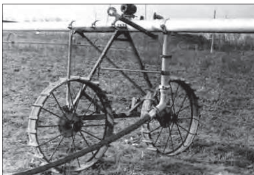
Рис. 9.11. Поливной шлейф для поверхностного полива на ДМ «Днепр»
