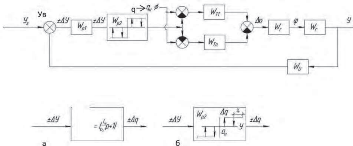
Рис. 3.30. Структурная схема системы управления фронтальной машины «Кубань-Л» с обратной связью: а – регулирующее звено по производной в обратной цепи W_o ; б – нелинейное форсирующее звено W_{p2} ; W_{p1} – линейное (пропорциональное) звено; W_p , W_r , W_c – динамические звенья опорной тележки, разворота и смещения машины соответственно; y_3 , y , y_o – заданное, текущее и возмущающее смещение машины; y_o – величина снижения отклонения машины от максимального; a_n – порог чувствительности регулятора; \phi – угол поворота машины
