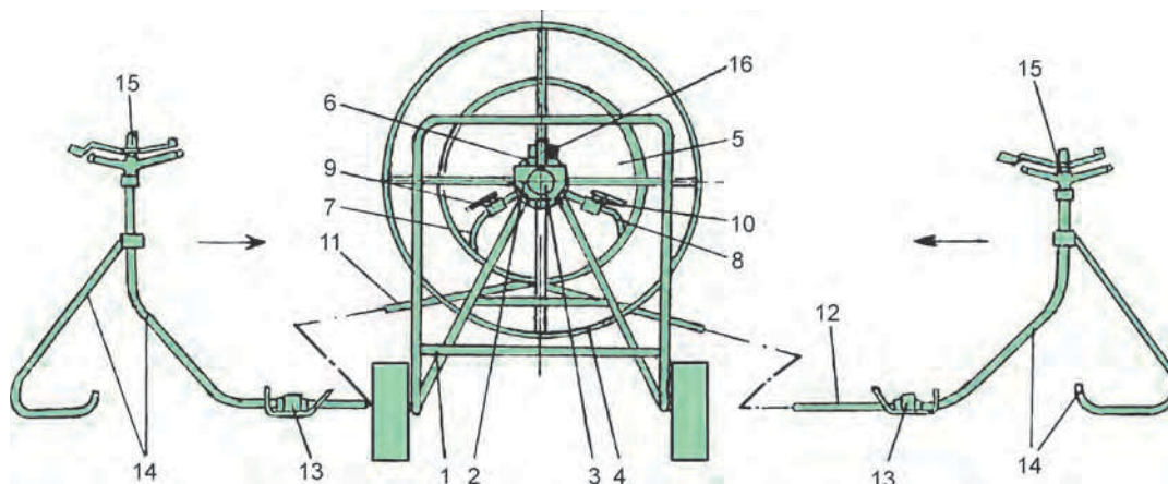
Рис. 4.4а. Шланговый дождеватель: 1 – рама; 2 – опора рамы; 3 – полый вал; 4 – катушка; 5 – барабан; 6 – внутренняя труба; 7,8 – отводы; 9,10 – краны; 11,12 – полиэтиленовые трубы \varnothing 32 мм, l = 50 м; 13 – муфта; 14 – опора; 15 – дождевательный аппарат; 16 – стопор
