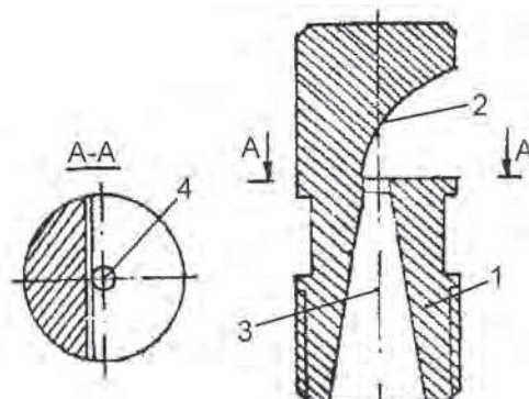
1 – корпус; 2 – цилиндрический дефлектор; 3 – проходной канал в форме конфузора
