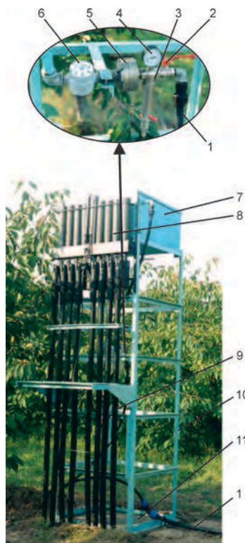
Рис. 8.13. Узел автоматизированного распределения водоподачи в саду: 1 – подводный трубопровод; 2 – кран; 3 – фильтр; 4 – манометр; 5 – стабилизатор расхода; 6 – счётчик воды; 7 – ёмкость; 8 – распределитель; 9 – распределительные трубопроводы; 10 – опора; 11 – опорная плита
