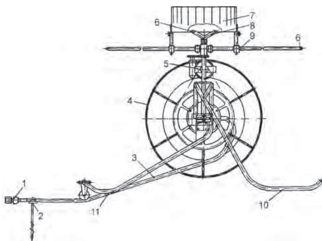
Рис. 7.5. Схема общего вида шлангового дождевателя ДШ-1: 1 – узел подсоединения; 2 – якорь; 3 – водопроводящий шланг; 4 – катушка; 5 – редуктор; 6 – сопла с рассекателями; 7 – корона; 8 – дождевальная аппаратура; 9 – сегнерово колесо; 10 – лыжи; 11 – опора с направляющим роликом
