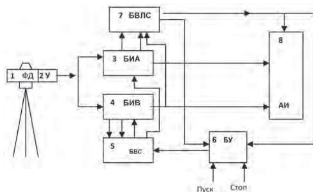
Рис. 1.7. Блок-схема ИИС «Спектр-4»
