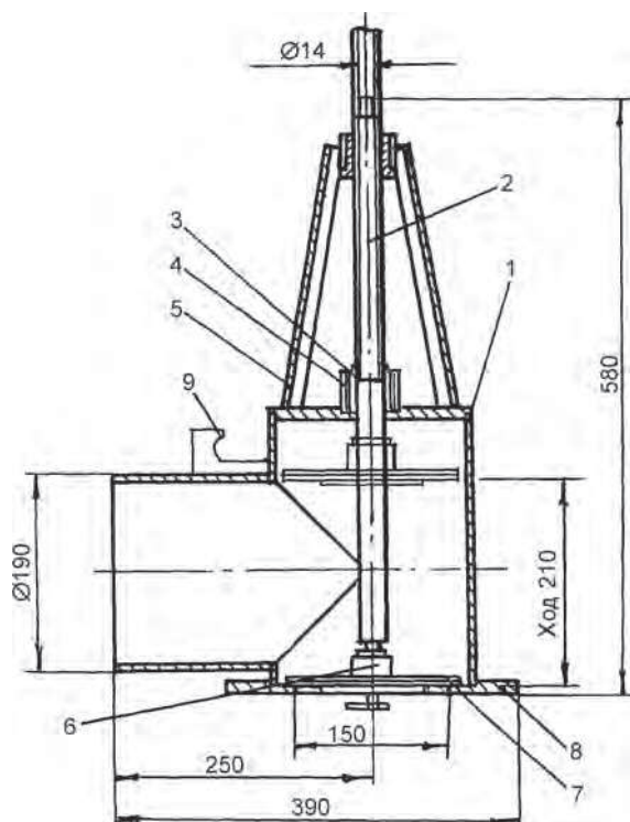
Гидрант ДМ ДДН-70
