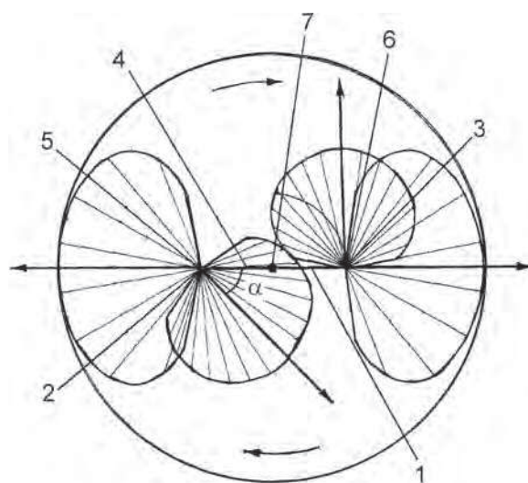
Рис. 7.3. Схема расположения насадок и формирования факелов дождя: 1, 4 – дождевальные крылья установки; 2, 3 – концевые горизонтальные насадки с соплами диаметром 5 мм; 5 – насадка с диаметром сопла 4 мм; 6 – насадка с диаметром сопла 3 мм; 7 – дождевальная установка (центр вращения); → – направления факелов насадок
