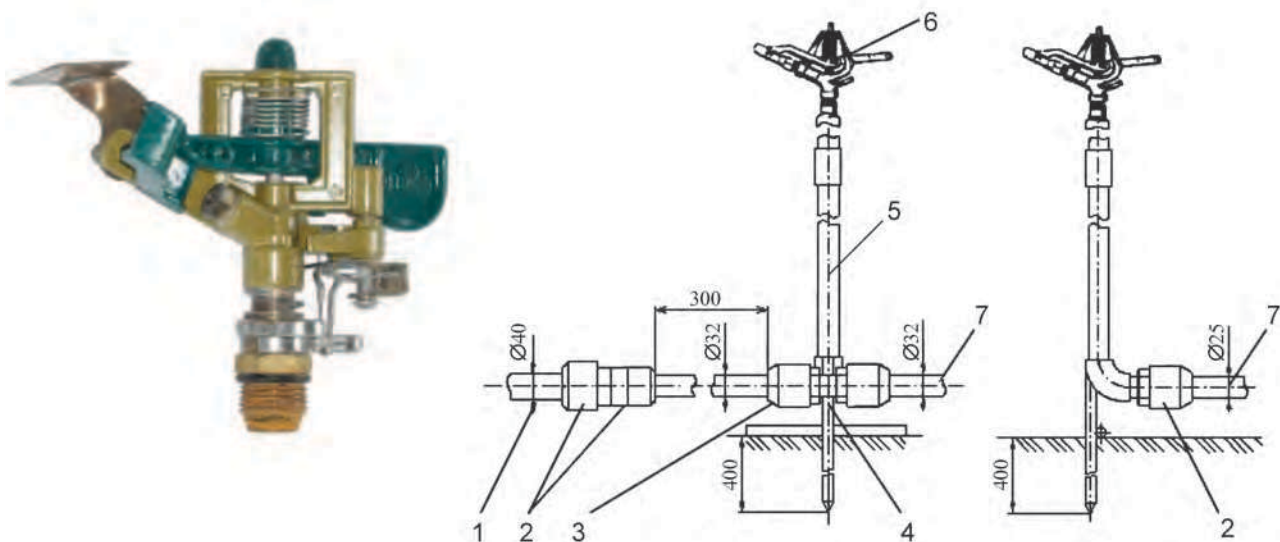
Рис. 6.9. Дождевальный аппарат «RACO» (Expert) 1/2" с соплом 3,5 мм: 1 – распределительный трубопровод; 2 – переходные муфты; 3 – тройник; 4 – основание; 5 – труба стояка; 6 – дождевальный аппарат; 7 – поливной трубопровод
