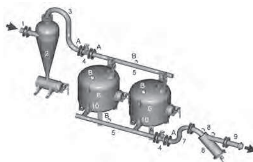
Рис. 8.7. Схема базовой комплектации фильтровальной станции:
