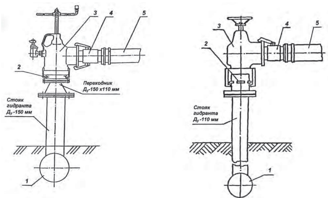
Рис. 3.13. Узлы подключения шланга к оросительной сети различного диаметра: 1 – трубопроводная оросительная сеть; 2 – запорное устройство; 3 – гидрант-колонка; 4 – наконечник для подсоединения к колонке; 5 – шланг
