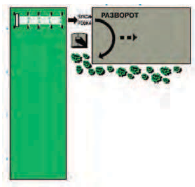
Рис. 3.4. Фронтально-перемещаемая схема движения ЭДМ: L – образная фронтальная схема движения ЭДМ, когда, завершив полив первой части орошаемого участка, машина производит разворот на 90° и продолжает полив второй части участка (рис. 3.5)
