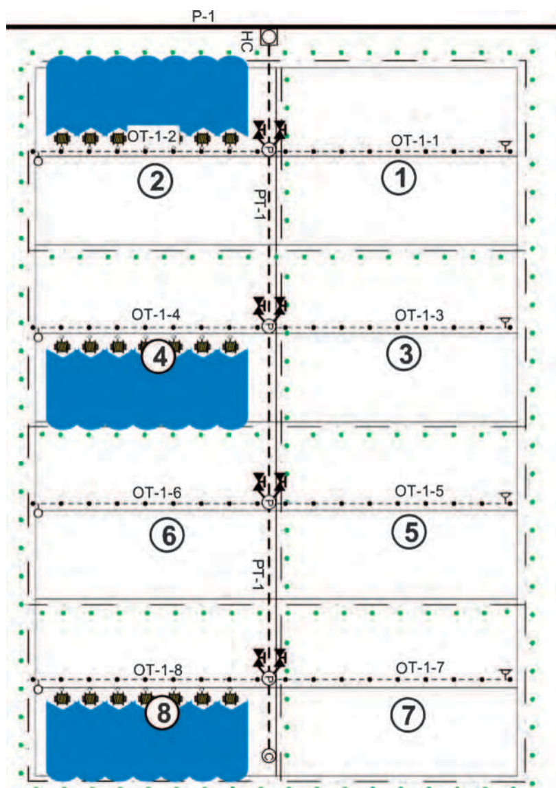
Рис. 4.13. Схема оросительной сети для полива шланговыми дождевателями барабанного типа
