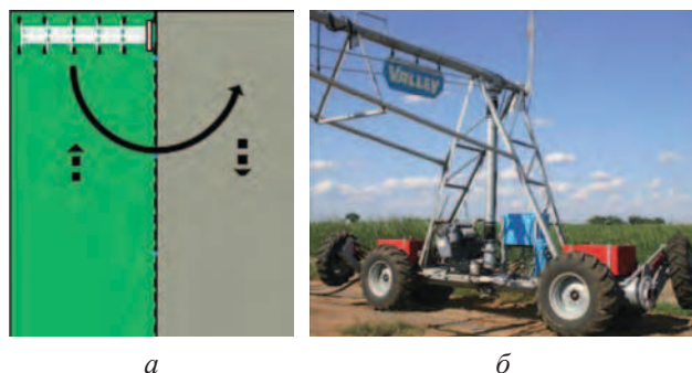
Рис. 3.3. а – фронтально-поворотная схема движения ЭДМ; б – 4-колесная поворотная опора-тележка для фронтально-поворотной схемы движения ЭДМ
