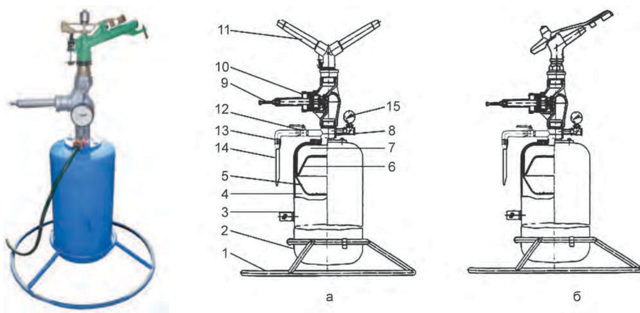
Рис. 6.7. Дождеватель импульсный автоколебательный АИД-1: а – с разгруженным дождевальным аппаратом; б – с коромысловым дождевальным аппаратом; 1 – опора; 2 – корпус водовоздушного бака; 3 – клапан воздушный; 4 – воздушная полость; 5 – перфорированный свод; 6 – эластичная мембрана; 7 – водяная полость; 8 – патрубок; 9 – болт регулировки давления срабатывания; 10 – запорный орган гидроуправляемый автоколебательный; 11 – дождевательный аппарат; 12 – кран непрерывной водоподачи; 13 – угольник переходный компрессионный; 14 – подводящий трубопровод; 15 – манометр
