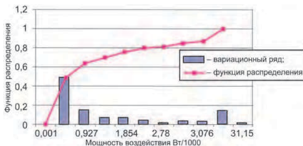
Рис. 1.11. Функция распределения мощности воздействия капель на почву
