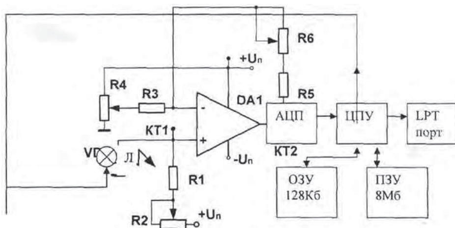
Рис. 1.5. Электронная схема фотопреобразователя и функциональная схема устройства сбора данных ФД-1: Л – лампа; VD1 – фотодиод; DA1 – усилитель; АЦП – аналого-цифровой преобразователь; ОЗУ, ПЗУ – оперативное и постоянное запоминающее устройство; ЦПУ – процессор
