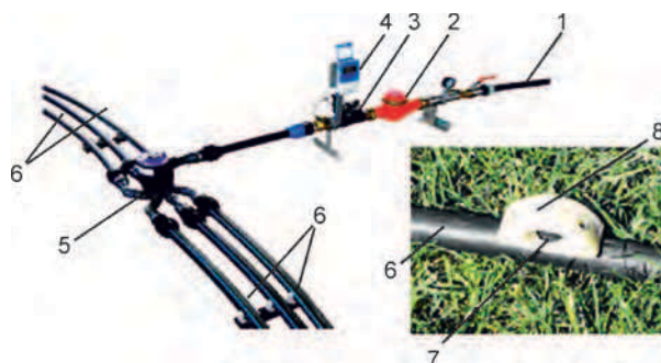
Рис. 9.6. Узел автоматического управления импульсного полива:
