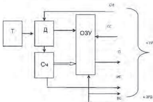
Рис. 1.13. Блок-схема МЦР-1
