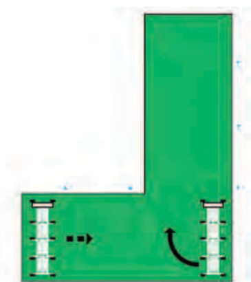
Рис. 3.5. L-образная фронтальная схема движения ЭДМ
