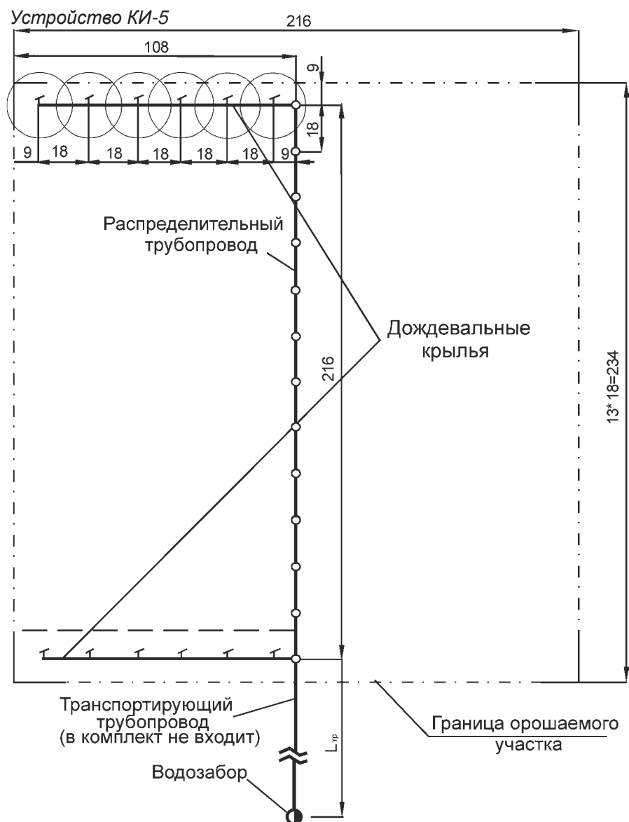
Рис. 5.1. Типовая схема монтажа комплекта КИ-5
