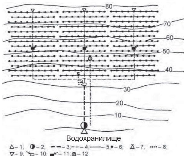
Рис. 6.1. Принципиальная схема системы синхронного импульсного дождевания: 1 – водозаборное сооружение; 2 – насосная станция; 3 – магистральный трубопровод; 4 – распределительный трубопровод; 5 – поливной трубопровод; 6 – импульсный дождеватель; 7 – датчик заполнения системы; 8 – управляющие линии; 9 – вантуз; 10 – генератор командных сигналов с дождевателем; 11 – усилитель командных сигналов; 12 – датчик необходимости полива
