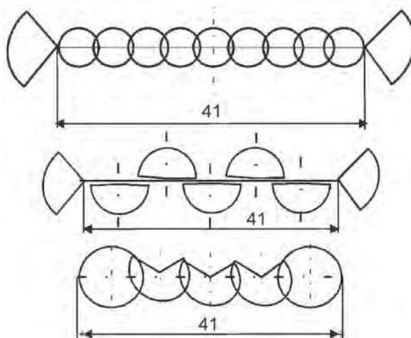
Рис. 4.12. Схемы расположения насадок и дождевальных аппаратов на ферменном водораспределителе
