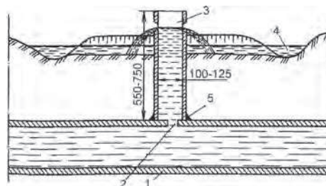
Рис. 9.1. Закрытый автоматизированный поливной трубопровод (АПТ) для полива садов и виноградников:
