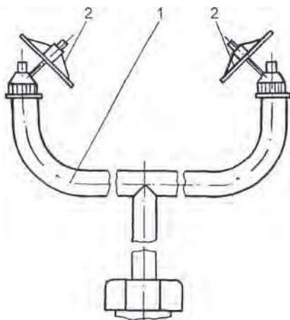
Рис. 7.10. Установка МДА: 1 – дополнительный трубопровод; 2 – малорасходный дождевальный аппарат (МДА)
