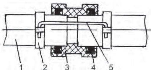
Рис. 5.17. Соединение труб: 1 – полиэтиленовая труба Ø110 мм; l = 6 м; 2 – хомут трубы; 3 – муфта; 4 – манжета; 5 – скоба
