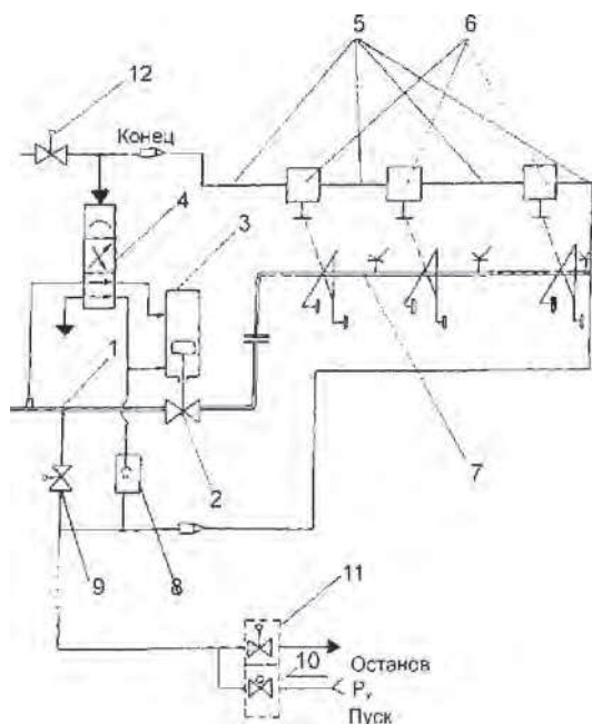
Рис. 3.26. Гидравлическая система аварийной защиты машины: 1 – неподвижный трубопровод; 2 – задвижка; 3 – гидроцилиндр; 4 – гидрореле; 5 – трубка гидрозащиты; 6 – клапаны гидрозащиты; 7 – подвижный трубопровод машины; 8 – обратный клапан; 9, 10, 11, 12 – вентили ручного и дистанционного пуска и останова машины
