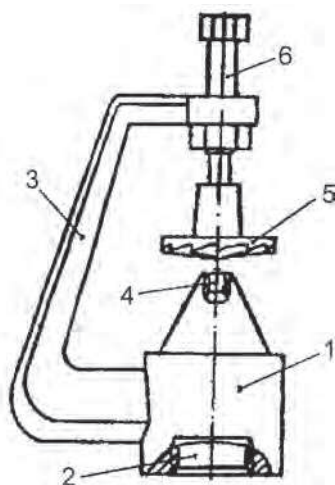
Рис. 4.8. Насадка дугового типа с вращающимся дефлектором: 1 – корпус; 2 – входное отверстие; 3 – дуга-держатель; 4 – выходное сопло; 5 – вращающийся дефлектор; 6 – винт-регулятор
