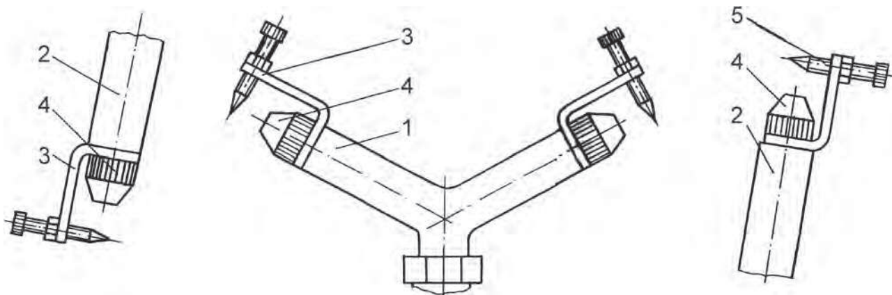
Рис. 7.9. Установка сопел и рассекающих: 1 – корпус дождевательного аппарата; 2 – отключок; 3 – скоба; 4 – сопло; 5 – рассекающий
