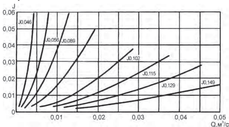
Рис. 8.3. График для определения удельных потерь давления в участковых трубопроводах
