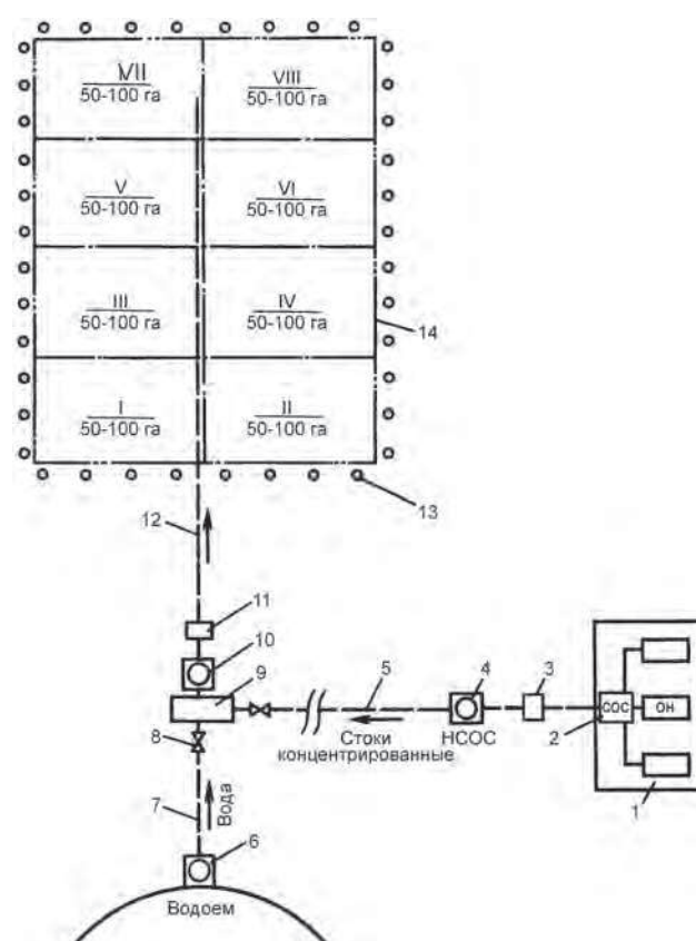
Рис. 10.1. Схема системы внутрипочвенного орошения с использованием животноводческих стоков: 1 – отстойники-навозонакопители (ОН); 2 – сборник осветленных стоков (СОС); 3 – приемный резервуар насосной станции сточных вод; 4 – насосная станция осветленных сточных вод (НСОС); 5 – напорный трубопровод стоков; 6 – насосная станция воды; 7 – напорный трубопровод воды; 8 – задвижка; 9 – смесительная камера; 10 – насосная станция смеси; 11 – узел приготовления минеральных удобрений; 12 – напорный трубопровод смеси; 13 – лесополоса; 14 – поле севооборота с сетью внутрипочвенных увлажнителей; I...VIII – номера полей
