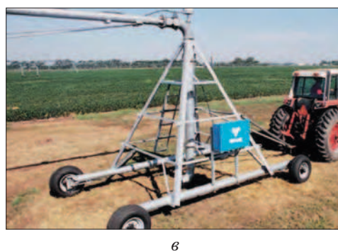
Рис. 3.7. Центральные опоры ЭДМ с поливом в движении по кругу: а – двухколесная буксируемая тележка; б – тележка на полозьях; в – четырехколесная буксируемая тележка
