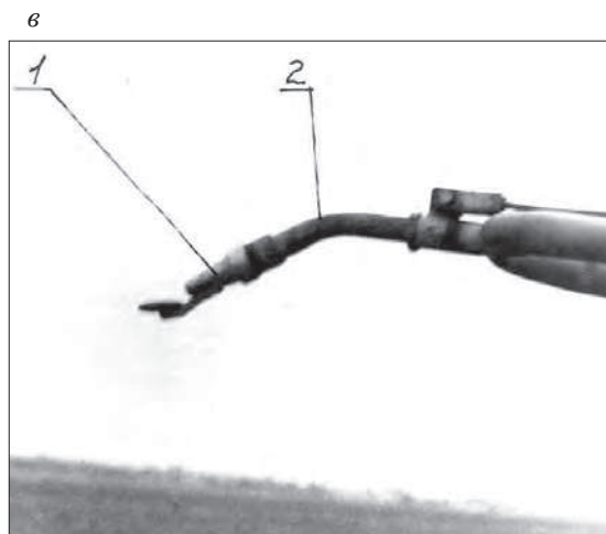
Рис. 3.36. Дефлекторные насадки секторного действия: а – на открылке; б – на трубе; в – концевая
