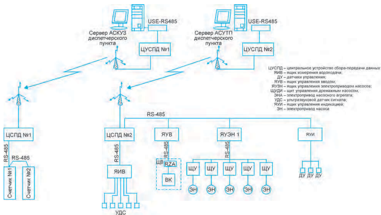
Рис. 12.1. Структурная схема СНС Марьяно-Чеборгульской оросительной системы
