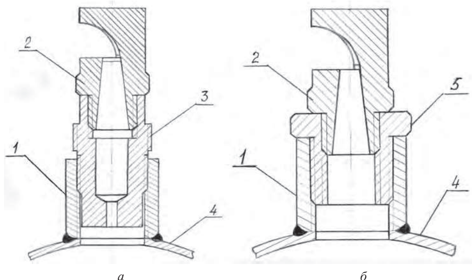
Рис. 3.24. Дождеобразующие устройства «Кубань-ЛК1»: а – с дросселирующим устройством; б – с переходником; 1 – муфта 1"; 2 – насадка короткоструйная секторная; 3 – дросселирующее устройство; 4 – трубопровод дождевальной машины; 5 – переходник
