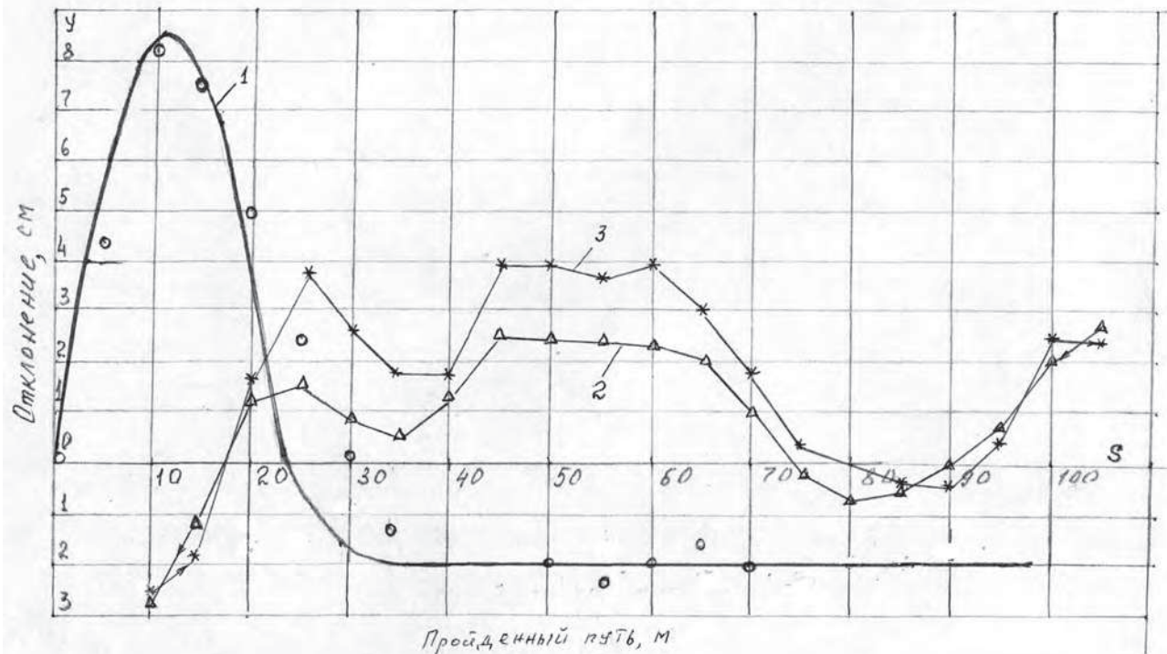
Рис. 3.31. Траектория движения центральной тележки ФДМ «Кубань-Л» по орошаемому участку с системой управления: 1 – теоретическая траектория движения центральной тележки машины при начальной ее установке под углом \varphi=0,92^\circ и о – фактическое значение; 2, 3 – экспериментальные отклонения центральной тележки машины при неоднократном движении машины и образовавшей колеи соответственно от начала к концу поля (кривая 2, \Delta – фактическое значение) и обратном направлении (кривая 3, * – фактическое значение) от возмущающих воздействий y_e
