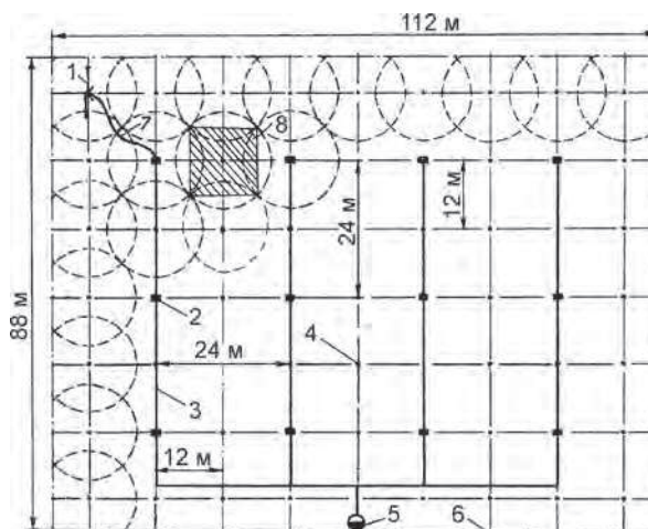
Рис 7.4. Технологическая схема орошения участка площадью до 1 га: 1 – дождевальная шланговая установка ДШУ-09; 2 – гидрант; 3 – оросительный трубопровод; 4 – позиции для работы ДШУ-09; 5 – насос; 6 – граница участка; 7 – питающий шланг; 8 – площадь орошения с перекрытием
