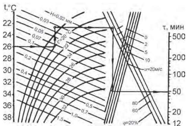
Рис. 6.14. Номограмма для расчета режима мелкодисперсного увлажнения (по А.П. Лихацевичу)
