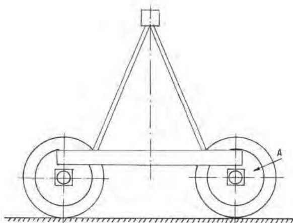
Рис. 3.27. Схема самоходной тележки машины с гипоидным приводом
