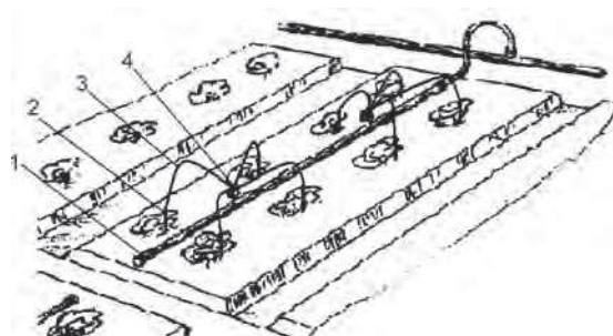
Рис. 8.18. Водовыпуски поливного трубопровода в теплице:
