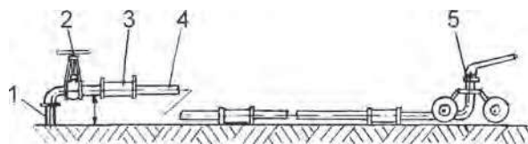
Рис. 5.16. Общий вид комплекта: 1 – гидрант оросительной сети; 2 – узел подсоединения трубопровода Ø110 мм, к гидранту; 3 – муфта Ø110 мм; 4 – полиэтиленовая труба Ø110 мм, l = 6 м; 5 – тележка с дождевальным аппаратом
