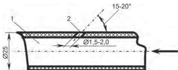
Рис. 8.17. Струйный водовыпуск
