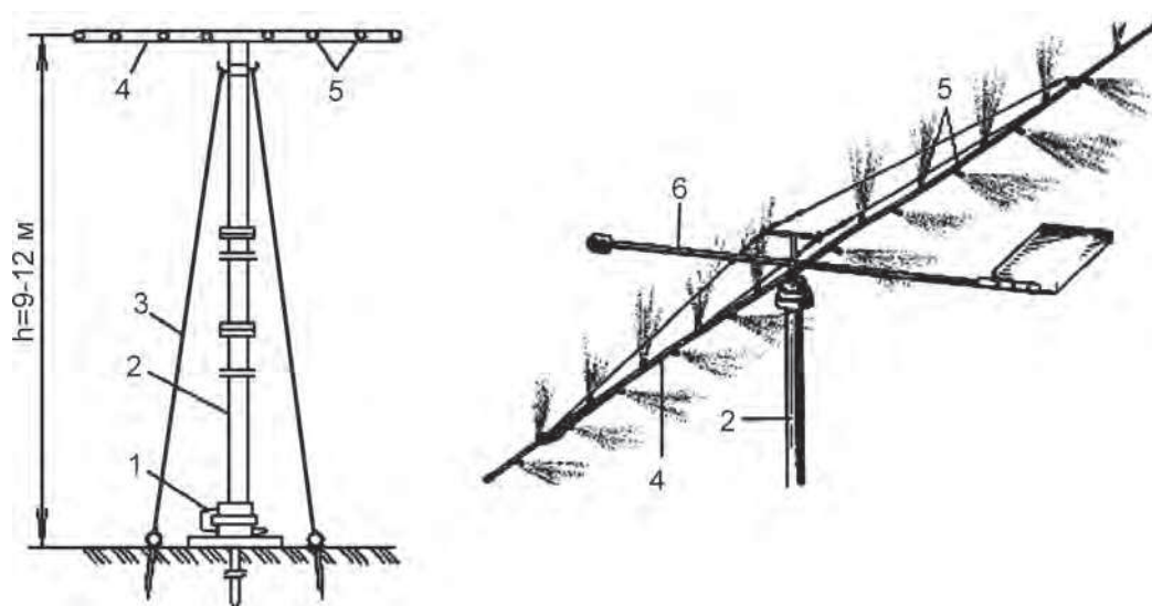
Рис. 6.17. Схема мелкодисперсной стационарной установки ВНПО «Радуга»: 1 – основание стойки; 2 – стойка; 3 – растяжки; 4 – штанга поворотная; 5 – форсунки; 6 – флюгер
