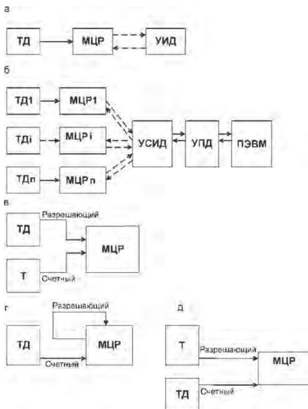
Рис. 1.14. Структурные схемы соединения средств регистрации:
