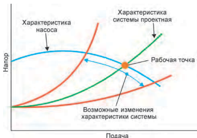
Рис.12.3. Рабочая характеристика оросительной системы и насосно-силового агрегата
