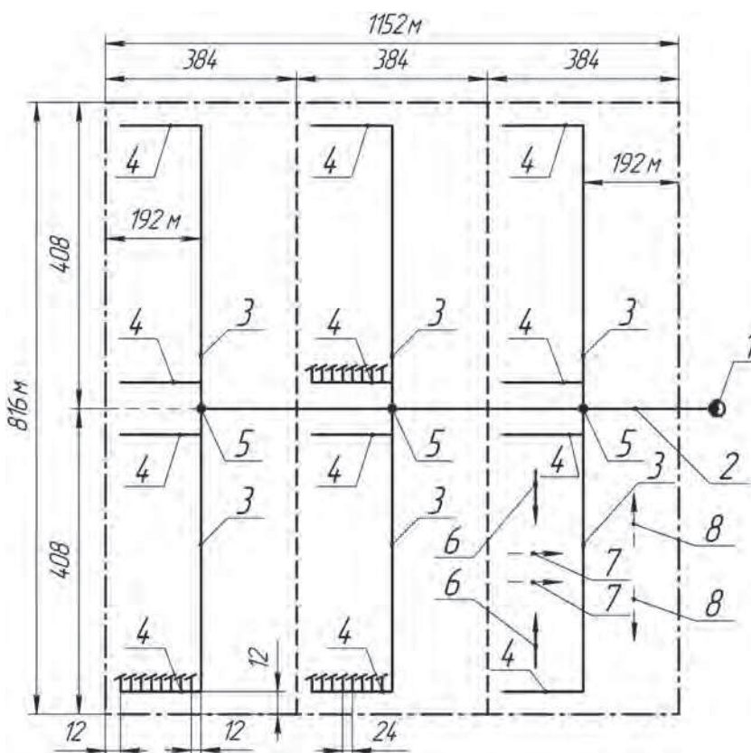
Рис. 5.21. Схема орошения участка десяти комплектами КИ-15 ( S=94 га, расход 88-90 л/с): 1 – насосная станция; 2 – магистральный трубопровод закрытой оросительной сети; 3 – распределительный трубопровод \Phi 110 мм, l = 396 м комплекта КИ-15; 4 – дождевальное крыло \Phi 90 мм, l = 180 м; 5 – гидрант с узлом подсоединения распределительных трубопроводов двух комплектов КИ-15; 6, 7, 8 – направления перемещения дождевальных крыльев
