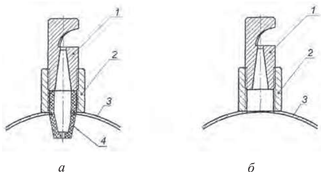
Рис. 3.20. Дождеобразующие устройства для ДМ «Фрегат»: а – с дросселирующим элементом (дюзой); б – без дросселирующего элемента; 1 – короткоструйная секторная насадка; 2 – муфта 1/2"; 3 – трубопровод ДМ «Фрегат» 4 – дросселирующий элемент
