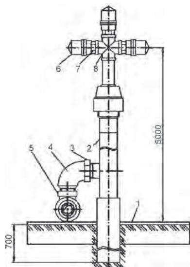
Рис. 6.19. Дождеватель: 1 – основание (анкер); 2 – трубчатый стояк; 3 – контргайка; 4 – угольник; 5 – тройник; 6 – насадка; 7 – ниппель; 8 – крестовина
