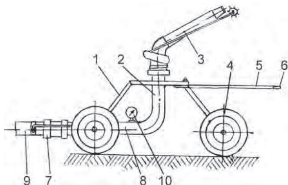
Рис. 5.18. Передвижная тележка: 1 – рама; 2 – стояк; 3 – дождевальный аппарат; 4 – колесо; 5 – водило; 6 – ручка; 7 – подводящая труба тележки; 8 – муфта; 9 – трубопровод; 10 – манометр
