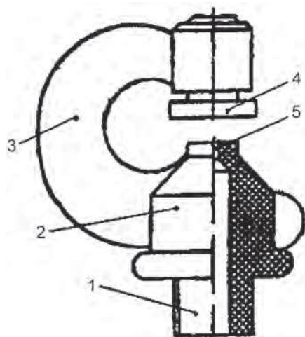
Рис. 4.7. Насадка дугового типа с плоским дефлектором: 1 – входное отверстие; 2 – корпус; 3 – дуга-держатель; 4 – плоский дефлектор; 5 – выходное сопло
