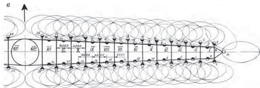
Рис. 3.35. Схемы расстановки дождеобразующих устройств на дождевальных агрегатах ДДА-100МА и карты формирования дождя: а – серийный; б – модернизированный для почв средней и пониженной водопроницаемости; в – модернизированный для почв низкой водопроницаемости
