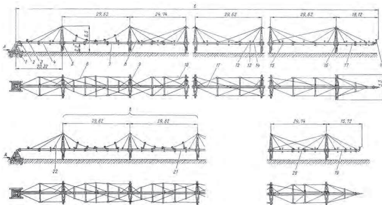
Рис. 3.19. Размещение основных частей машины ДМ «Фрегат»:
