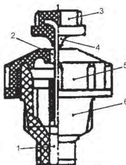
Рис. 4.6. Насадка стержневого типа: 1 – входное отверстие; 2 – выходное отверстие (сопло); 3 – гайка-регулятор; 4 – дефлектор; 5 – крышка; 6 – корпус
