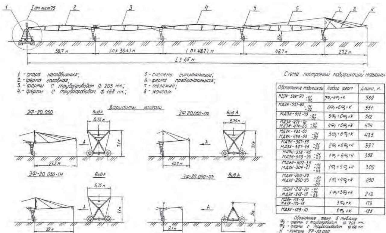
Рис. 3.23. Схема общего вида и составление модификаций дождевальной машины «Кубань-ЛК1»
