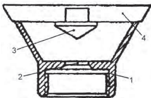
Рис. 4.9. Насадка кругового действия с коническим неподвижным дефлектором: 1 – корпус; 2 – выходное отверстие (сопло); 3 – конический дефлектор; 4 – планка-держатель
