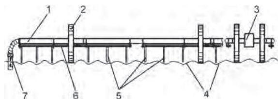
Рис. 9.15. Принципиальная схема поливного колесного трубопровода ТКП-П:
