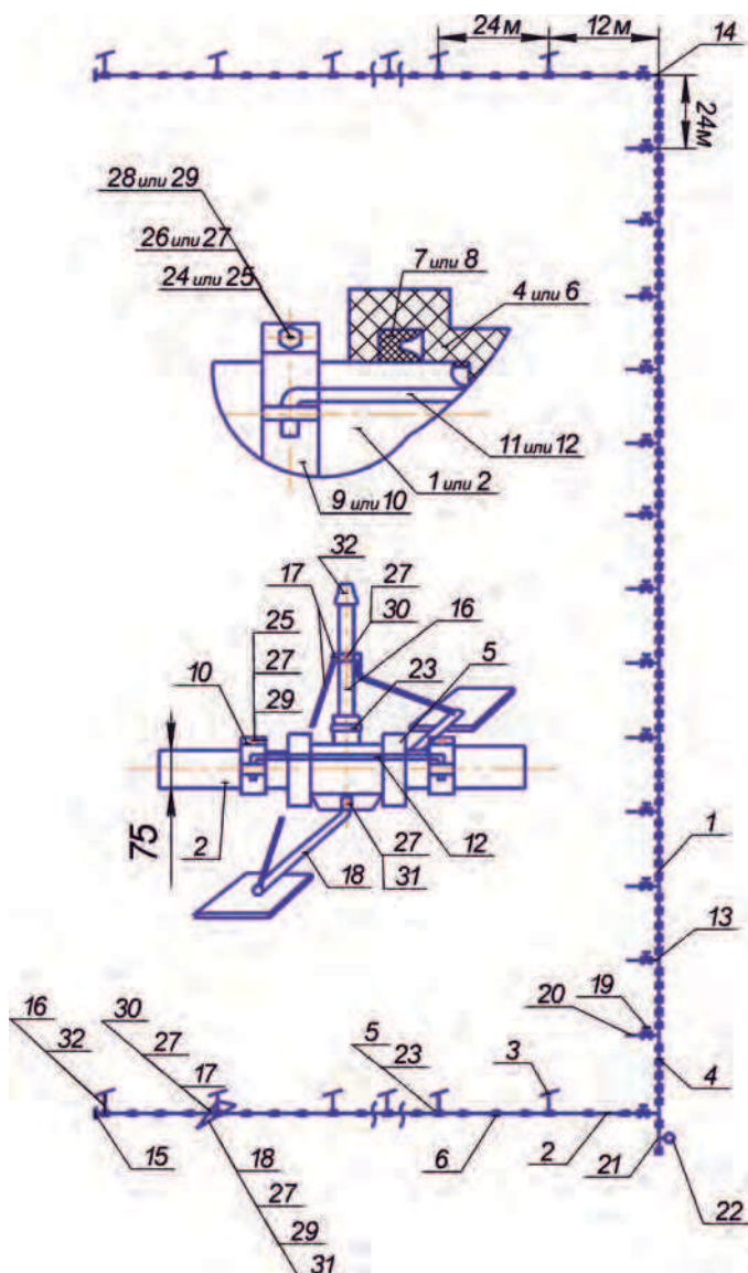
Рис. 5.4. Монтажная схема комплекта КИ-10
