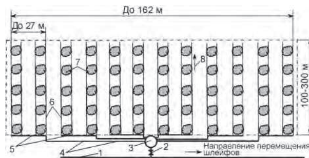
Рис. 9.7. Технологическая схема импульсного полива сада по бороздам комплектом КИП-С:
