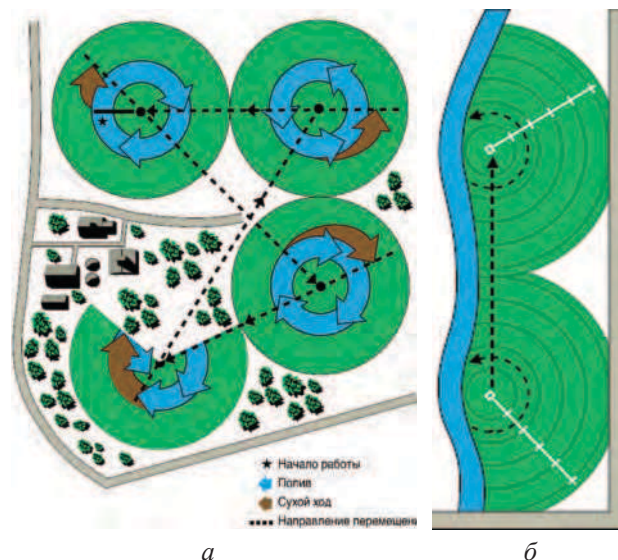
Рис. 3.9. Схема буксировки ЭДМ: а – с поливом в движении по кругу с двухколесной тележкой; б – при секторном поливе
