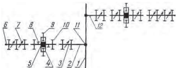
Рис. 3.32. Общая схема устройства колесных дождевальных трубопроводов: 1 – оросительный трубопровод; 2 – узел присоединения; 3 – секция трубопровода; 4 – приводная тележка; 5 – двигатель привода с реверс-редуктором; 6 – концевая заглушка; 7 – дождевальный аппарат с механизмом самоустановки; 8 – тормозной упор; 9 – ведущее колесо; 10 – опорное колесо; 11 – гидрант с колонкой; 12 – второе крыло
