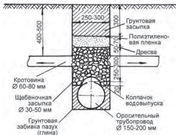
Рис. 10.7. Поперечный разрез траншеи оросительного трубопровода с пористой засыпкой
