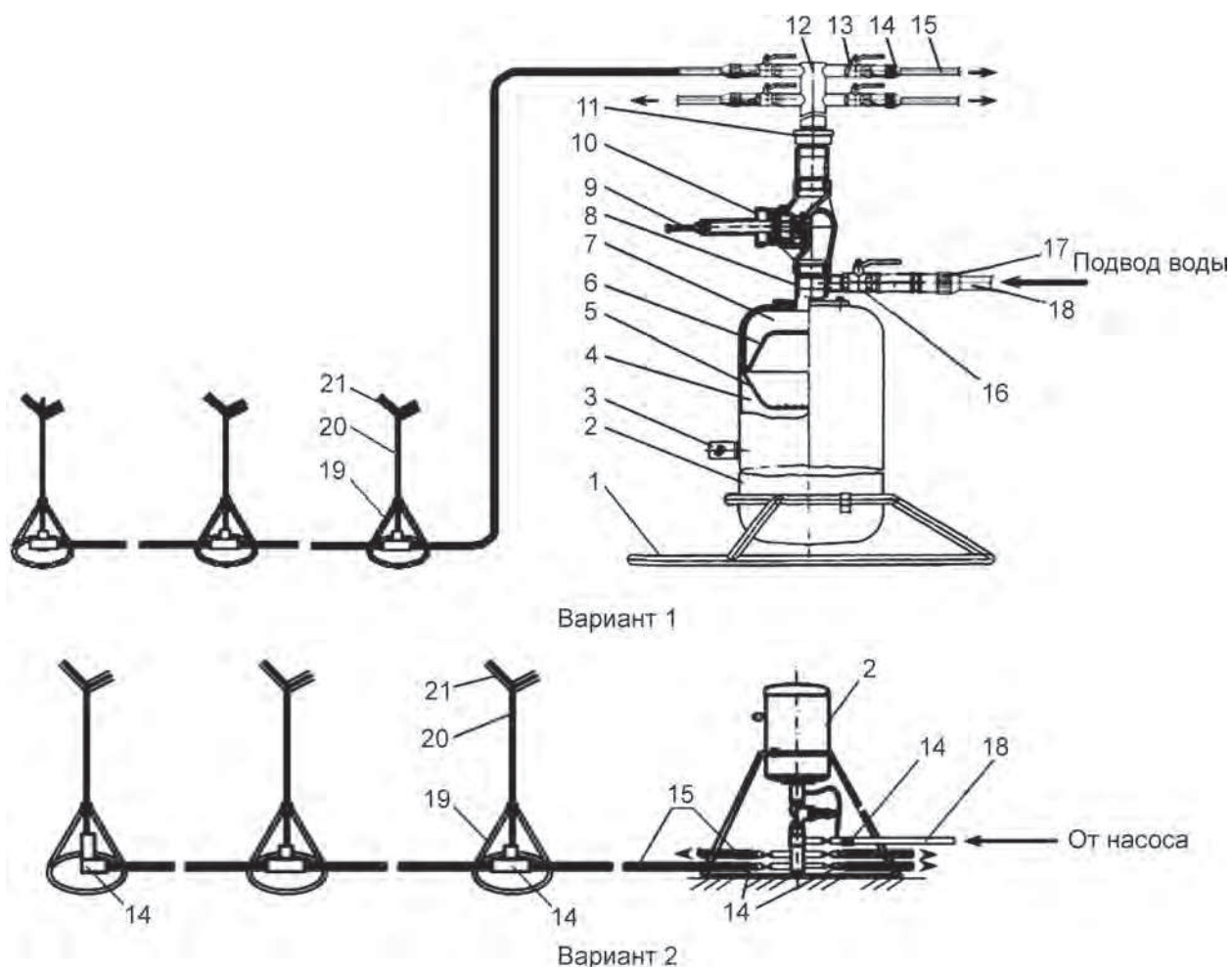
Рис. 6.11. Схема импульсного аппарата и поливного трубопровода КСИД-Р:
