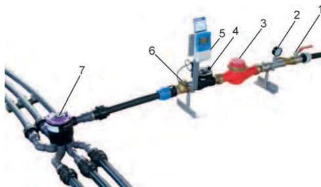
Рис. 6.13. Узел управления комплекта КИД-1: 1 – кран; 2 – манометр; 3 – счётчик воды; 4 – клапан электроуправляемый; 5 – контроллер-таймер; 6 – обратный клапан; 7 – клапан распределительный
