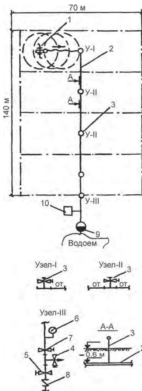
Рис. 7.11. Технологическая схема полива модульного участка с ДШ-1: 1 – дождеватель шланговый ДШ-1; 2 – оросительный трубопровод; 3 – гидрант в сборе; 4 – вентиль; 5 – задвижка, 6 – счетчик воды; 7 – регулятор давления; 8 – клапан обратный; 9 – электрифицированная насосная станция; 10 – гидроподкормщик
