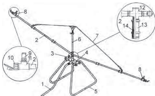
Рис. 7.2. Схема дождевальной шланговой установки ДШУ-09: 1 – подводящий шланг; 2 – водопроводящее звено; 3 – узел вращения; 4 – платформа; 5 – опора; 6 – стояк; 7 – регулируемые растяжки с крюками; 8 – пакет дождевальных насадок; 9 – вертикальные дождевальные насадки секторного действия; 10 – концевая насадка горизонтального действия; 11 – тройник; 12 – крестовина; 13 – корпус; 14 – стакан
