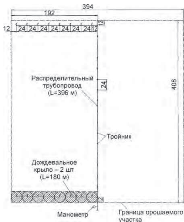
Рис. 5.9. Схема участка и монтажа комплекта КИ-15
