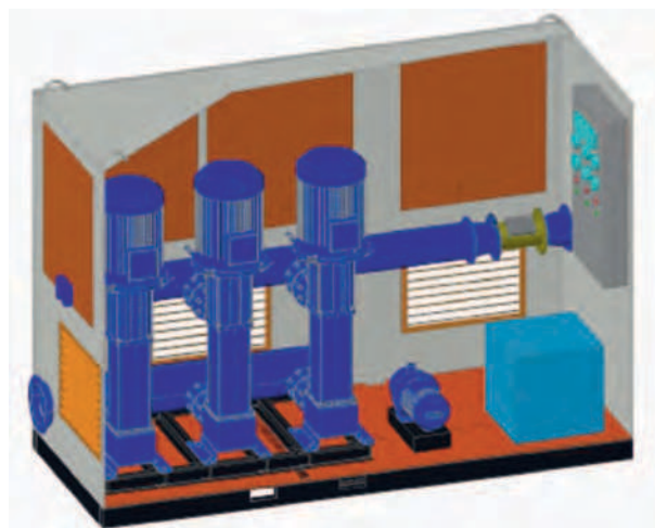
Рис.12.7. Общий вид насосной установки типа «Ладога» на базе насосов ЦНС
