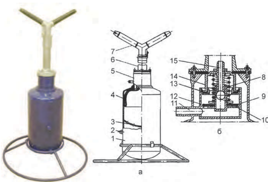
Рис. 6.2. Импульсный дождевательный аппарат ДИ-15 (а) и его гидроуправляемый запорный орган (б): 1 – пневмогидроаккумулятор; 2 – штуцер для закачивания воздуха; 3 – перфорированный ограничительный свод; 4 – эластичная шаровая мембрана; 5 – гидроуправляемый запорный орган; 6 – стояк; 7 – дождевательная насадка; 8 – пружина; 9 – обратный клапан; 10 – шаровой клапан; 11 – штуцер; 12 – центральная камера; 13 – манжета; 14 – поршень; 15 – сбросная втулка
