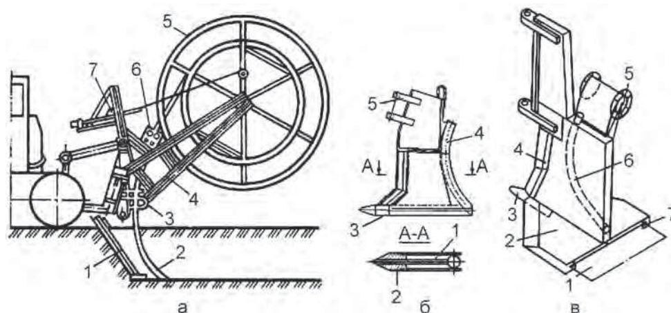
Рис. 10.4. Навесной бестраншейный трубоукладчик:
