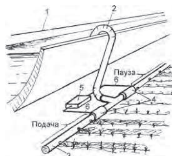
Рис. 9.4. Переносной клапанный комплект дискретного полива (КДП)
