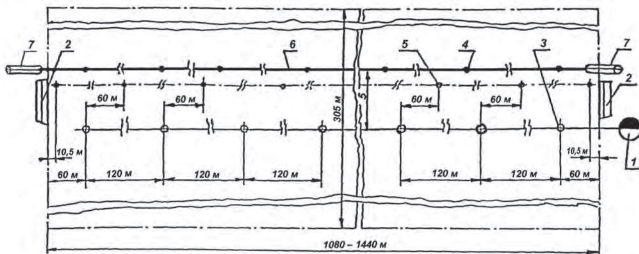
Рис. 3.12. Схема оросительной сети и оборудования для управления дождевальной машиной «Ладога»: 1 – насосная станция; 2 – упор «конца поля»; 3 – гидрант оросительной сети; 4 – стойка поддержки троса; 5 – упор для автоматической остановки; 6 – направляющий трос; 7 – тумба
