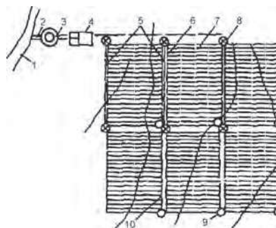
Рис. 10.2. Схема системы внутрипочвенного орошения:
