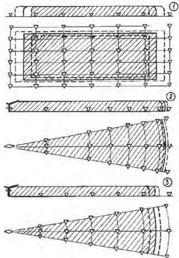
Рис. 1.4. Схемы расстановки: 1 — прямоугольная; 2 — радиальная с равными по площади кольцевыми зонами; 3 — радиальная с равным шагом; Δ — дождемеры
