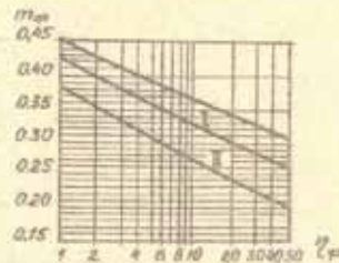
Рис. 3. График m_\phi = f(Z_\phi) допустимой пористости грунтов укладываемых в фильтры
