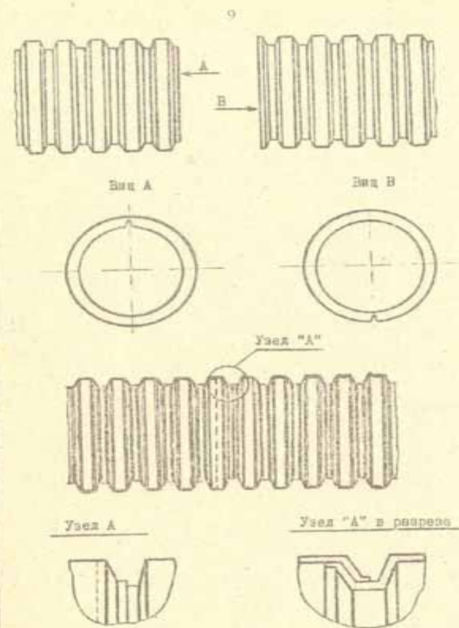
Рис. 3 Соединение плосотносочных гофрированных труб, одинаковых по диаметру
