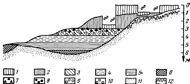
Рис. 2.9. Важнейшие профили болот в северной части ФРГ [3.2]: 1 — молодой мховый торф; 2 — старый мховый торф; 3 — торф разнороссы; 4 — осоковый торф; 5 — тростниковый торф; 6 — сапропель; 7 — сосновые луга в торфе; 8 — сосновая древесина; 9 — березовая древесина; 10 — ольховая древесина; 11 — песок; 12 — ортсанд.
