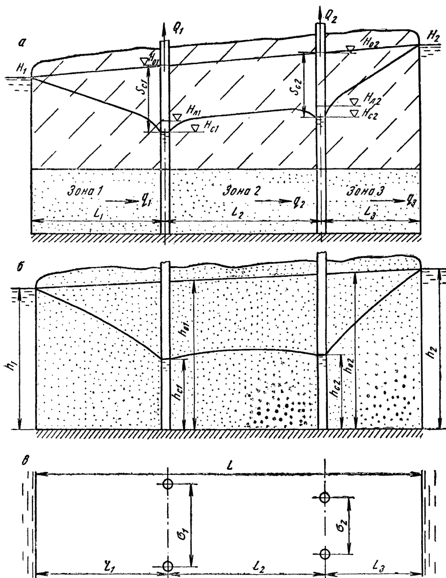
Рис. 53. Два ряда скважин между двумя областями питания или стока: а, б — разрезы для напорного и однородного безнапорного потоков, в — план расположения скважин
