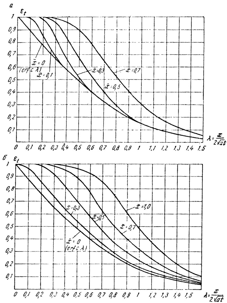
Рис. 12. Графики относительного подпора грунтовых вод \varepsilon_t : а — в потоке с постоянным напором на верховой границе, б — в потоке с непро- ницаемой верховой границей [14] при \lambda = x/L
