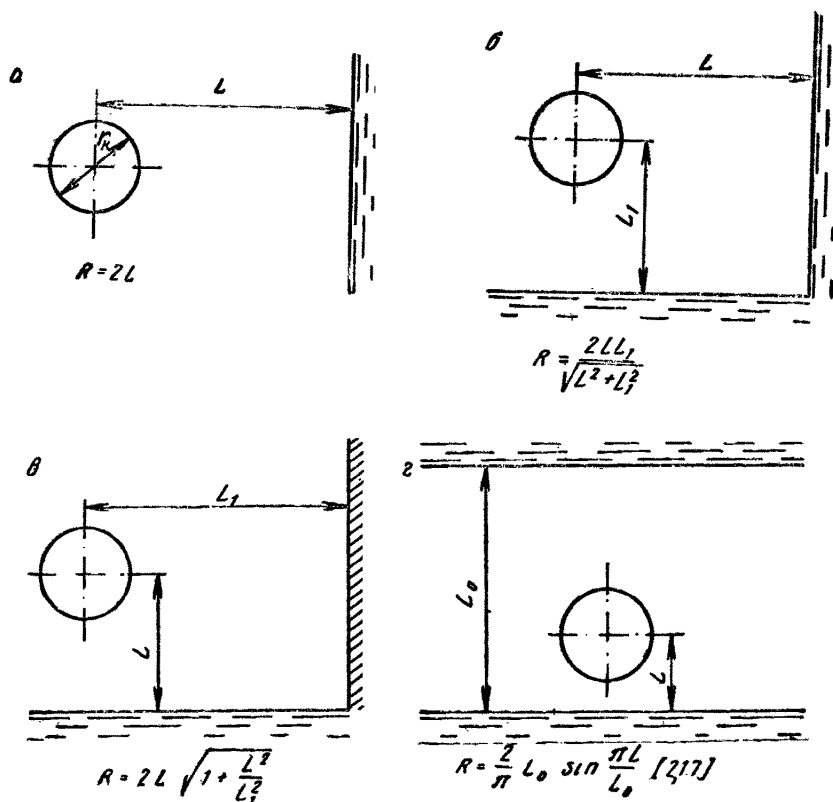
Рис. 50. Схемы условий а — колодец у реки у линейной области питания, б — колодец в углу, между двумя границей, в — колодец в полосе между двумя областями питания или стока, г — колодец в круговой области питания, ж — колодец в неоднородном полуграничи
