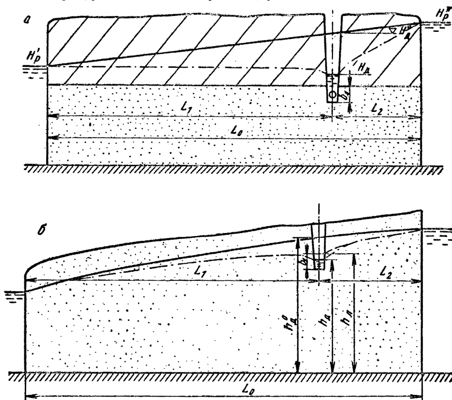
Рис. 54. Горизонтальная дрена между двумя контурами питания или стока: а — в пласте с постоянной проводимостью, б — в однородном безнапорном пласте
