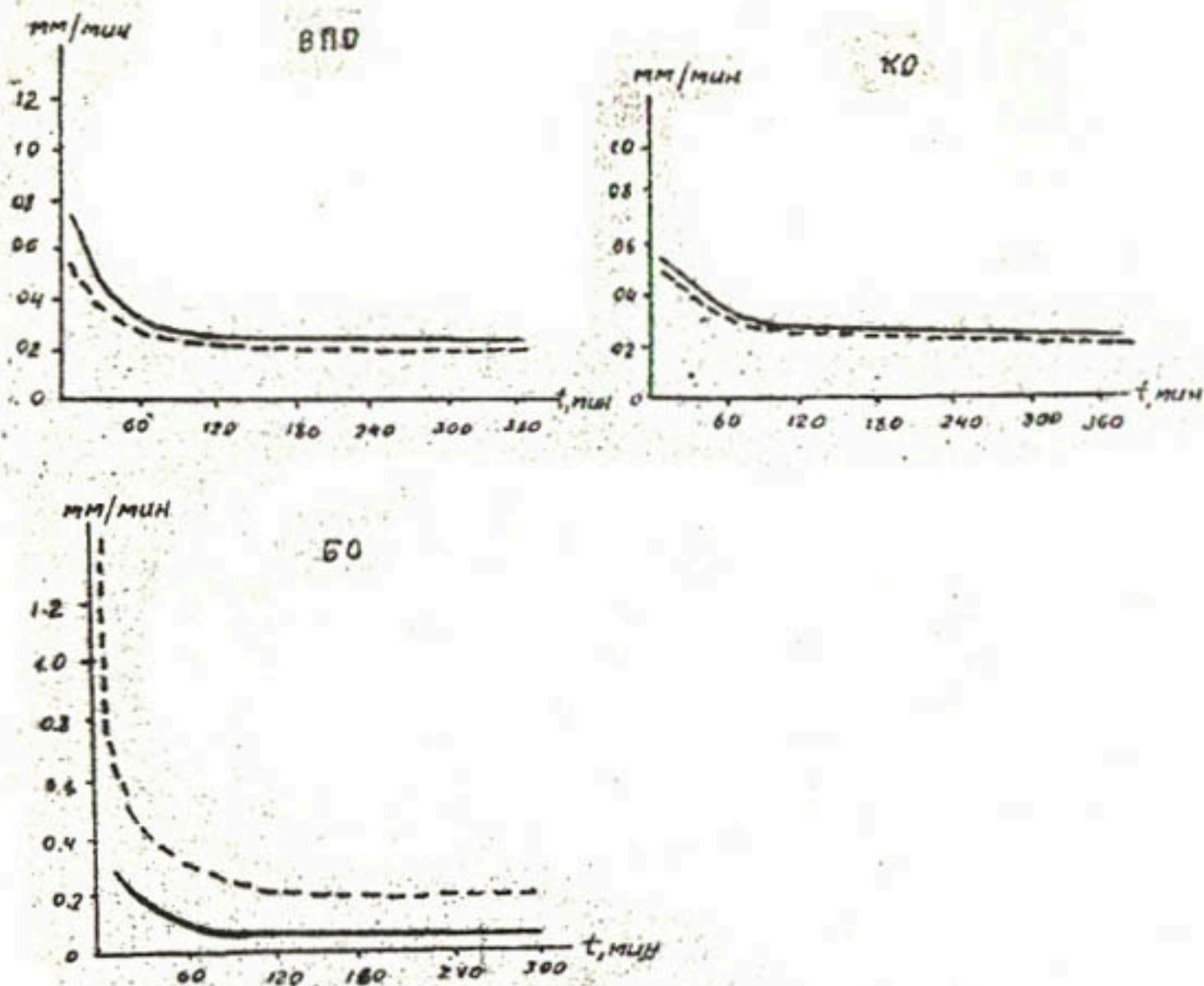
Рис. 3. Водопроницаемость почв: ---- после сева; — в конце вегетации
