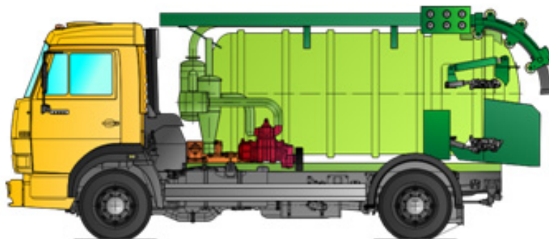
Рис. 1. Машина ДКТ-305 для эксплуатации до -10^{\circ}\text{C} с самосвальным механизмом разгрузки и кассетой всасывающего рукава
