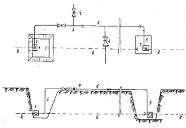
Рис. 3. Схема монтажа разборного трубопровода на восстанавливаемом участке водопровода.
