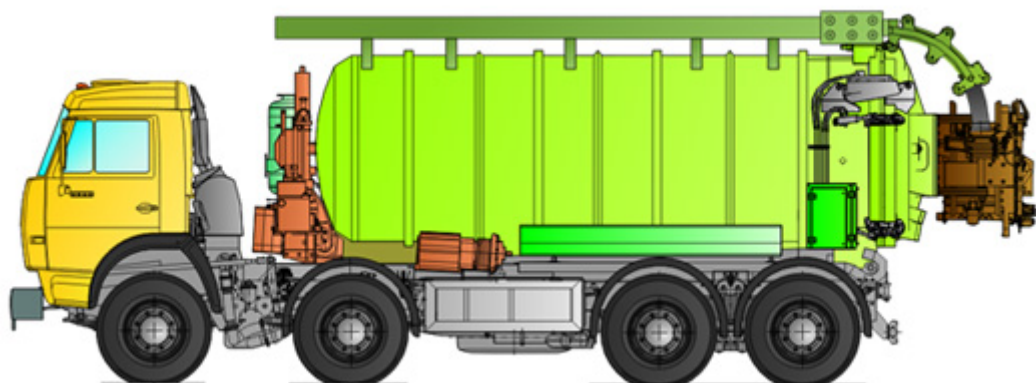
Рис. 1. Машина ДКТ-320 с обогревателем воды для эксплуатации до -10°C
