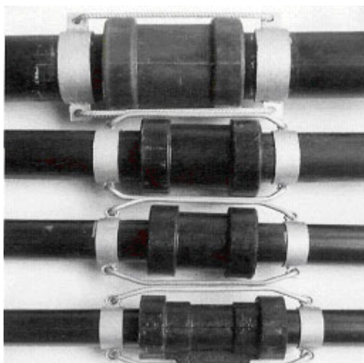
Рис.1. Сборно-разборные трубопроводы Д 75, 90, 110, 160 мм
