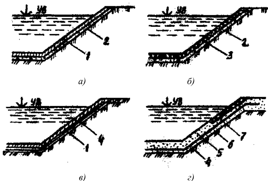
a – бетонные и железобетонные; б – асфальтобетонные; в – бетонопленочные; г – грунтопленочные; 1 – бетонное покрытие; 2 – подстилающий слой щебня; 3 – слой асфальтобетона; 4 – пленочный противофильтрационный экран; 5, 6 – грунт; 7 – крепление камнем
